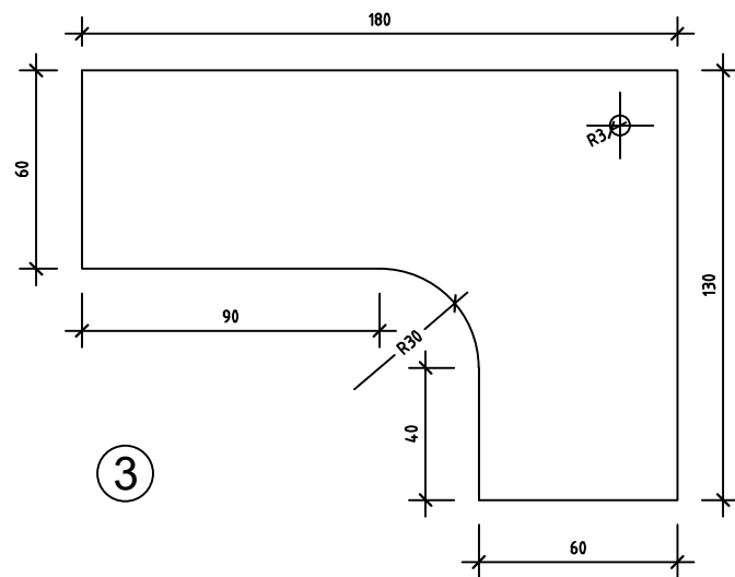
VISTA SUPERIOR (mesa meio ambiente)
