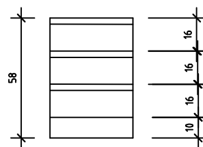
VISTA FRONTAL GAVETEIRO
