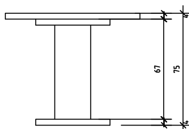
VISTA FRONTAL (mesa redonda)
