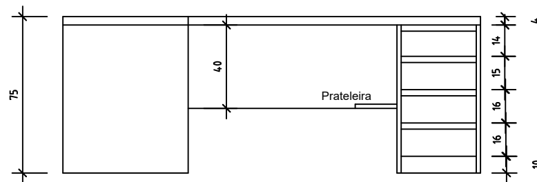
VISTA FRONTAL MESA (meio ambiente)
