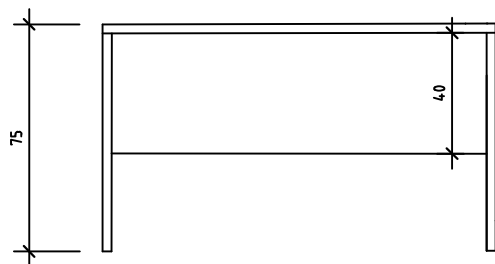
VISTA FRONTAL MESA (meio ambiente)
