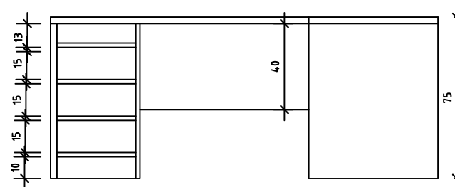
VISTA FRONTAL(mesa meio ambiente)
