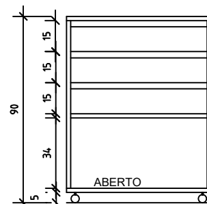
VISTA FRONTAL (APOIO)
