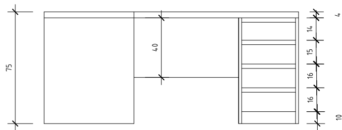
VISTA FRONTAL MESA (Assistência)
