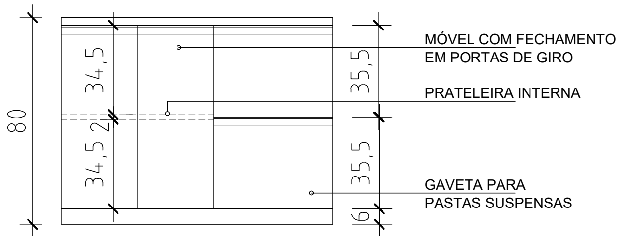
02 Vista Frontes Fechadas Esc. 1/100
