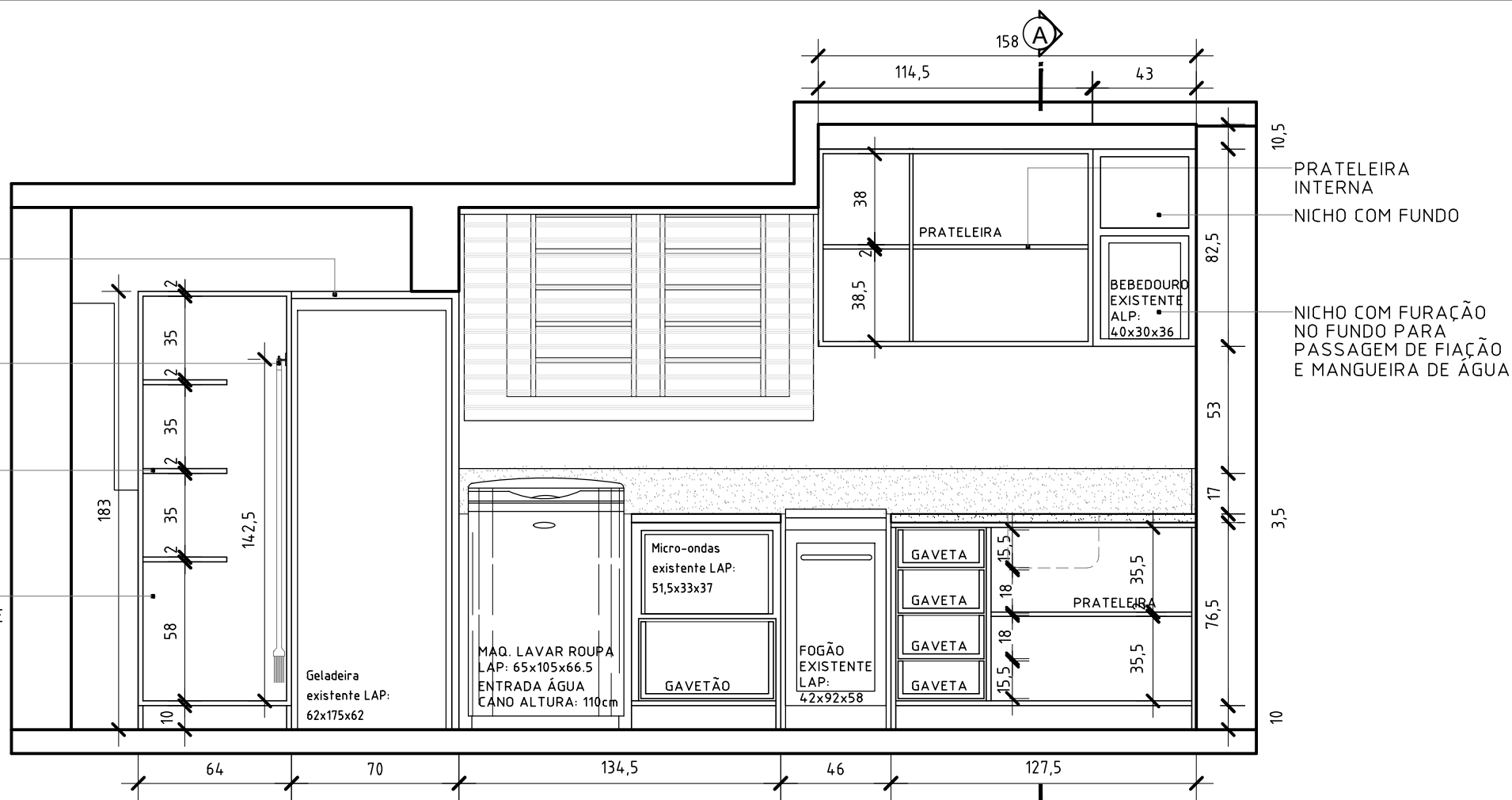
MÓVEIS EM MDF 18mm COR BRANCO. NICHOS EM MDF 36mm COR BRANCO. GRANITO A DEFINIR TODAS AS DOBRADIÇAS E CORREDIÇAS SERÃO COM SISTEMA DE AMORTECIMENTO OS PUXADORES SERÃO DO TIPO BARRA NA COR ALUMÍNIO COM PROTEÇÃO NAS EXTREMIDADES.
