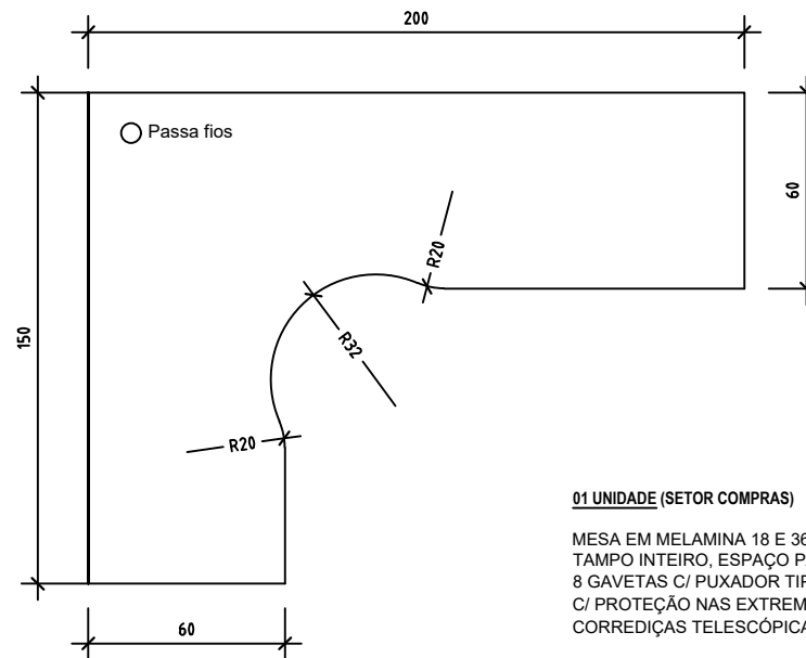
VISTA SUPERIOR (mesa compras)
