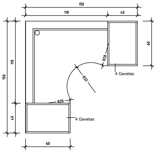
VISTA INFERIOR (mesa compras)
