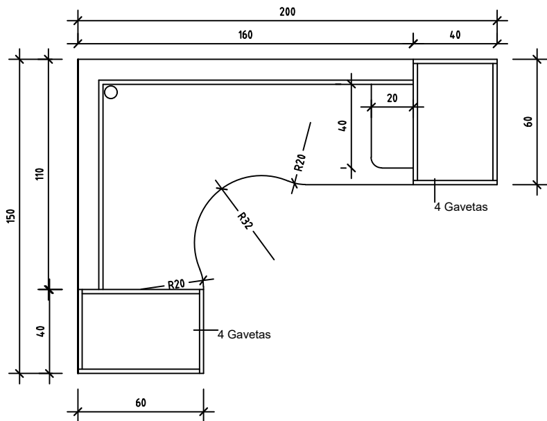
VISTA INFERIOR (mesa compras)
