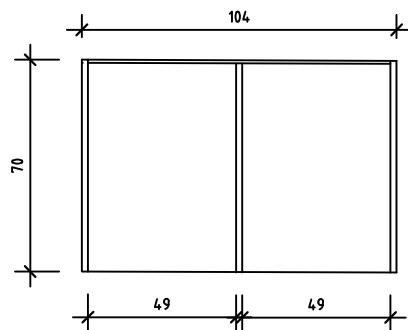
VISTA INFERIOR (armário FAPS)
