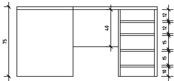
VISTA LATERAL (mesa compras)
