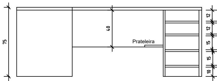
VISTA LATERAL (mesa compras)
