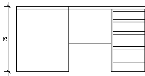
VISTA FRONTAL (mesa compras)
