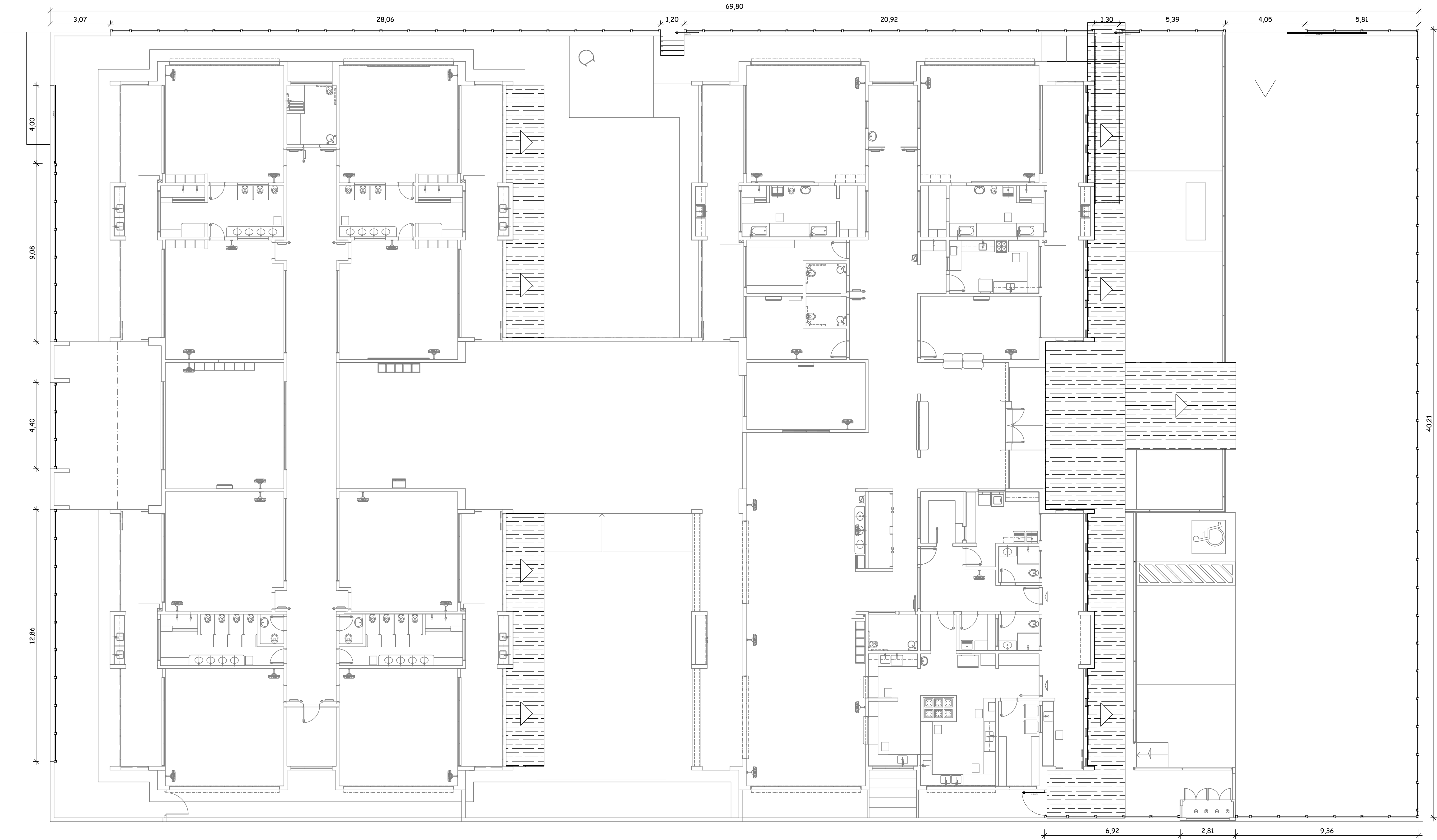
IMPLANTAÇÃO ESC.: 1/120
