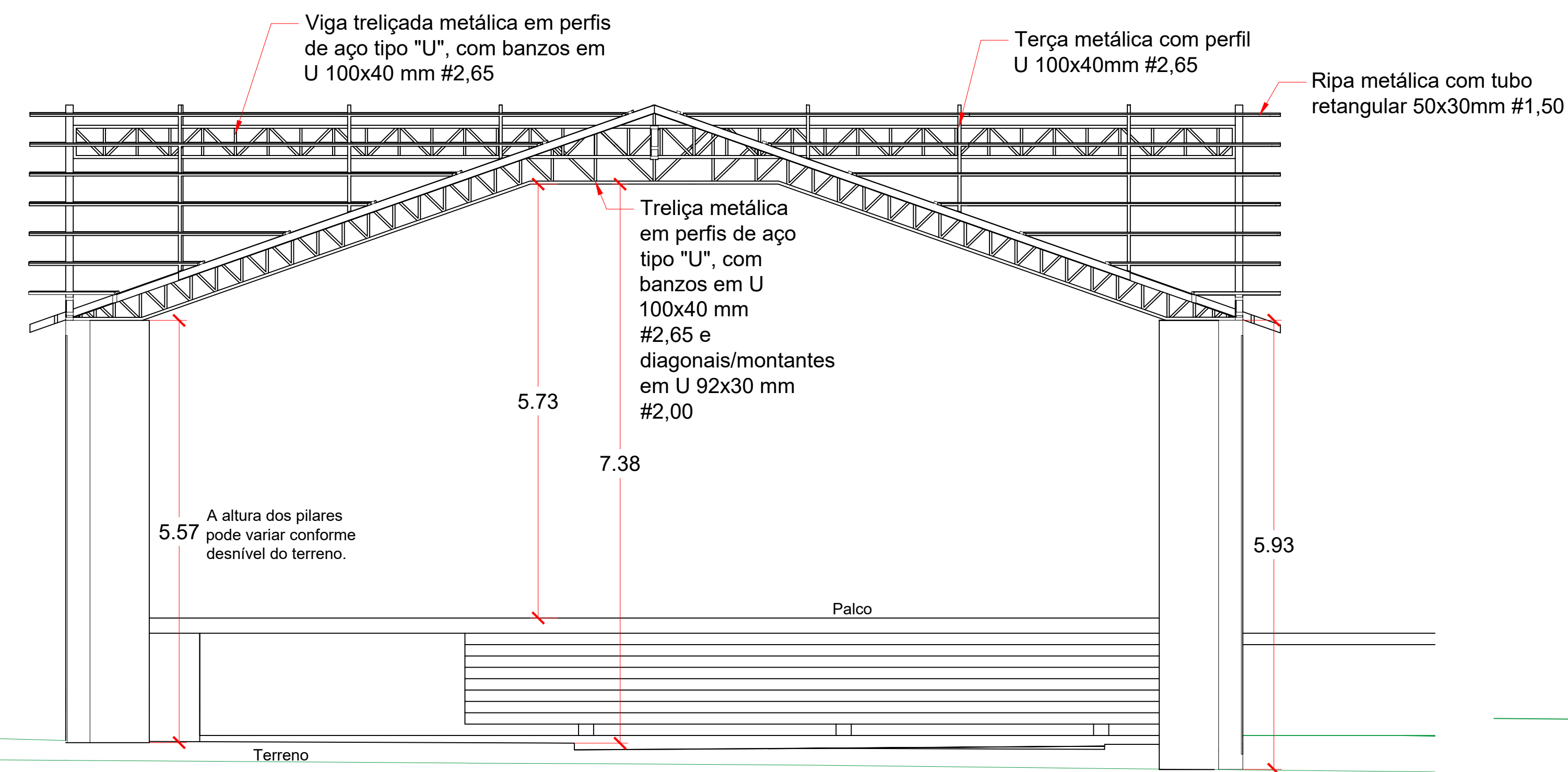
VISTA FRONTAL ESC.: 1:50
