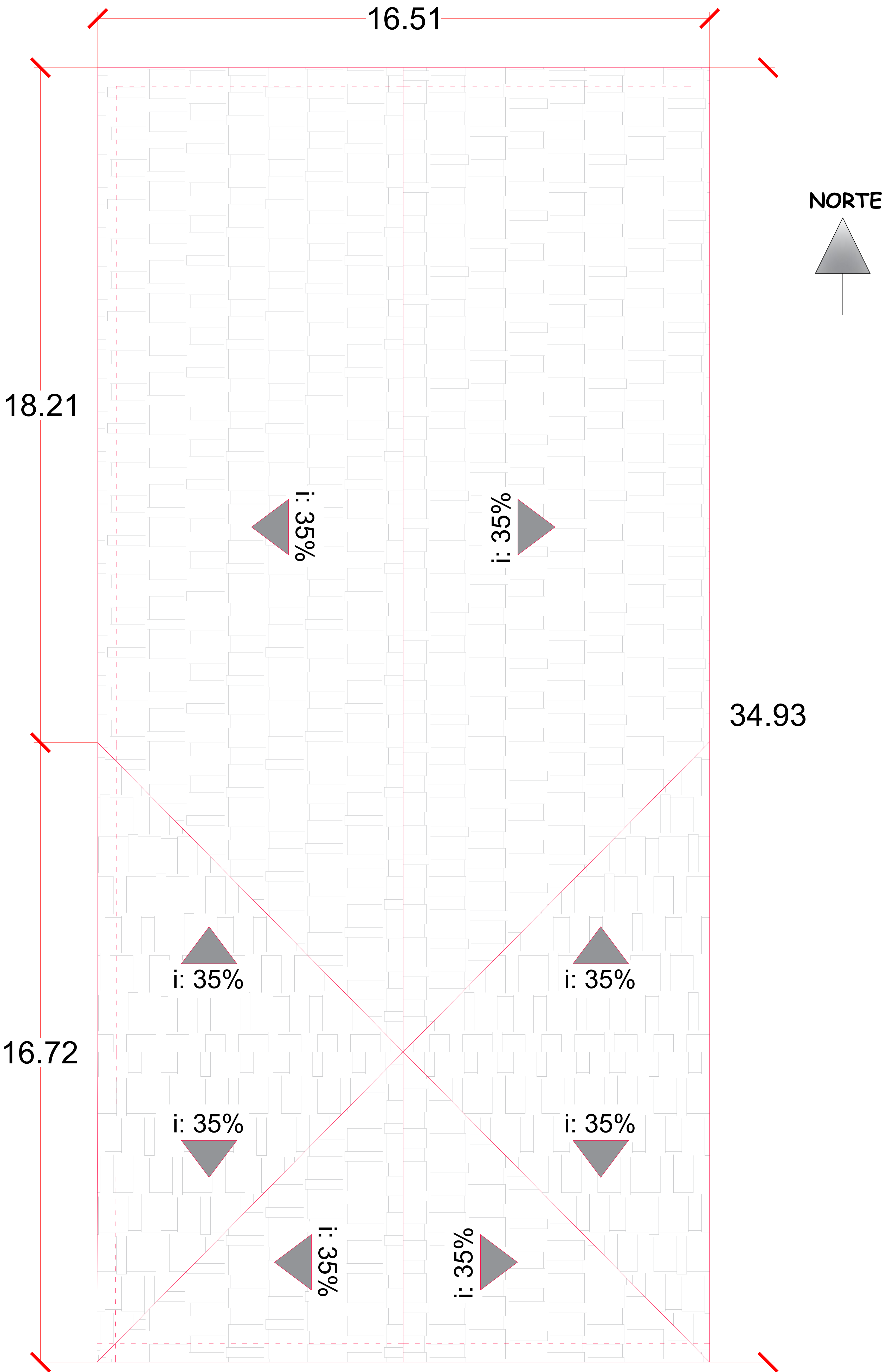
PLANTA DE COBERTURA ESC.: 1:50
