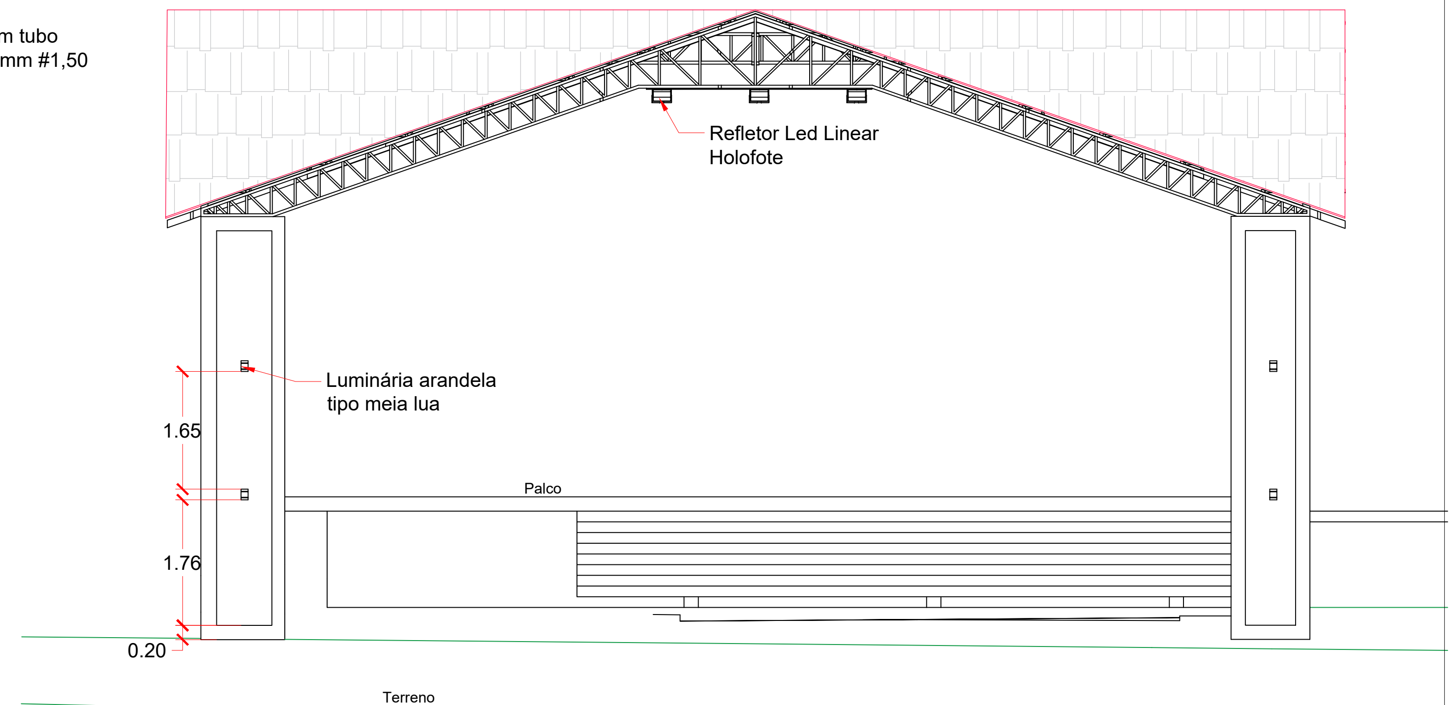
FACHADA ESC.: 1:50
