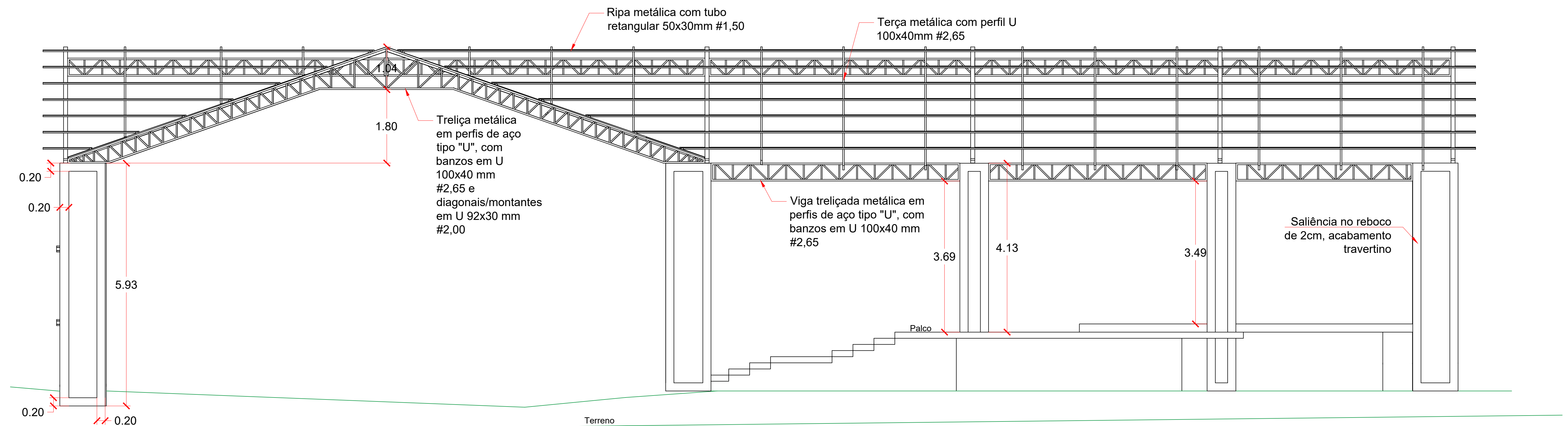
VISTA LATERAL ESC.: 1:50
