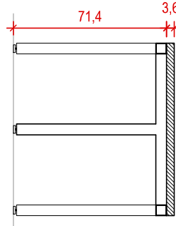
CORTE AA
