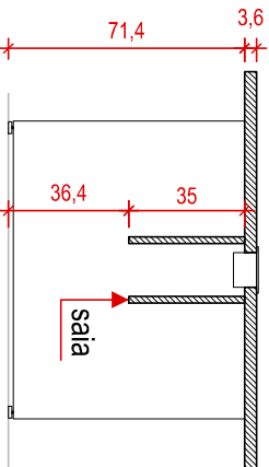
CORTE AA
