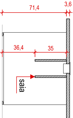
CORTE AA
