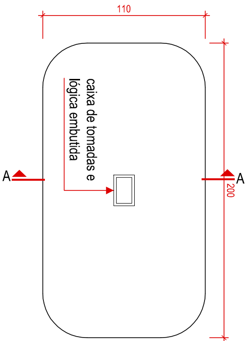
VISTA SUPERIOR
