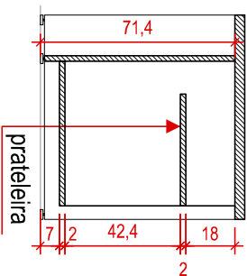
CORTE BB
