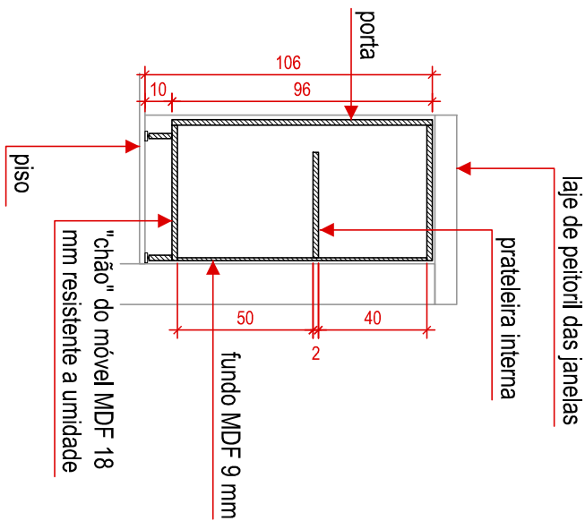
CORTE TRANSVERSAL
