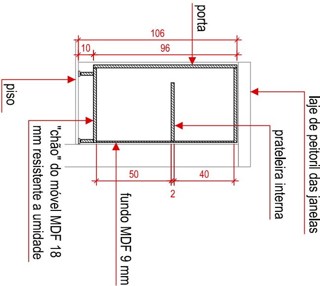
CORTE TRANSVERSAL (todos os balcões sob as janelas)
