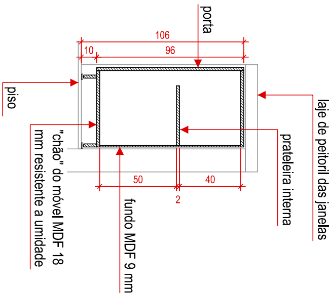
CORTE TRANSVERSAL
