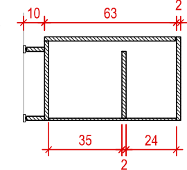
CORTE AA
