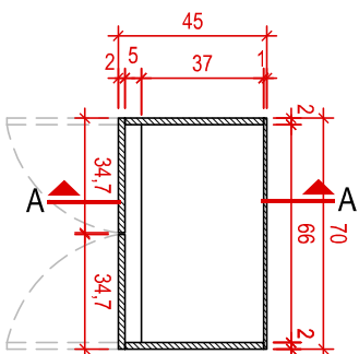
PLANTA BAIXA
