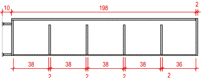
CORTE AA
