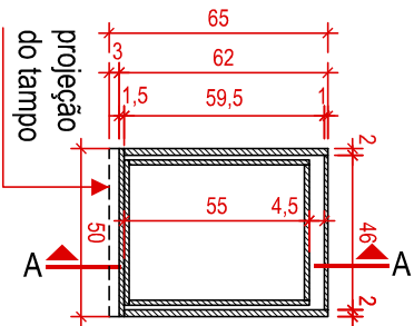
PLANTA BAIXA
