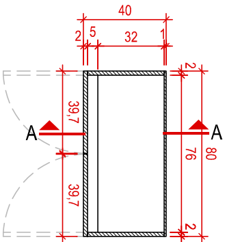
PLANTA BAIXA
