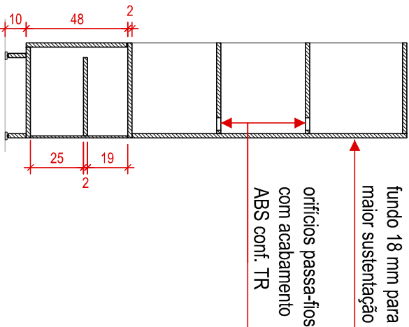
CORTE AA
