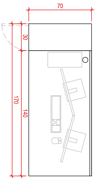
VISTA SUPERIOR
