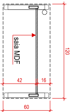
PLANTA BAIXA
