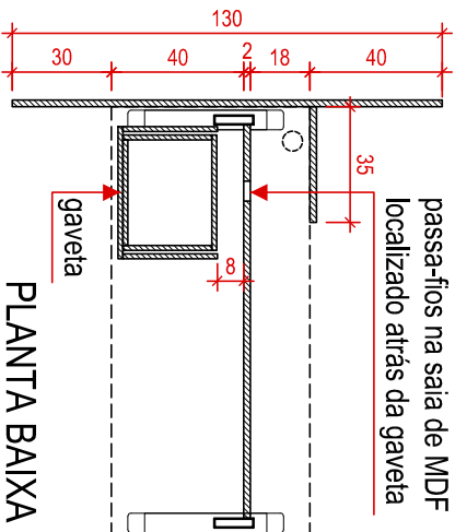
PLANTA BAIXA SUPORTE CPU
