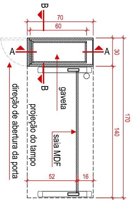
PLANTA BAIXA
