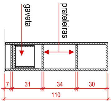
CORTE BB
