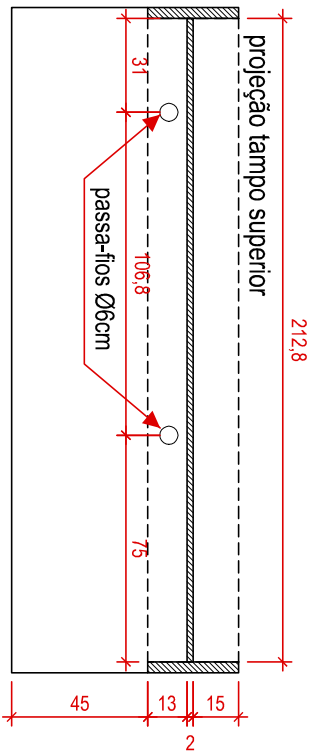
PLANTA BAIXA - TAMPO
