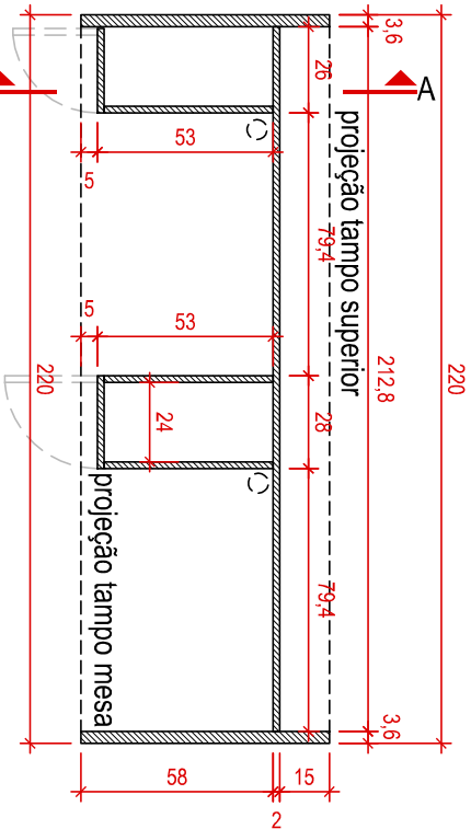
PLANTA BAIXA - PÉS
