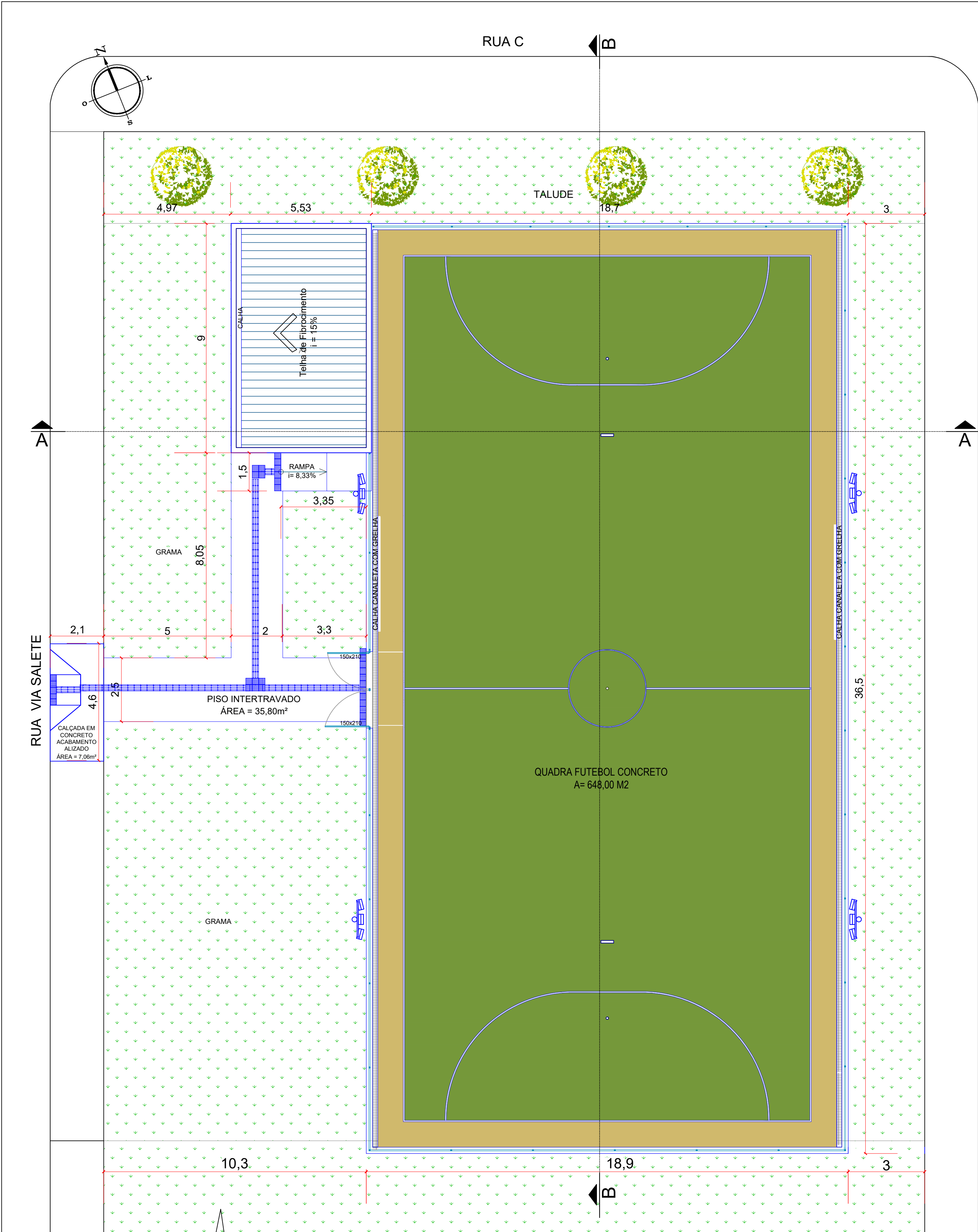
PLANTA BAIXA E PLANTA DE LOCALIZAÇÃO ESC: 1/100
