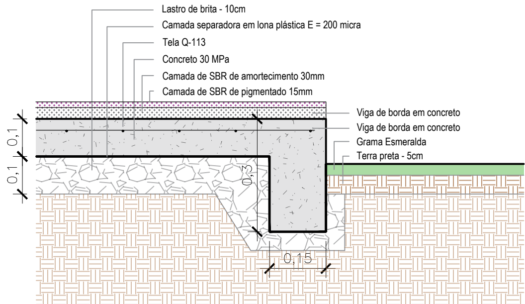
DETALHE RADIER
