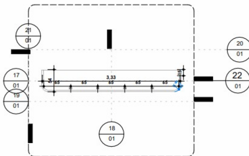
Mesa diretiva El topo | ESCALA: 1 : 50
