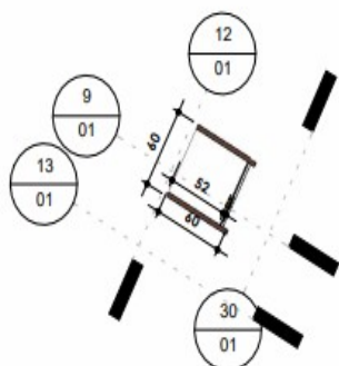
Planta de detalhe Pulpito | ESCALA: 1 : 50
