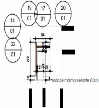
Detalhe do corte B | ESCALA: 1 : 50
