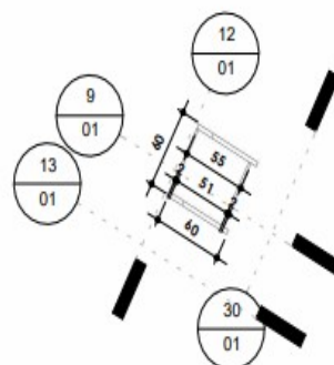
Elevação de topo | ESCALA: 1 : 50
