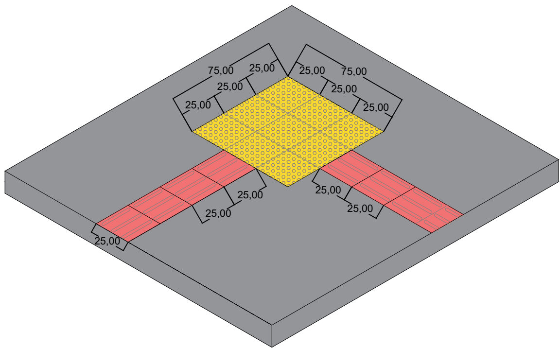
DETALHE PISO TÁTIL
