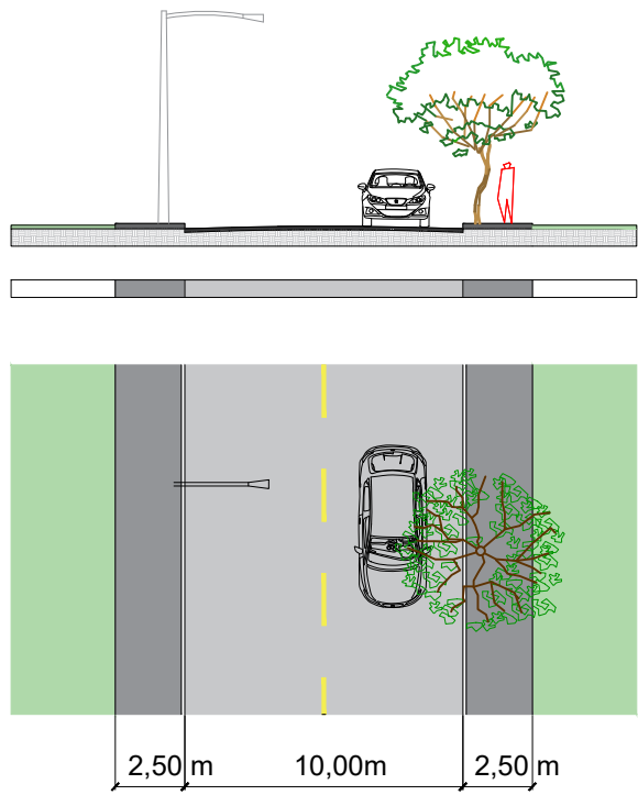
RUAS COM 10 M
