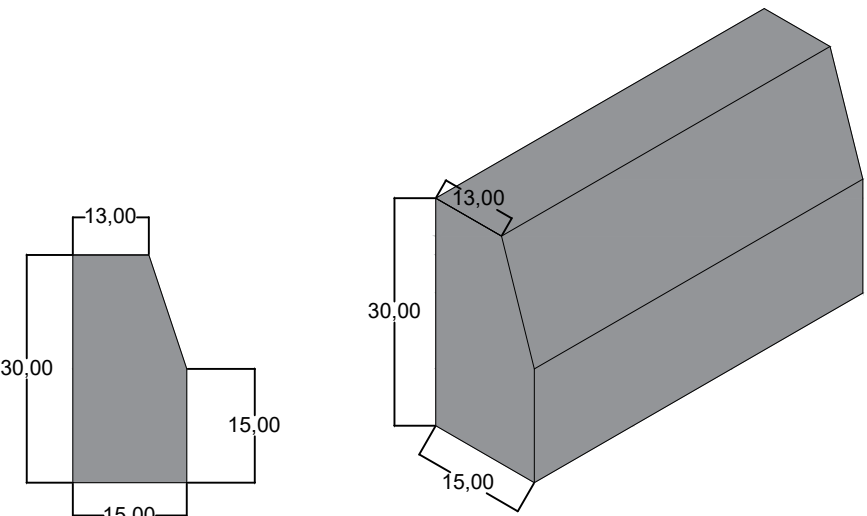
DETALHE MEIO-FIO EM CONCRETO PRÉ-MOLDADO
