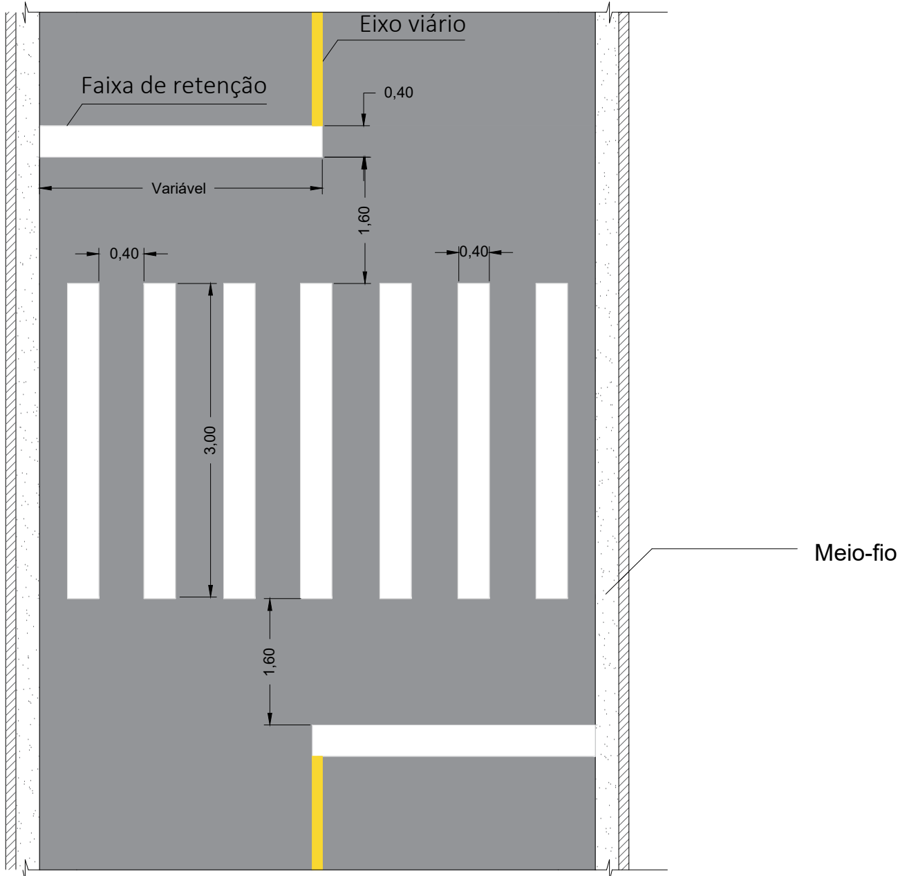
DETALHAMENTO 1 FAIXA DE PEDESTRE
