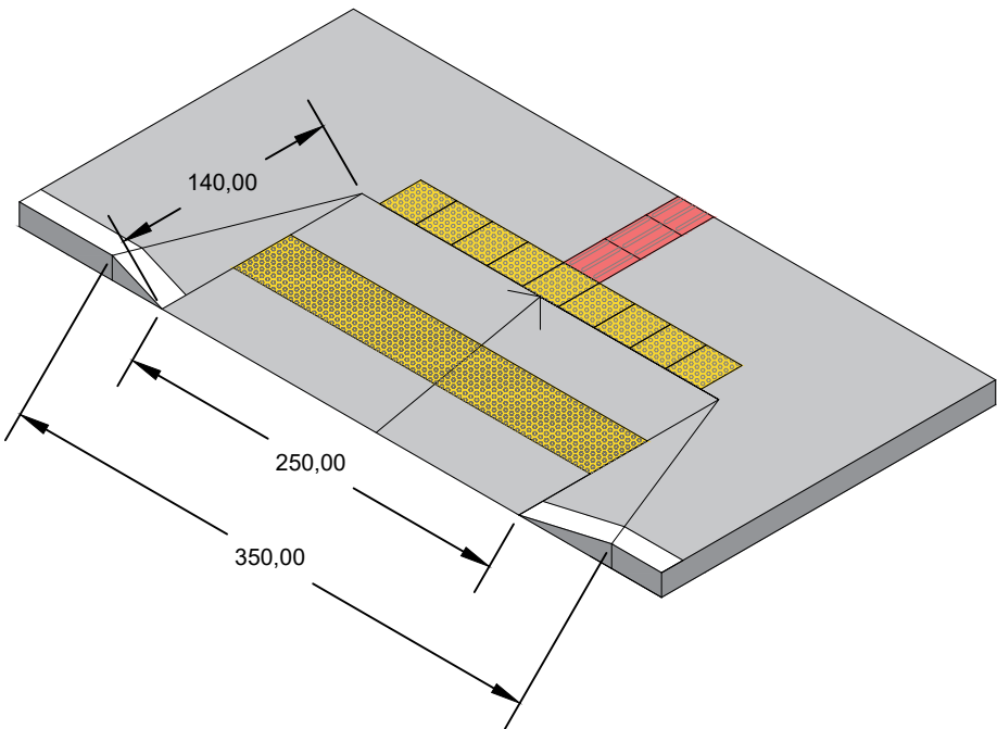
DETALHE RAMPA ACESSIBILIDADE
