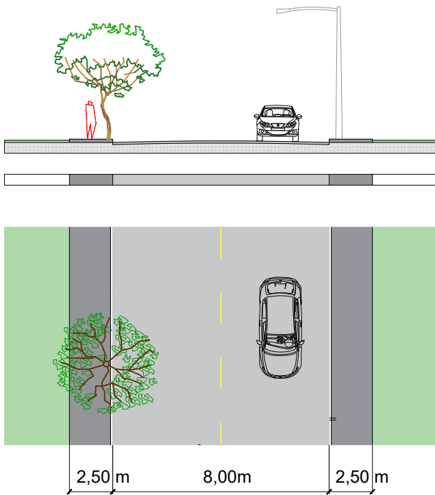
RUAS COM 8 M
