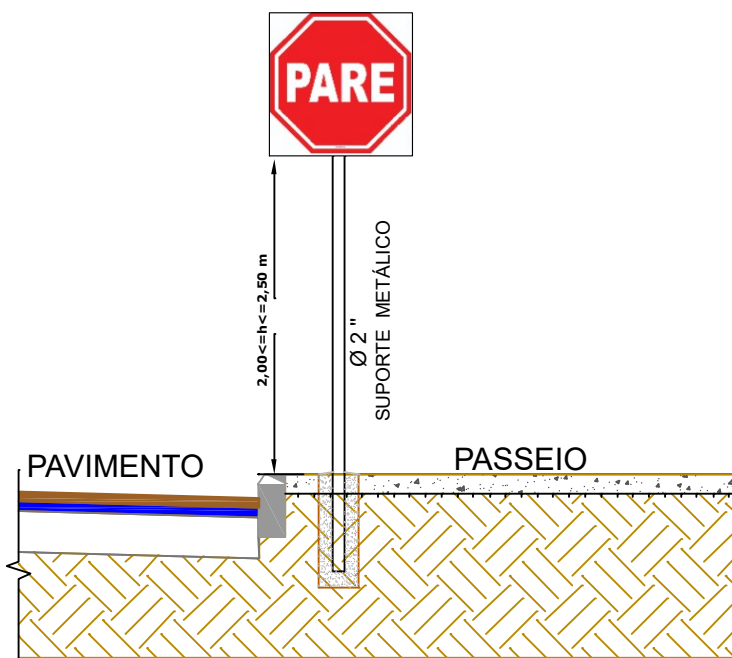
DETALHE INST. PLACAS DE SINALIZAÇÃO SEM ESCALA
