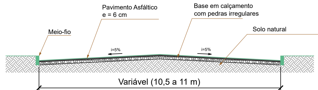
SEÇÃO TRANSVERSAL "BB" Sem escala
