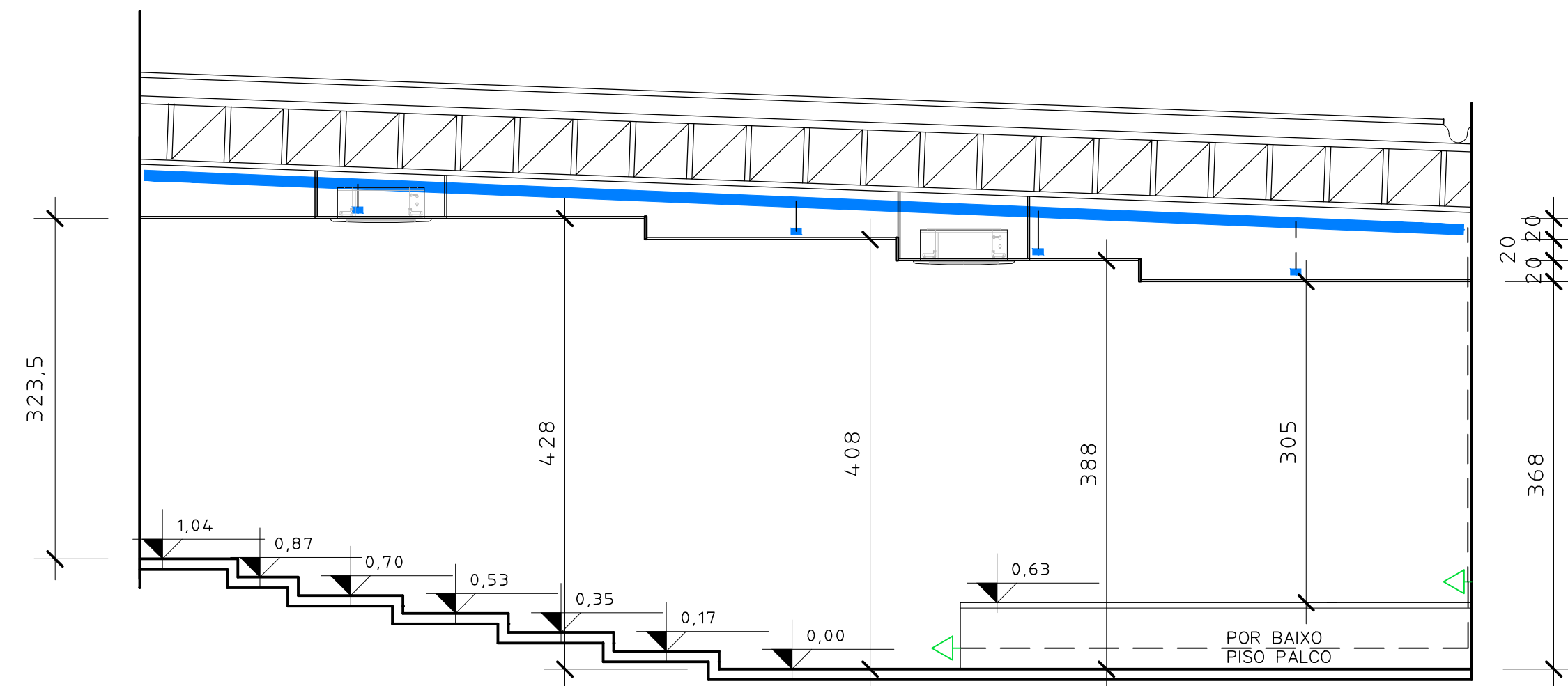
Corte Escala: 1/50
