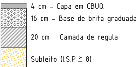
CORTE B-B' (PISTA)
