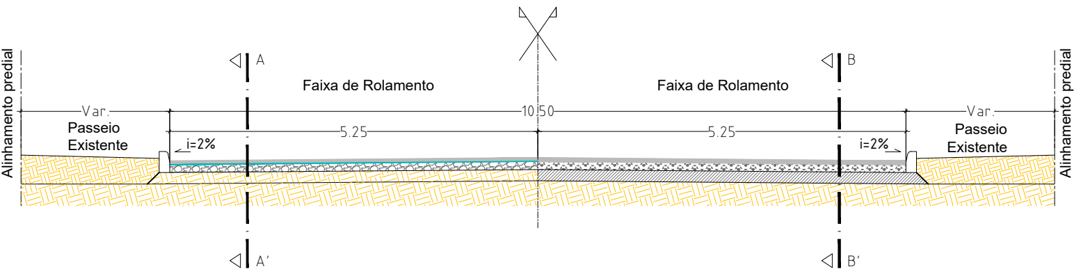
CORTE B-B' (PISTA)
