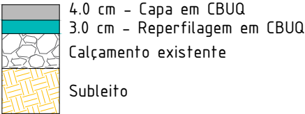
CORTE A-A' (PISTA)
