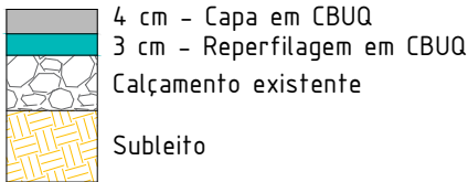
CORTE A-A' (PISTA)
