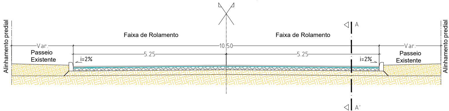
CORTE A-A' (PISTA)
