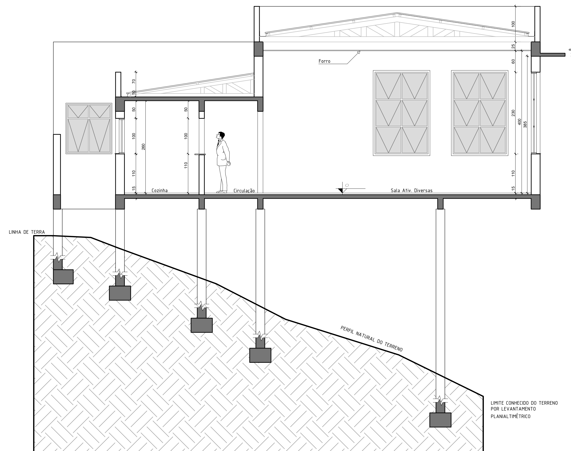
CORTE CC' ESC: 1/50
