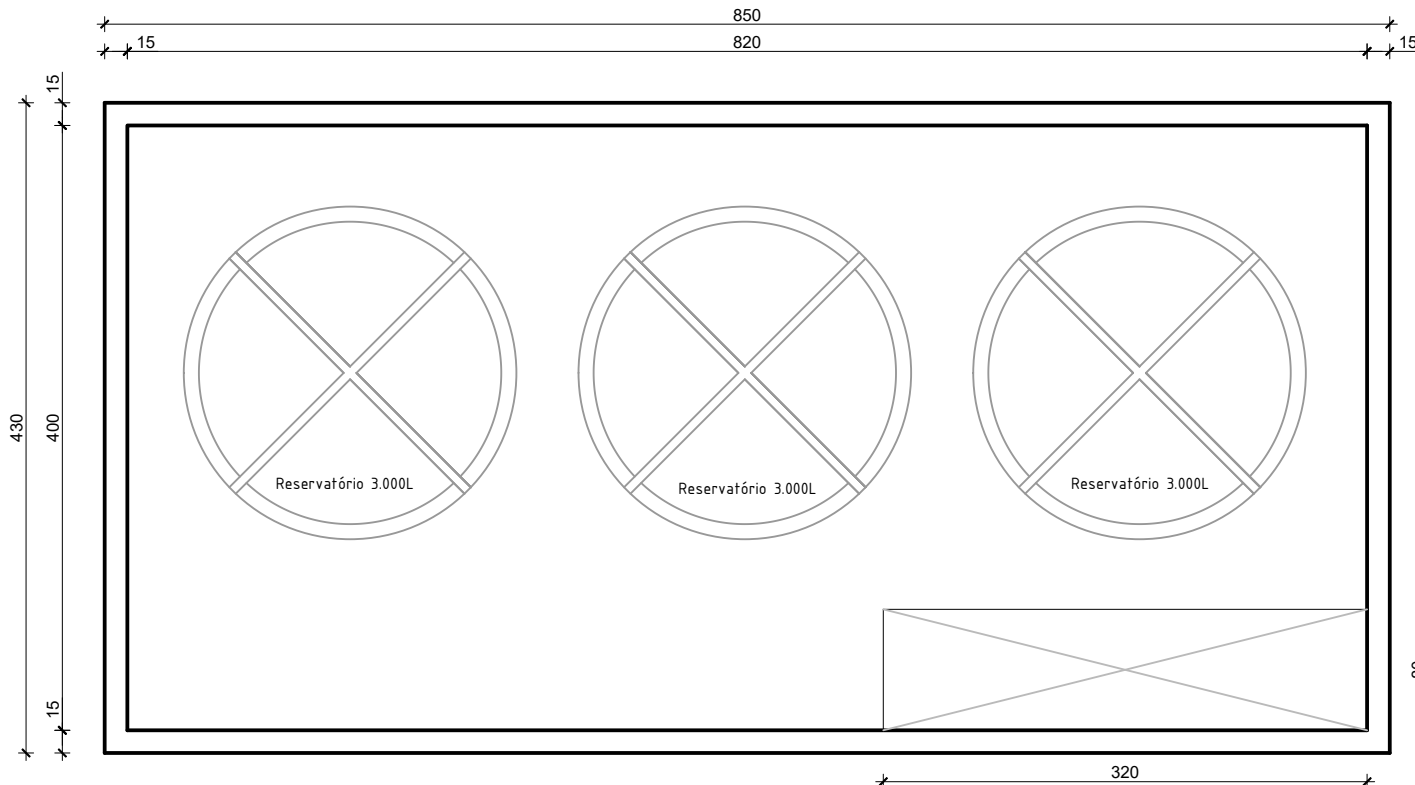
PLANTA BAIXA RESERVATÓRIO SUPERIOR ESC: 1/50
