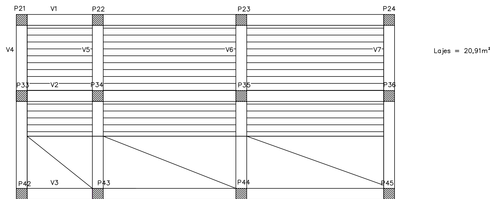
PLANTA BAIXA – VIGAS DE AMARRAÇÃO E LAJE DOS RESERVATÓRIOS ESC: 1/50
