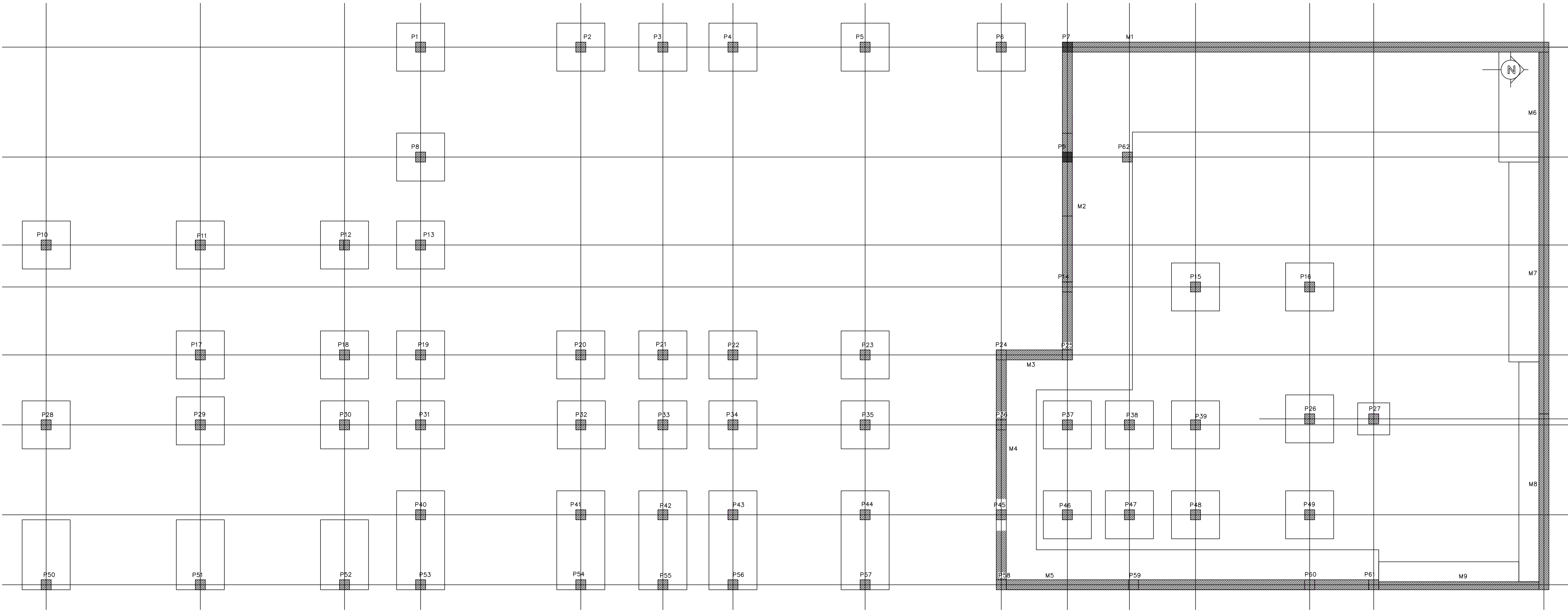
PLANTA BAIXA – SAPATAS E PILARES ESC: 1/50
