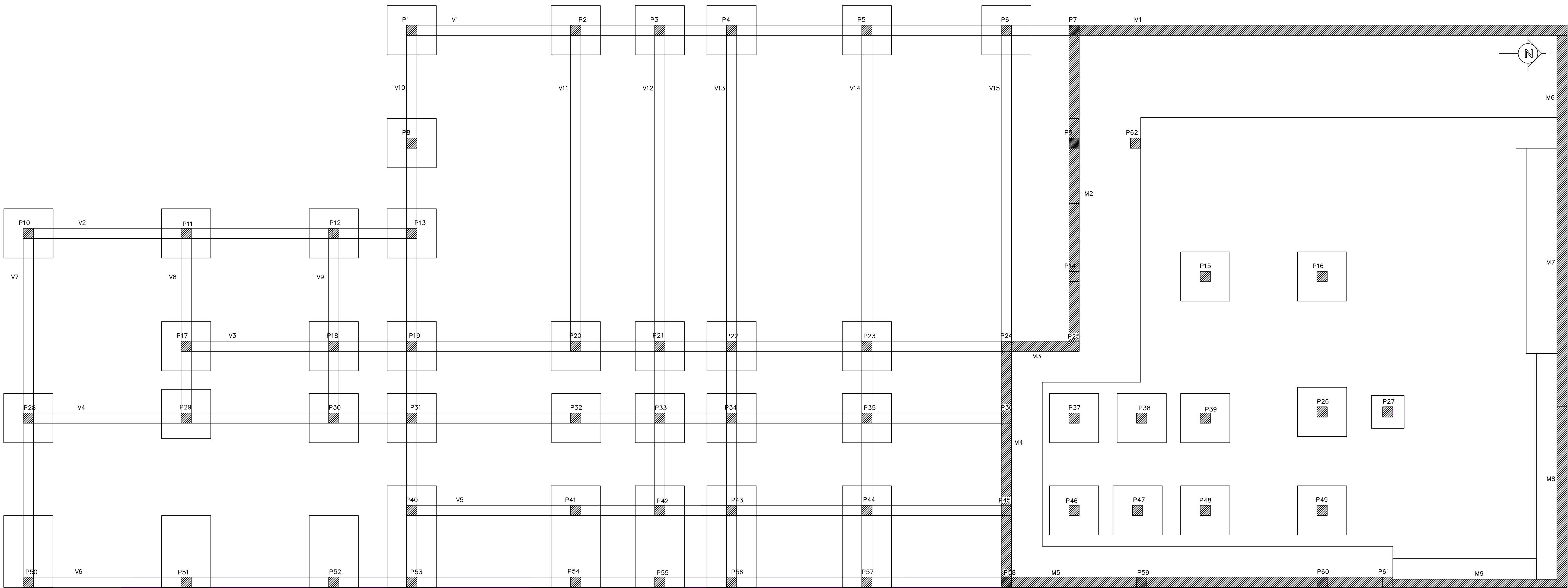
PLANTA BAIXA – SAPATAS E VIGAS BALDRAME – SUBSOLO ESC: 1/50
