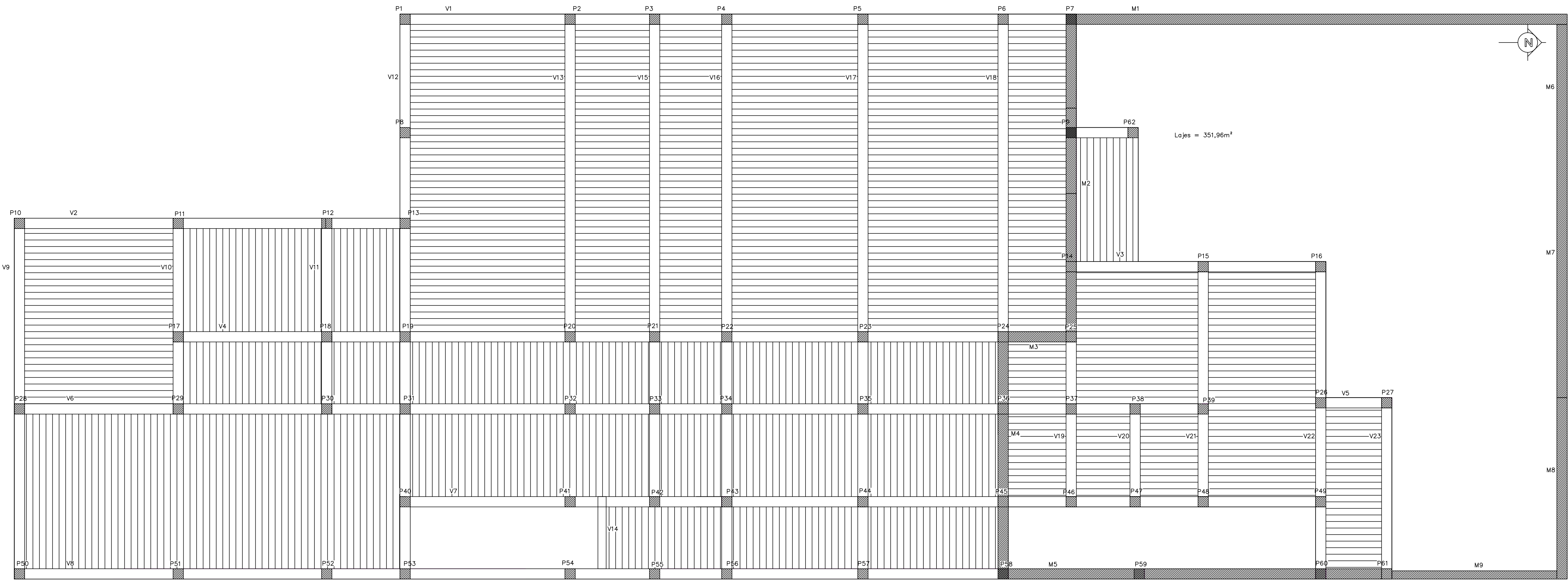
PLANTA BAIXA – VIGAS DE TRANSIÇÃO – TÉRREO ESC: 1/50
