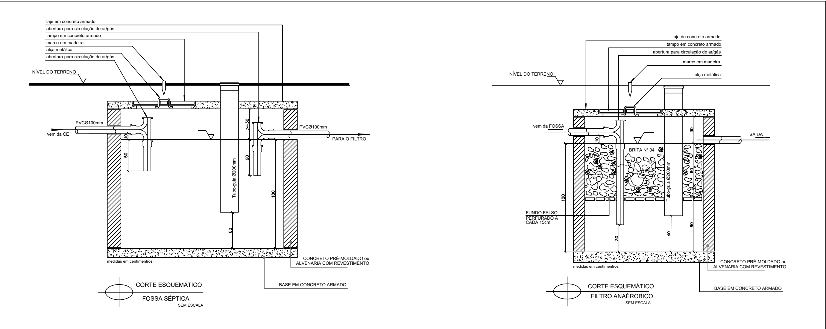
DETALHAMENTO DE FOSSA SÉPTICA E FILTRO ANAERÓBIO
