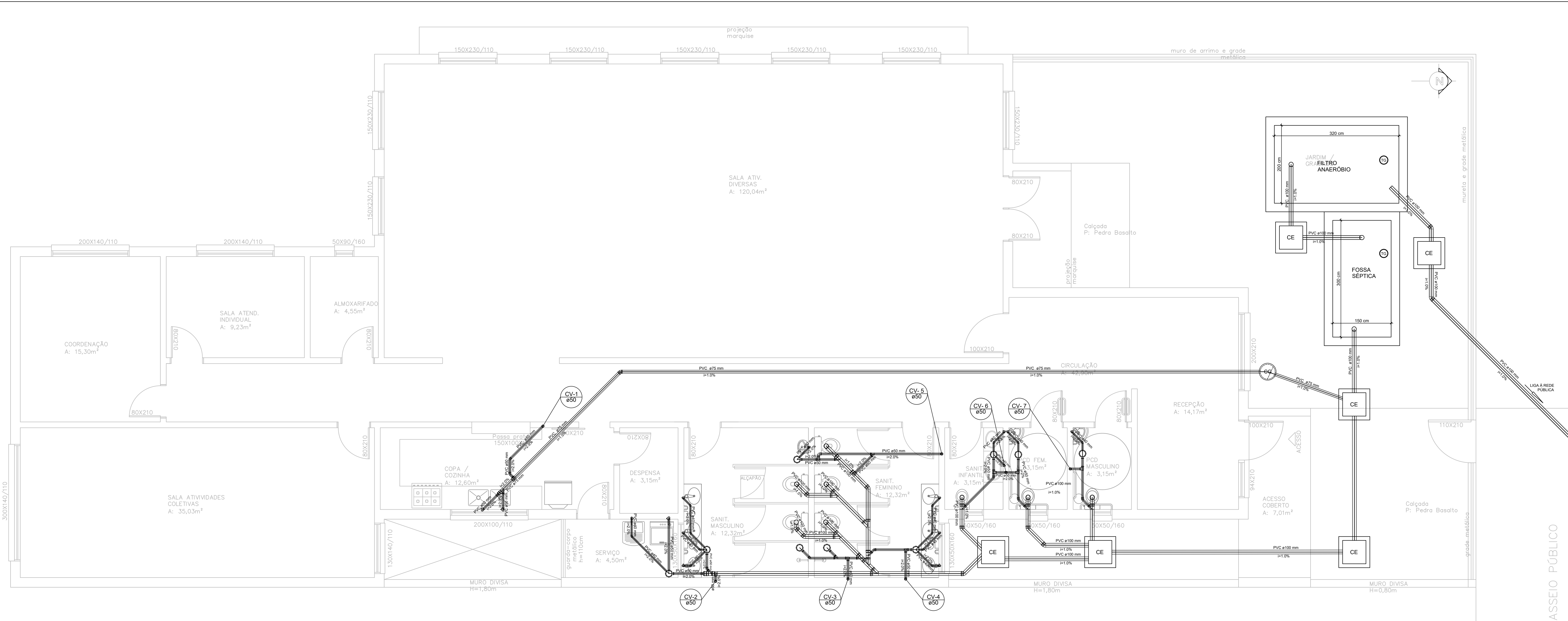
PLANTA BAIXA – INSTALAÇÕES DE ESGOTO SANITÁRIO A: 346,16m² Esc. 1:50
