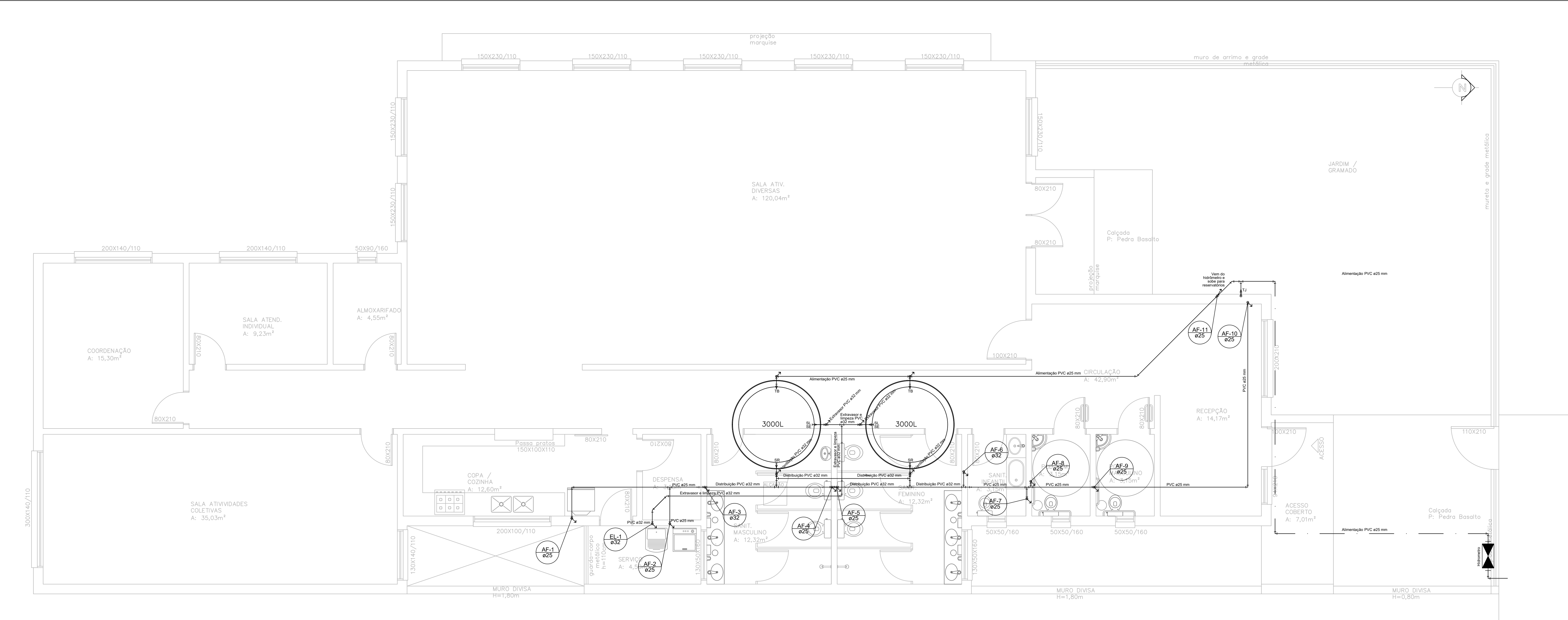
PLANTA BAIXA COM RESERVATÓRIOS E LIGAÇÕES DESDE O HIDRÔMETRO ATÉ AS PRUMADAS A: 346,16m² Esc. 1:50
