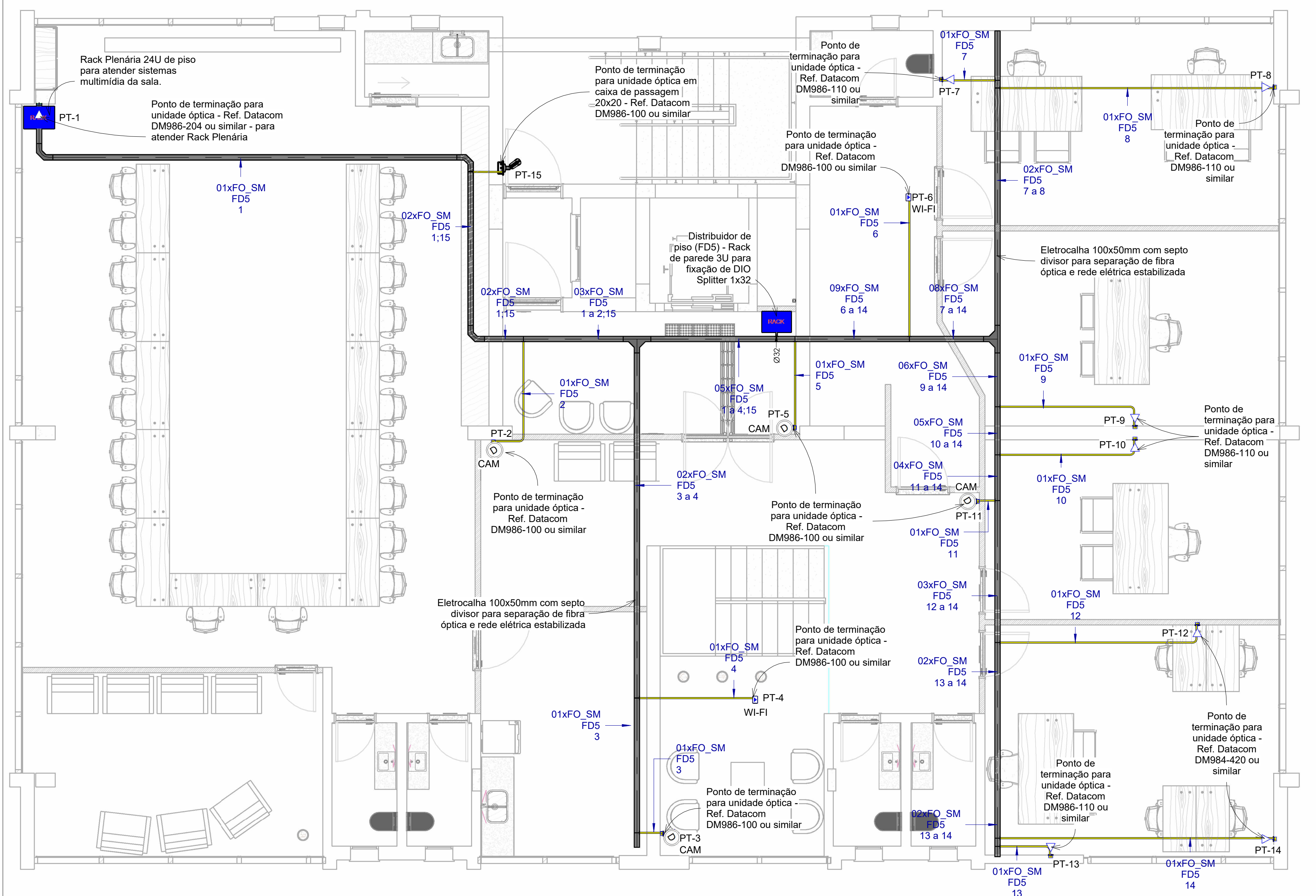
Pvto 5 (GPON)
