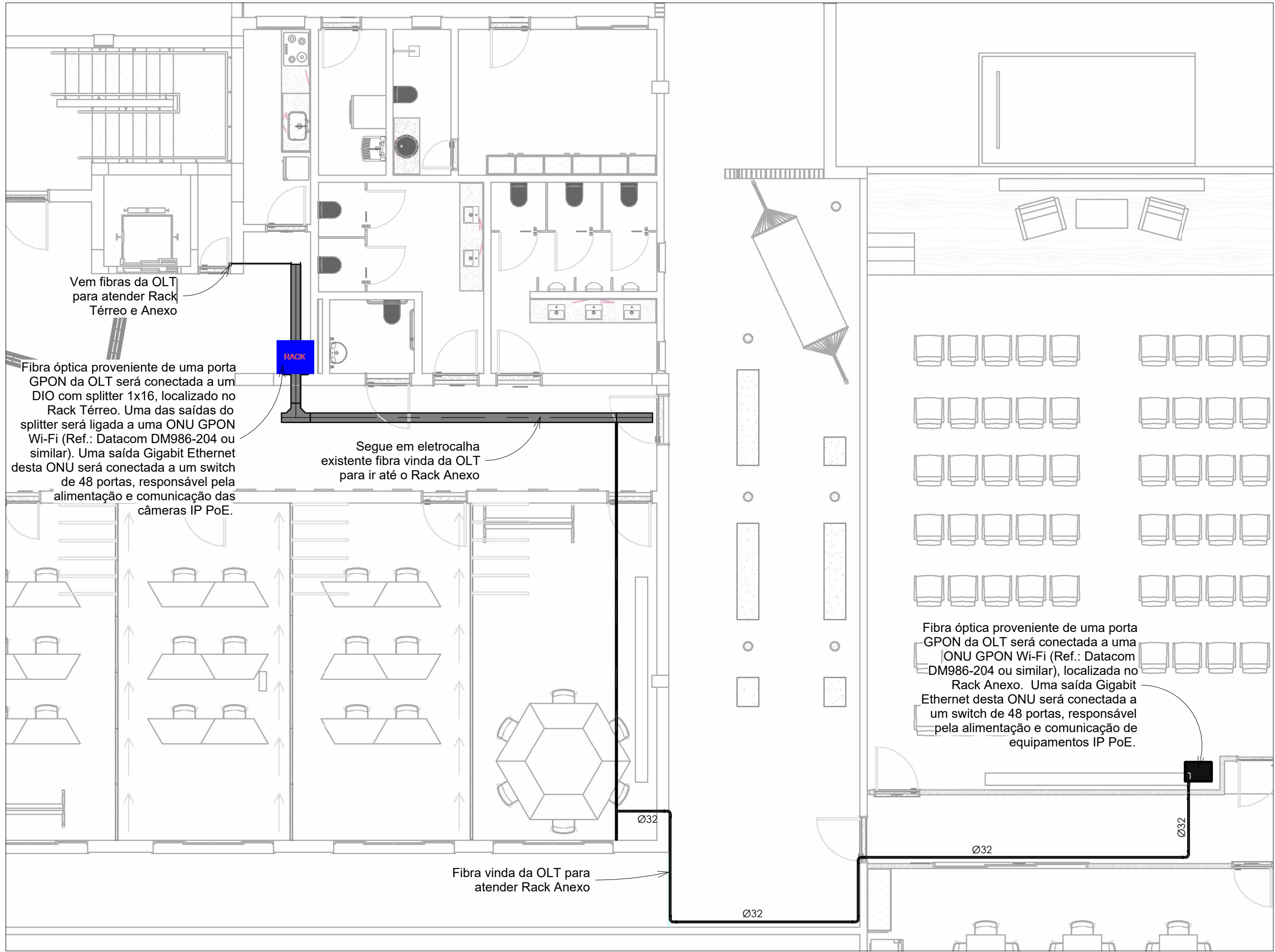
Térreo e Anexo (Implantação)
