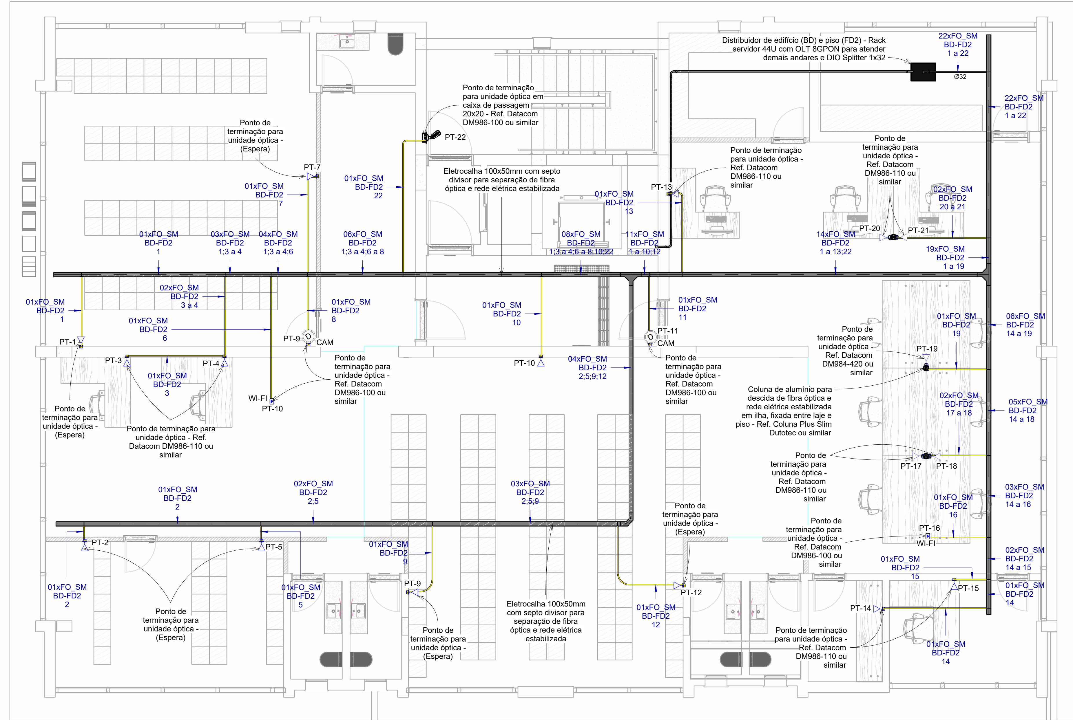
Pvto 2 (GPON)
