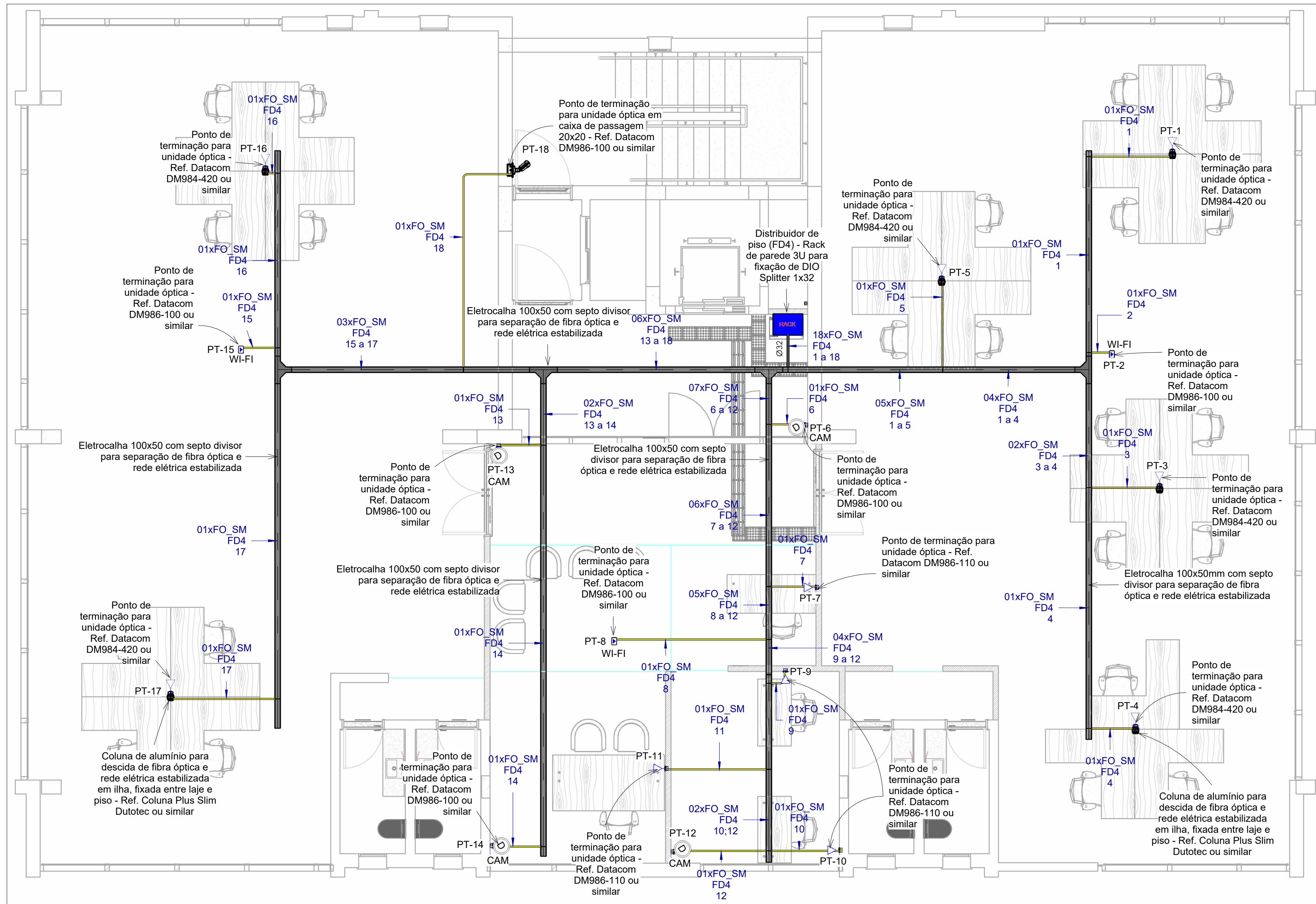
Pvto 4 (GPON)
