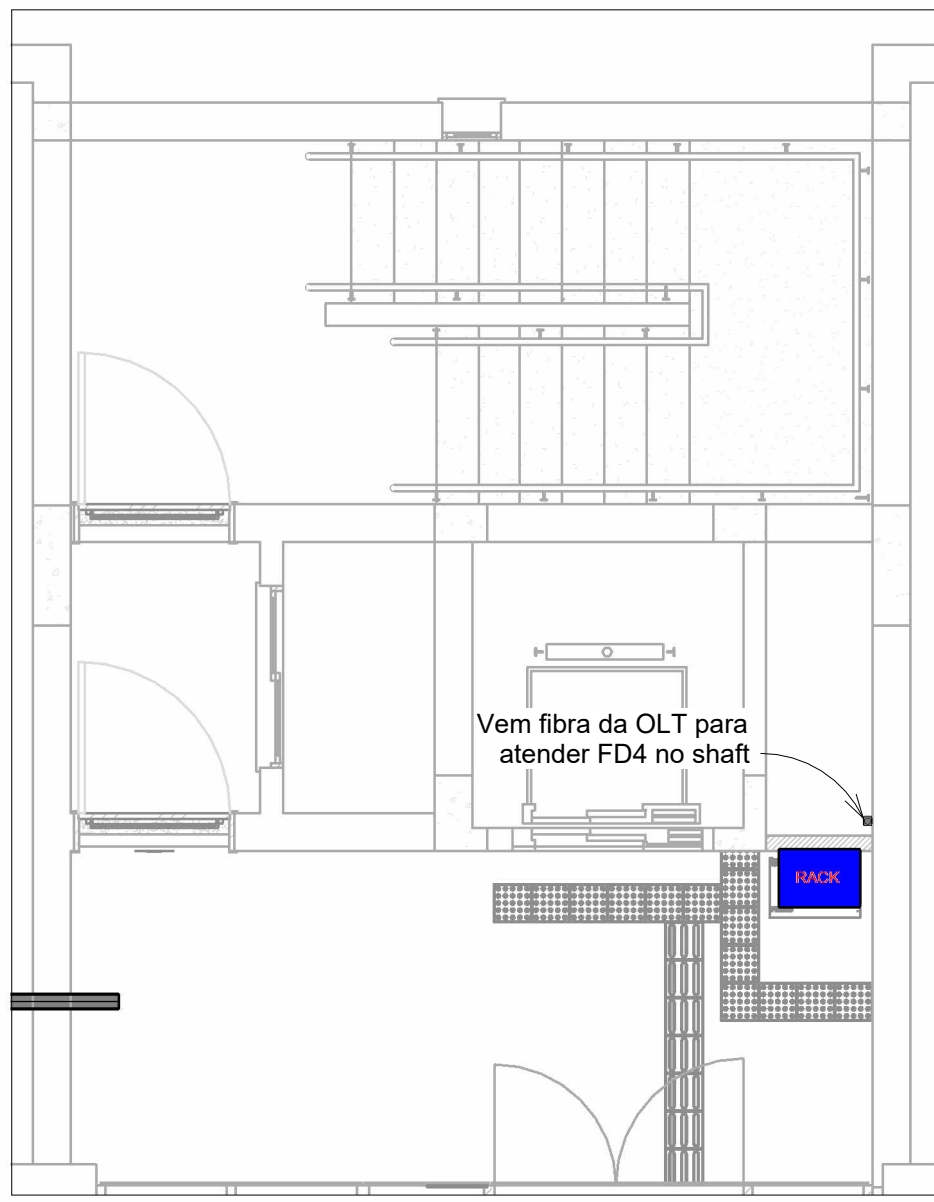
Ptvo 4 (Implantação)
