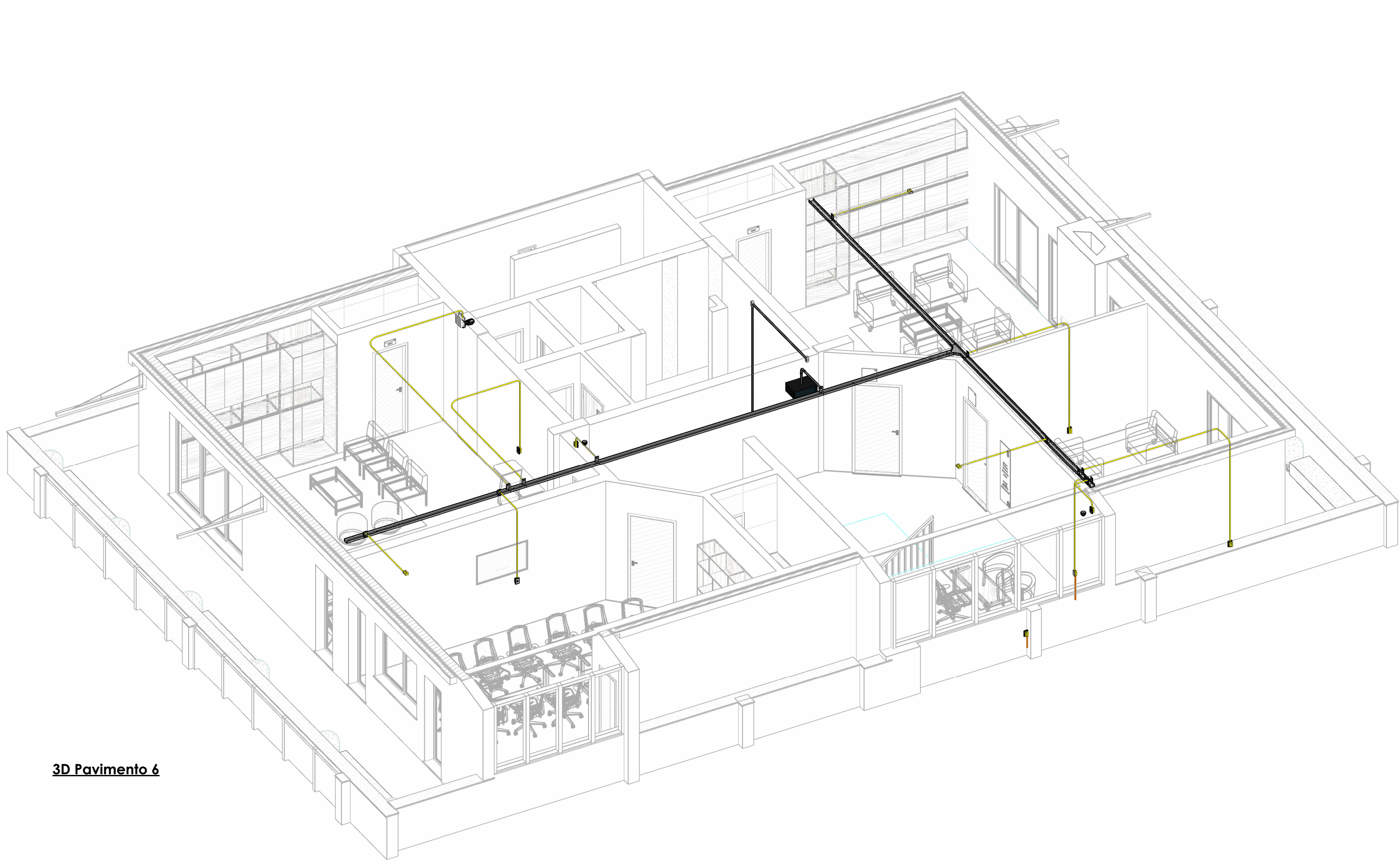
Pvto 6 (GPON)
