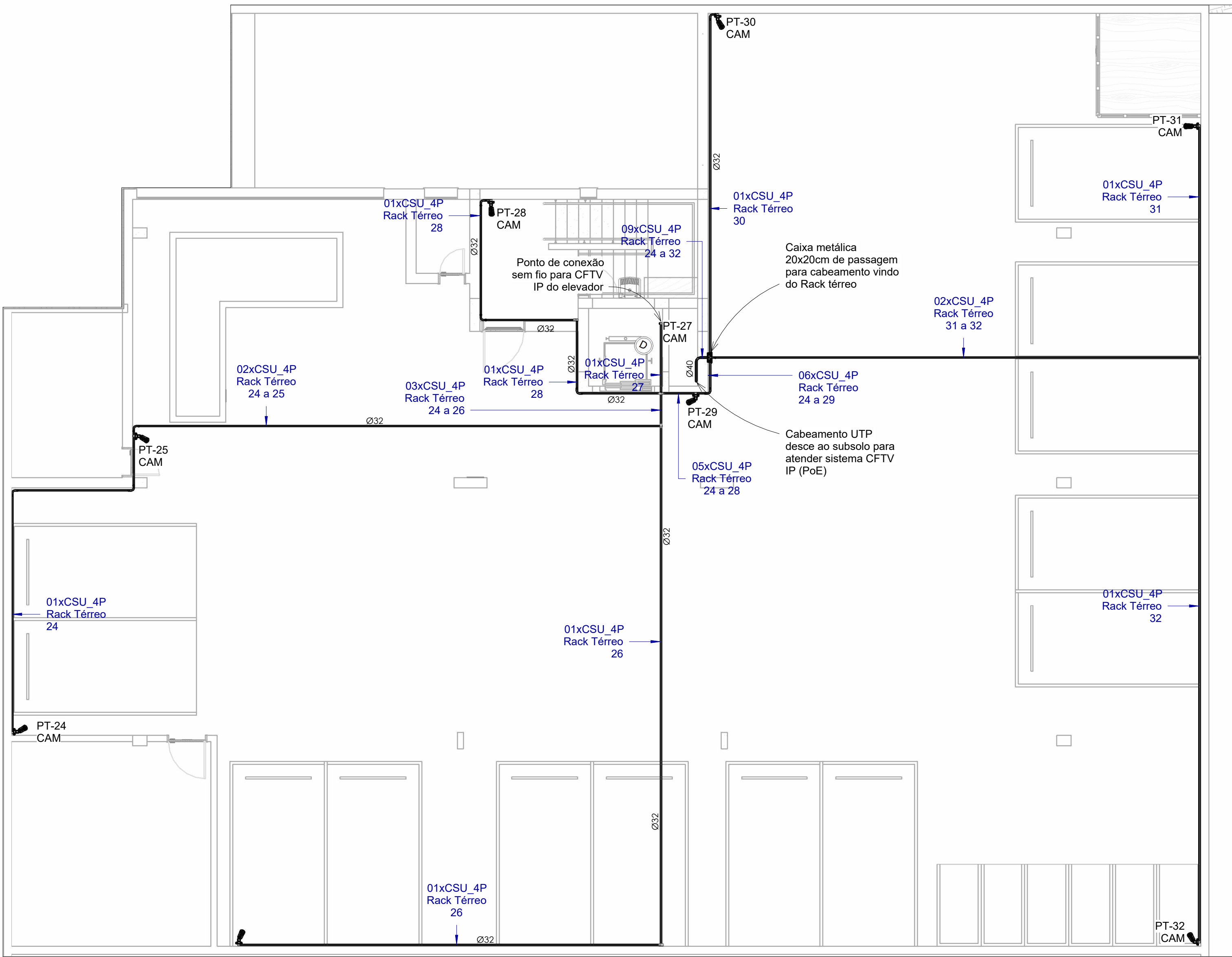
Subsolo (Cabeamento)
