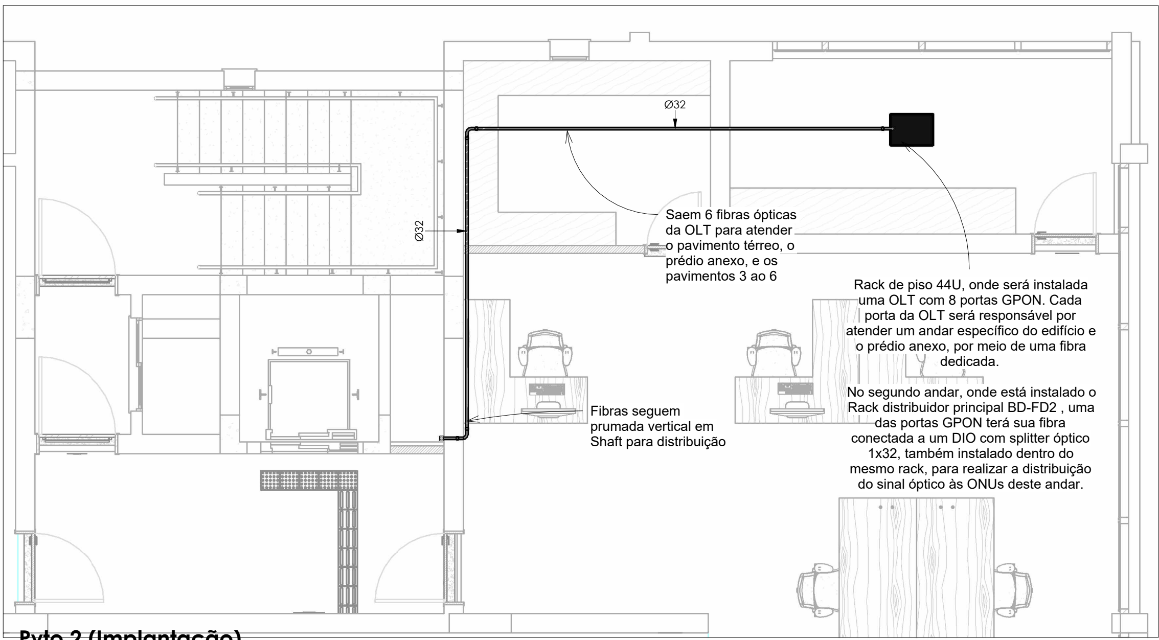
Ptvo 2 (Implantação)
