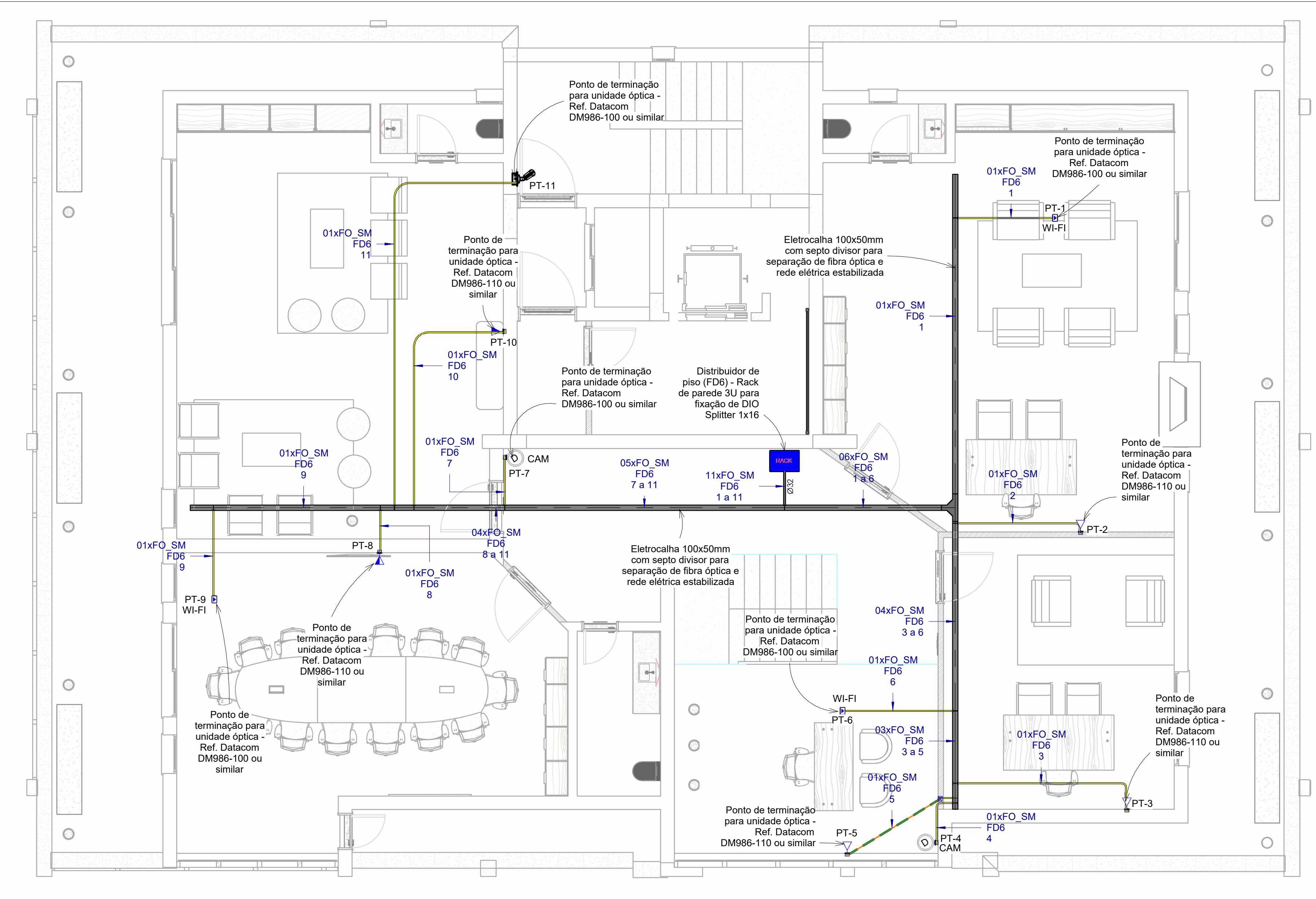
Pvto 6 (GPON)
