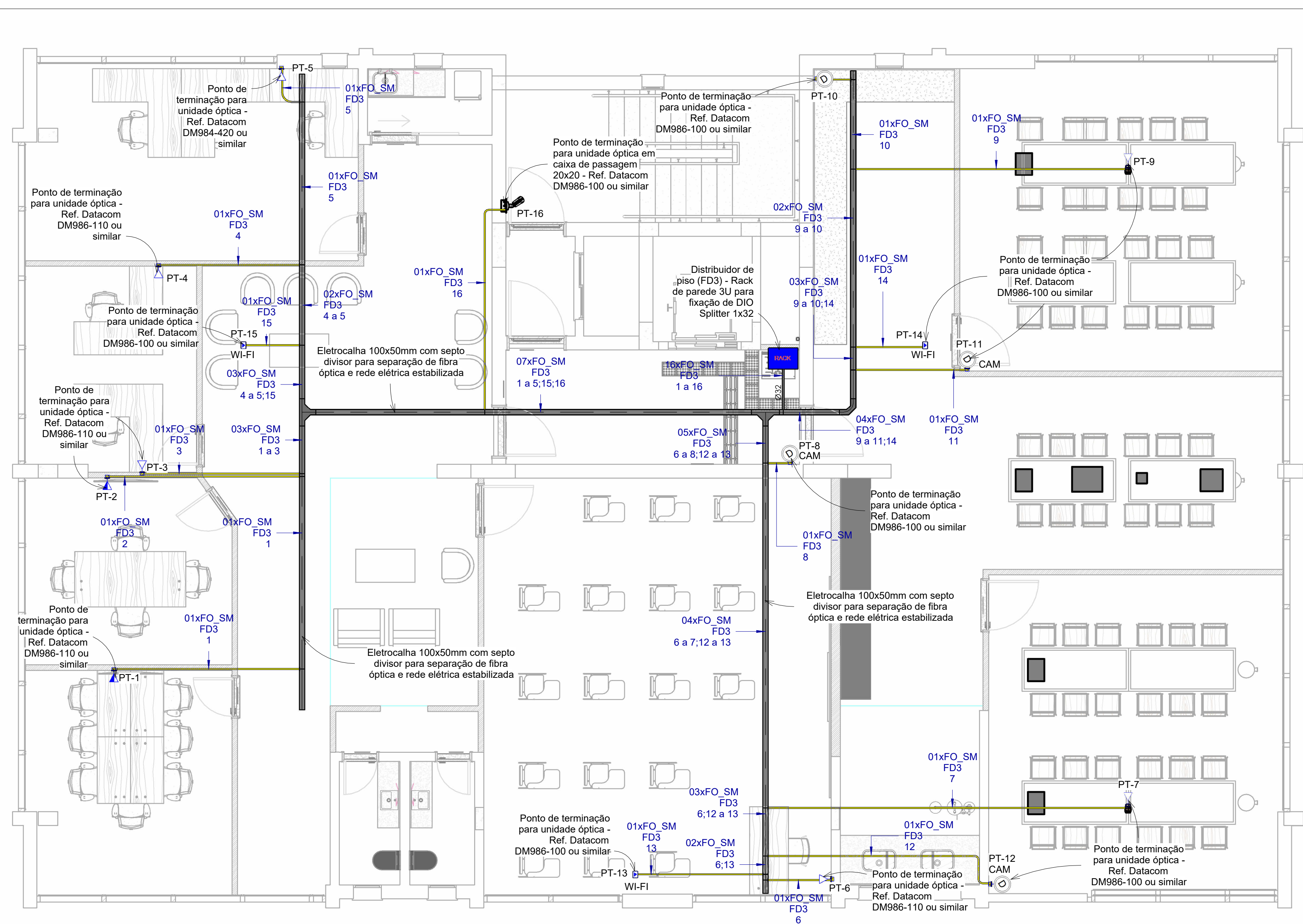
Pvto 3 (GPON)
