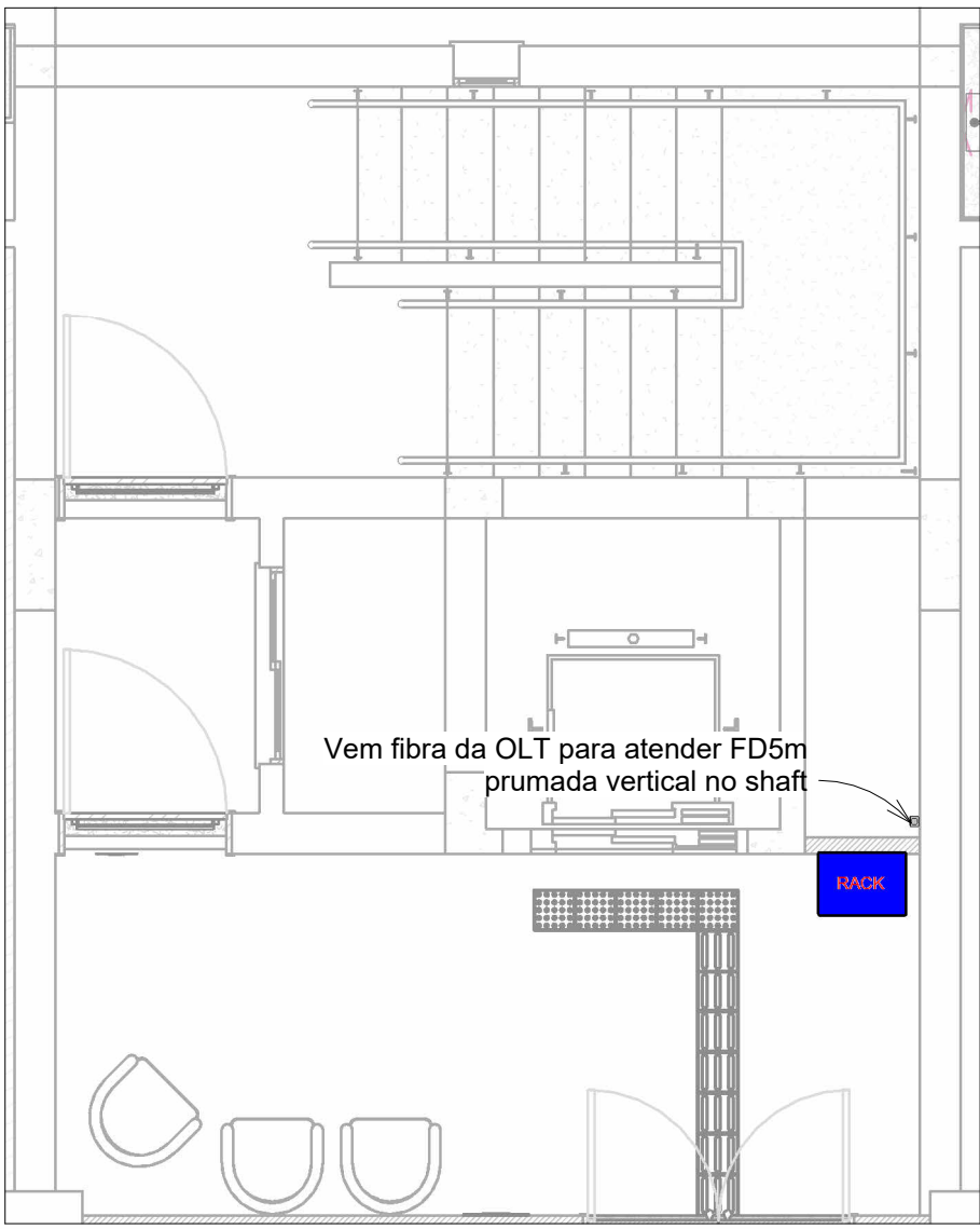
Ptvo 5 (Implantação)
