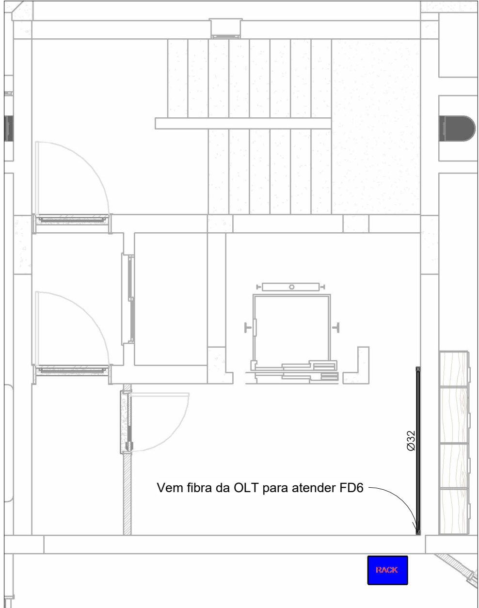
Ptvo 6 (Implantação)
