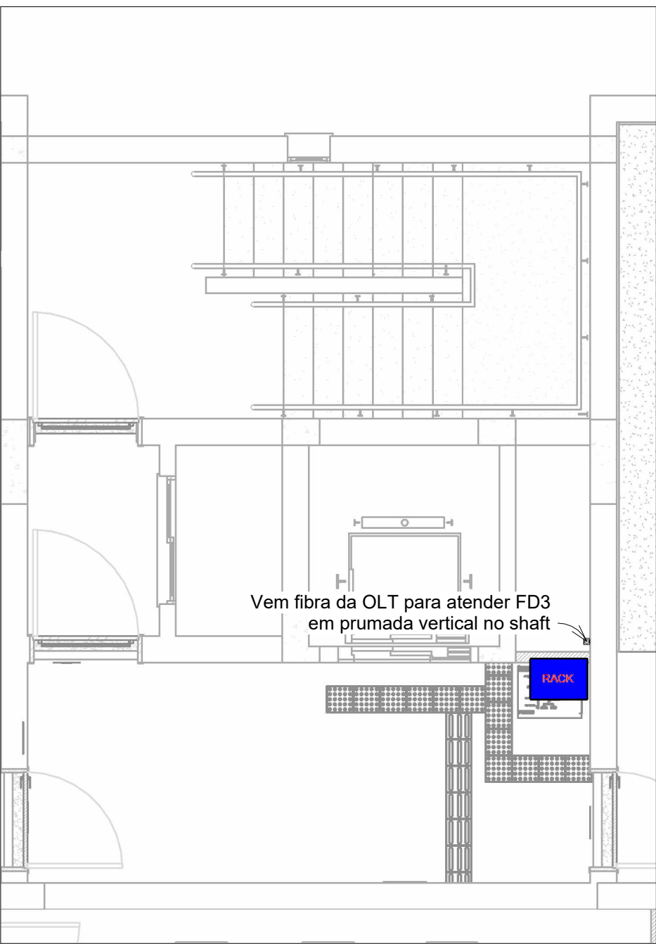
Ptvo 3 (Implantação)
