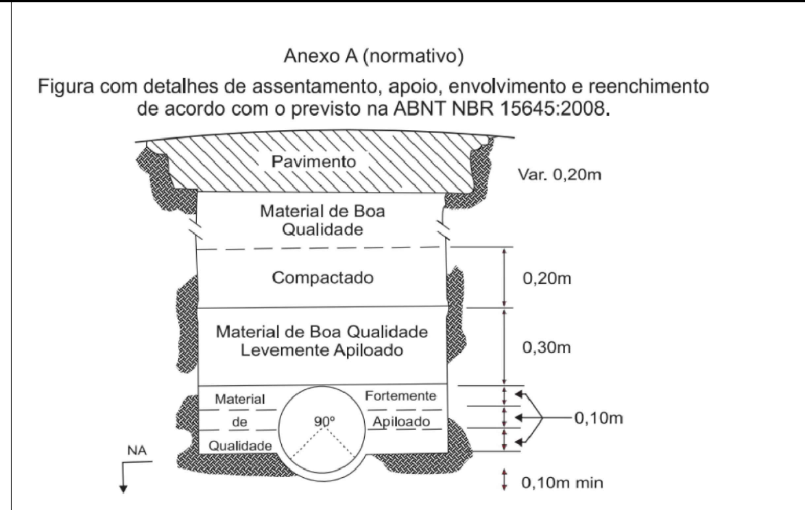
08 Assentamento de Tubos S/Escala
