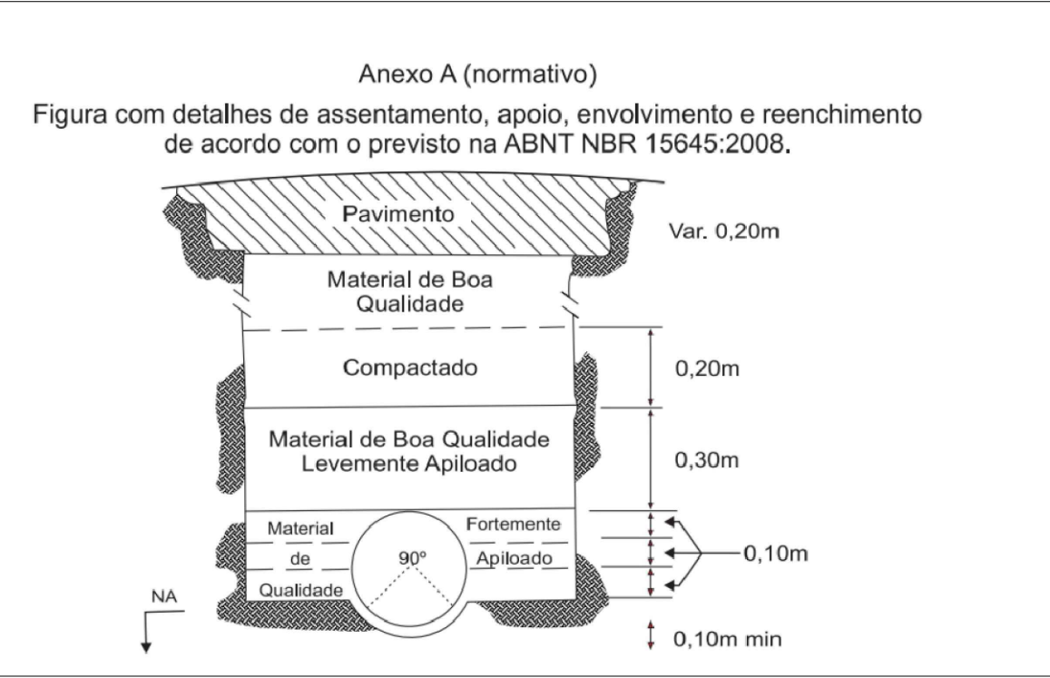
07 Assentamento de Tubos S/Escala
