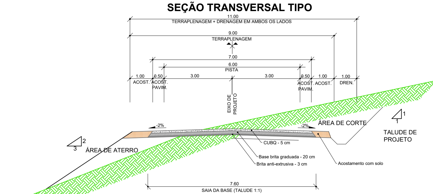
04 Seção Transversal Tipo Escala: 1/100
