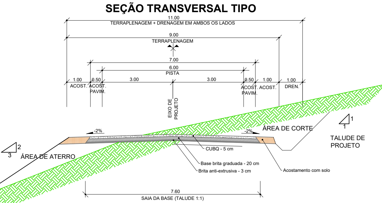
03 Seção Transversal Tipo Escala: 1/100
