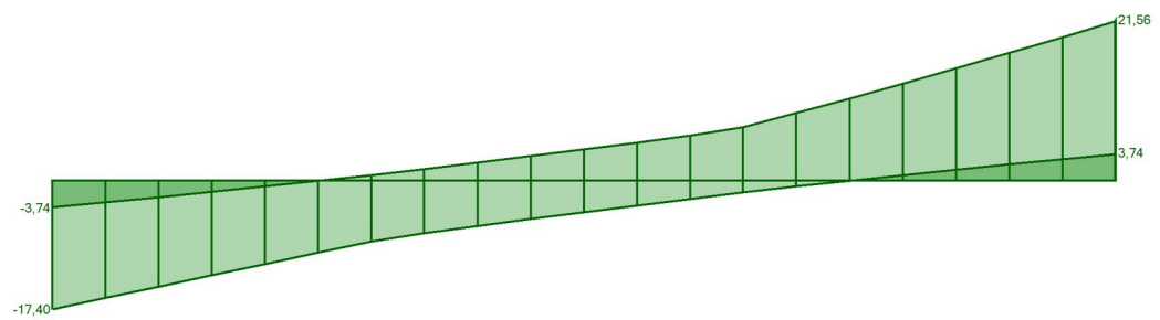
Envoltória de momento torçor combinação de cálculo: V3
