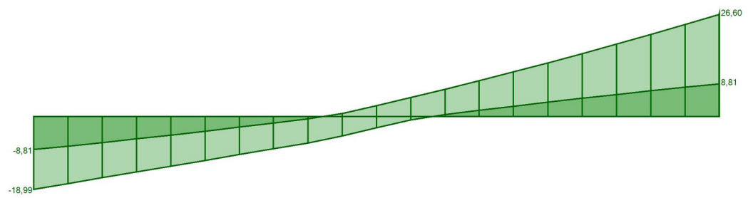
Envoltória de momento torçor combinação de cálculo: V2
