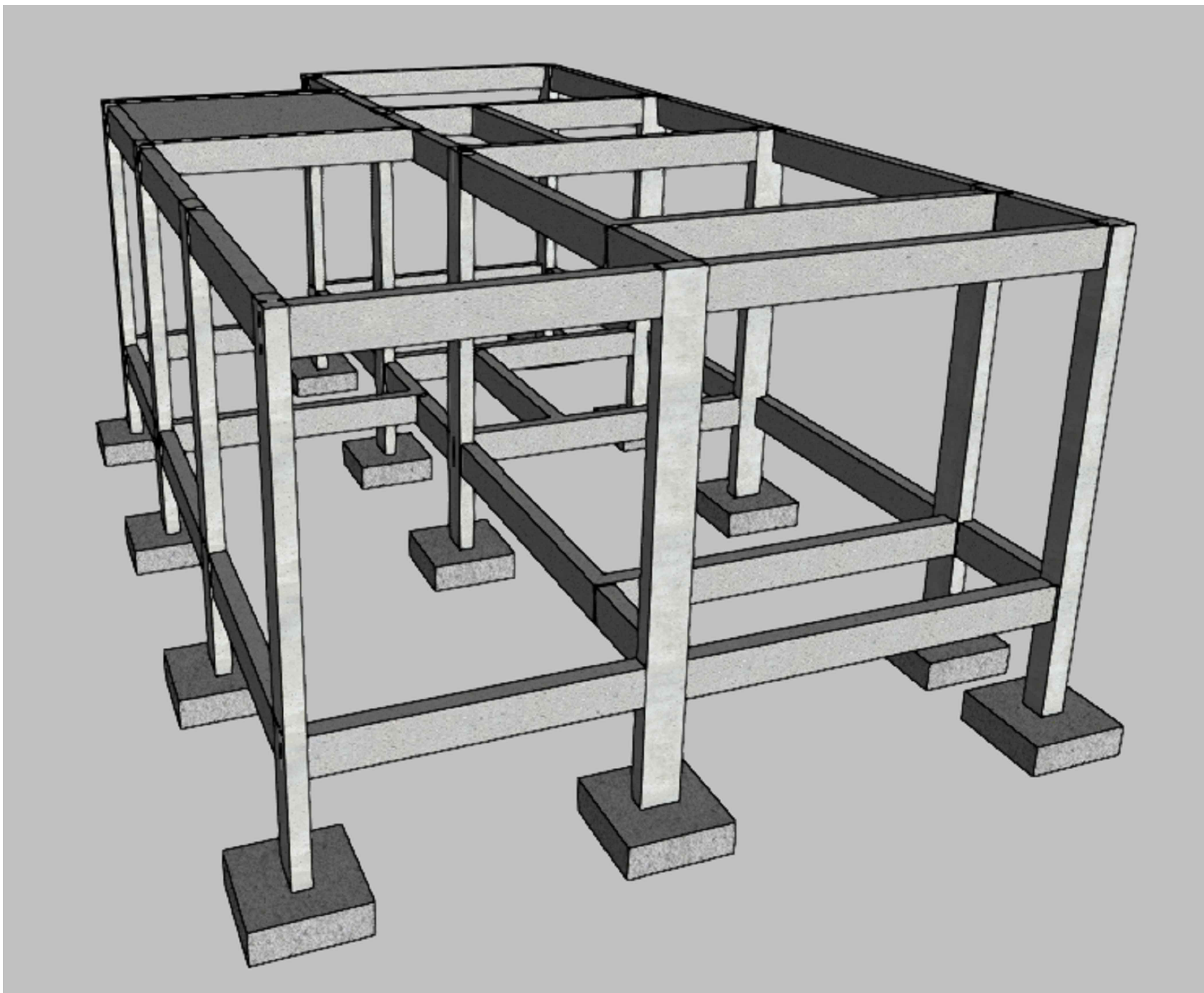
DETALHAMENTO 3D DA ESTRUTURA
