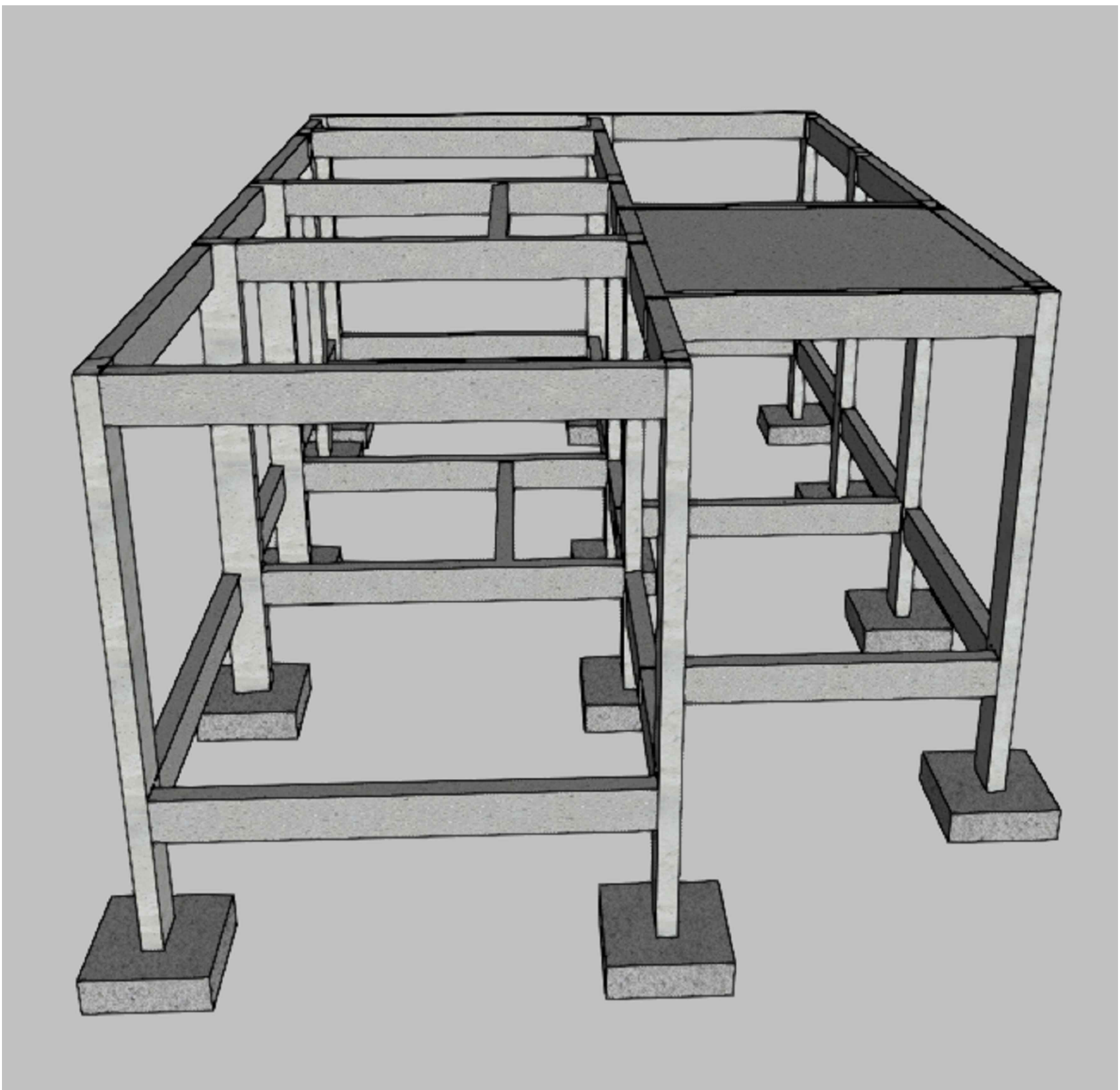
DETALHAMENTO 3D DA ESTRUTURA
