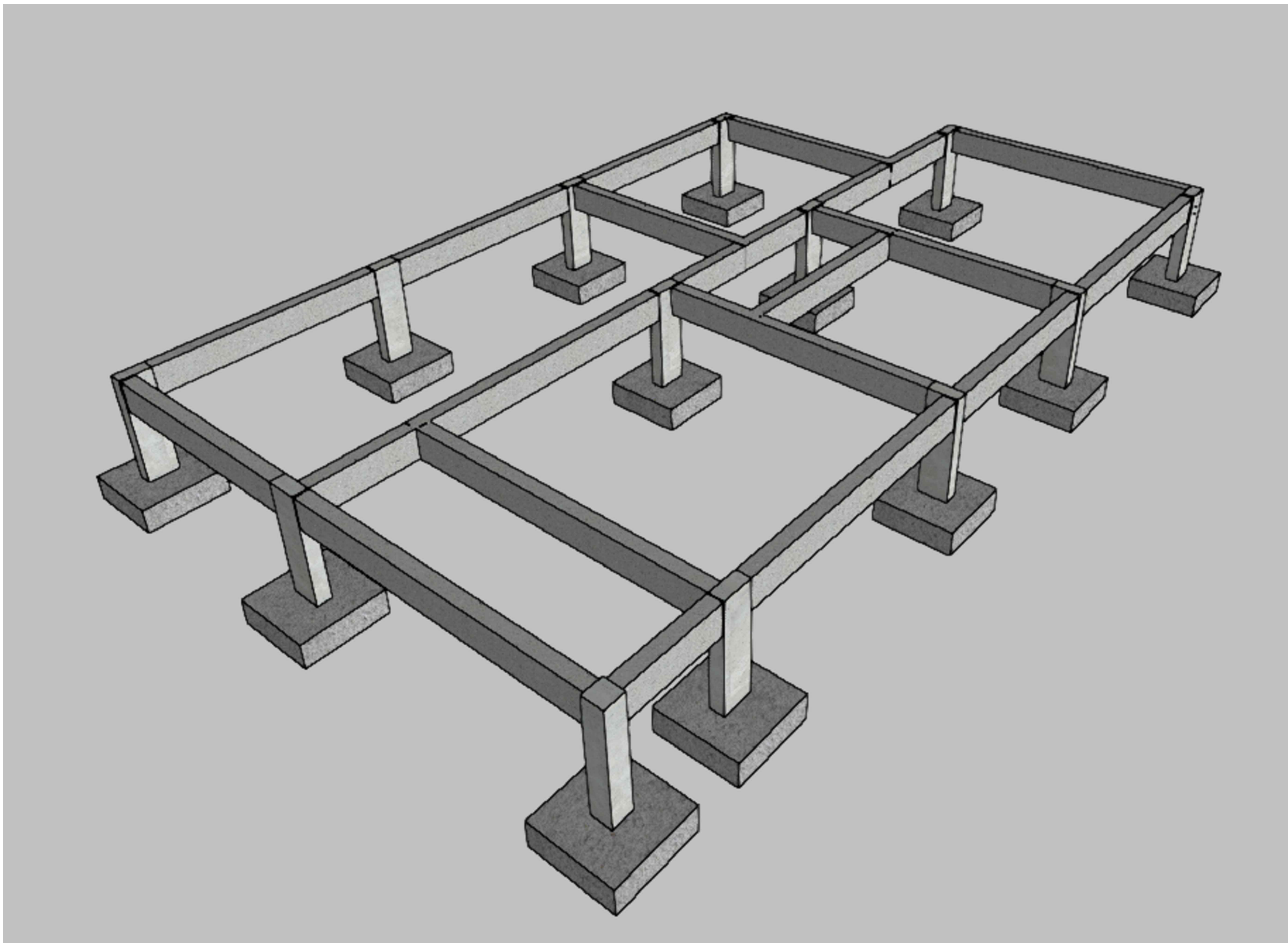
DETALHAMENTO 3D DA ESTRUTURA
