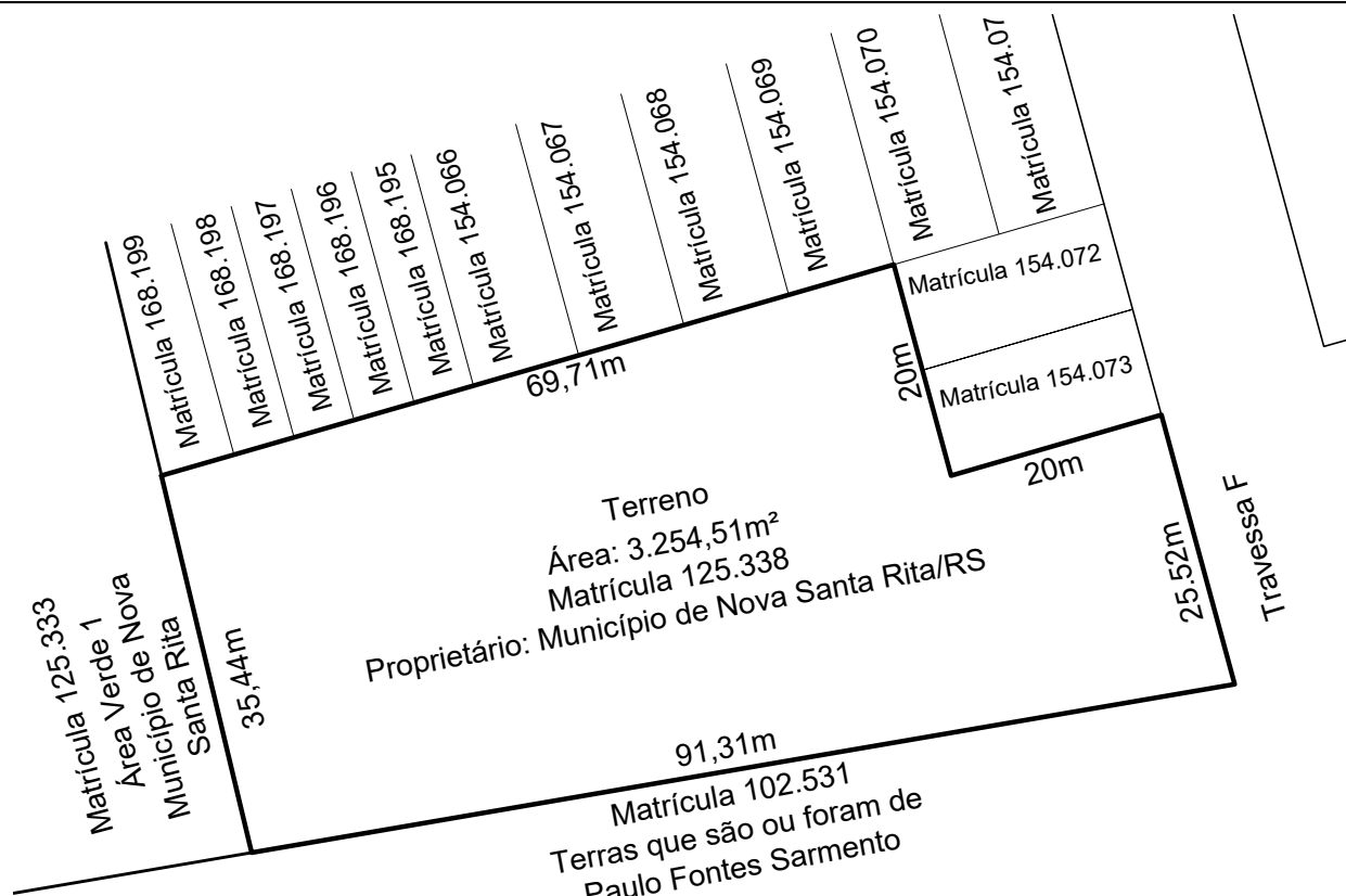
PLANTA DOS CONFORNTANTES ESCALA: 1/750
