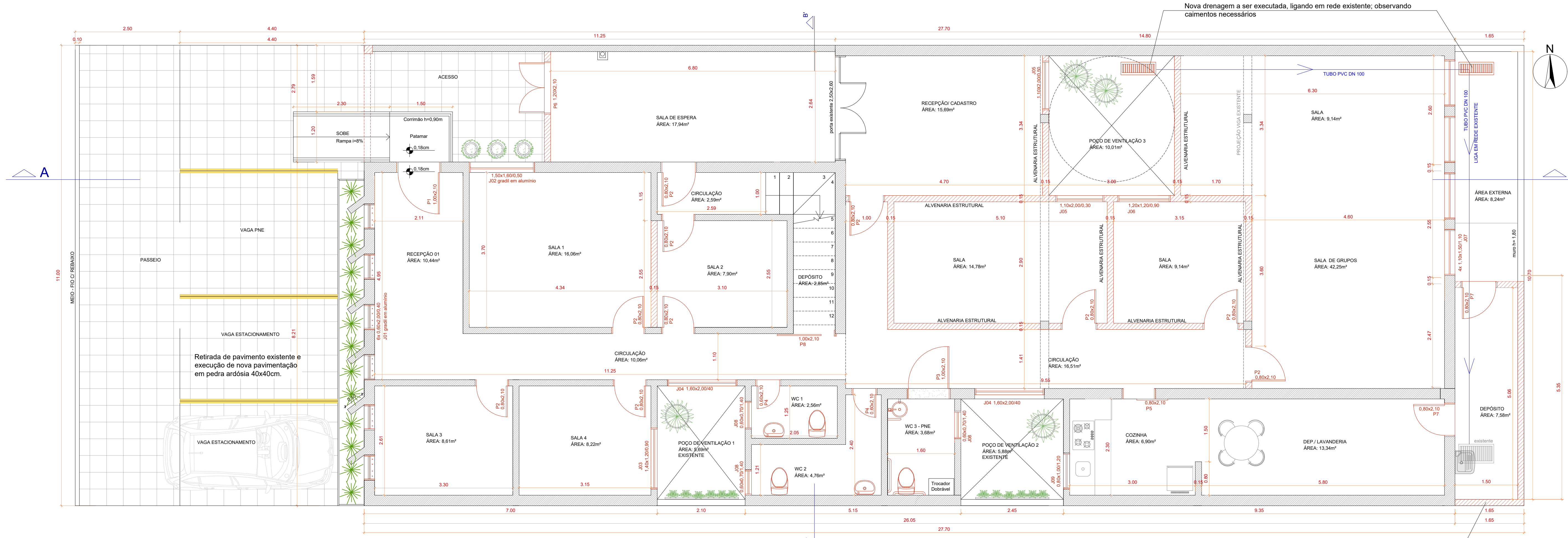
PLANTA BAIXA TÉRREO - INTERVENÇÕES ESC 1/50 ÁREA TOTAL TÉRREO: 272,37m²
