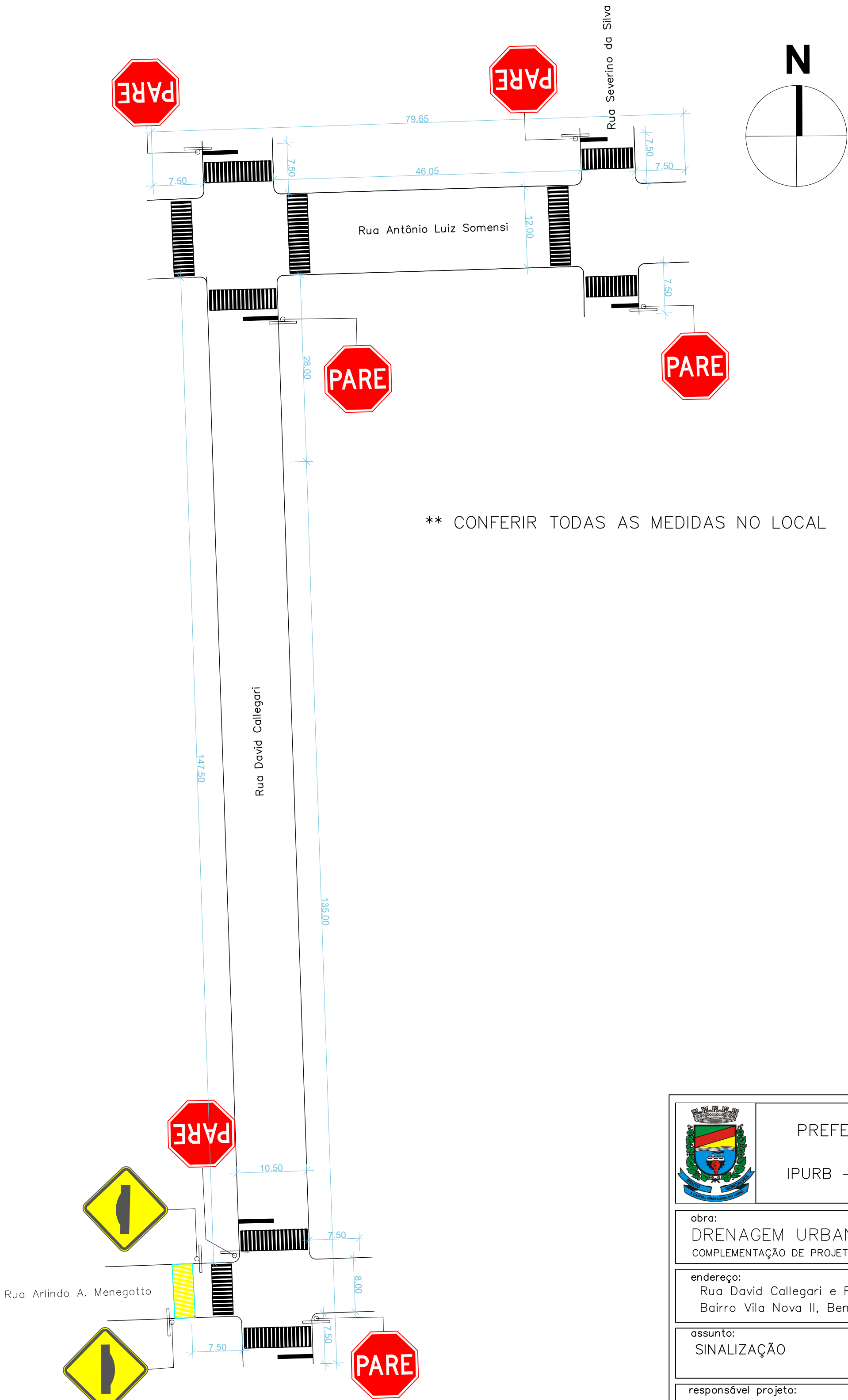
Projeto de Sinalização Escala 1:500
