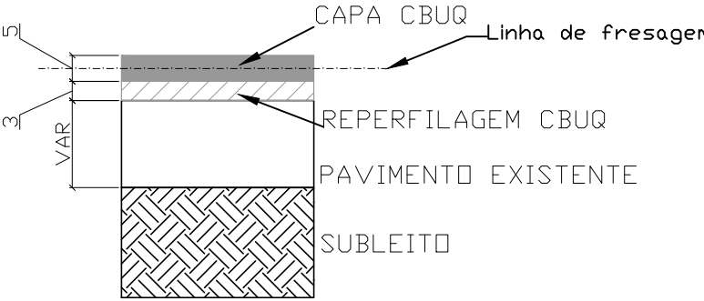
Detalhe 1 Seção do pavimento
