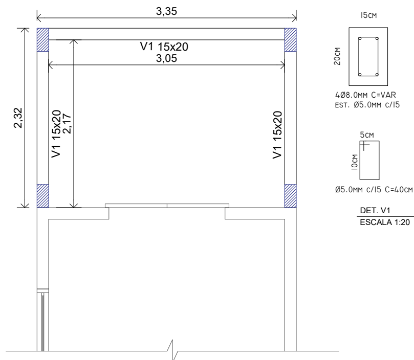
VIGAS DE CINTAMENTO ESC 1/50
