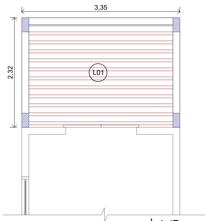
VIGAS DE CINTAMENTO ESC 1/50
