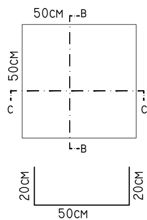
DET. BLOCOS DE COROAMENTO
