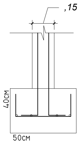
CORTE BB
