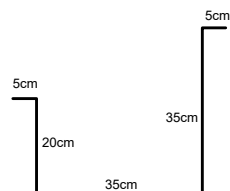
RUFO CORTE 25
