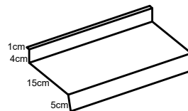
PINGADEIRA CORTE 25
