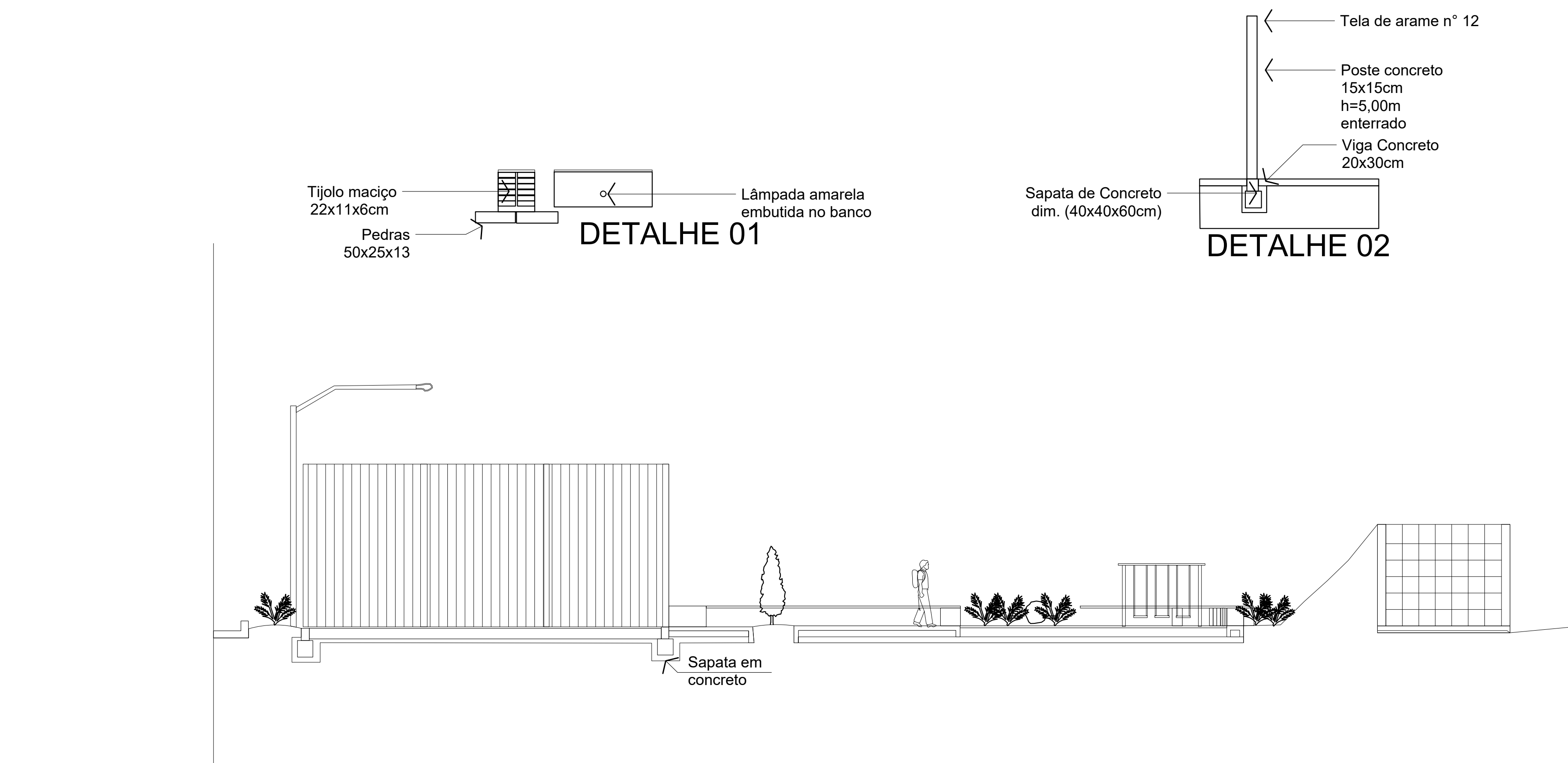
CORTE BB ESC 1/125
