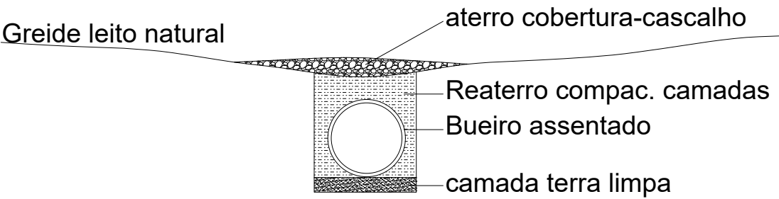
VISTA em Perfil Bueiros - Zona rural
