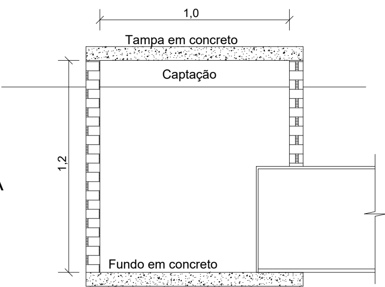
VISTA EM CORTE Sem Escala
