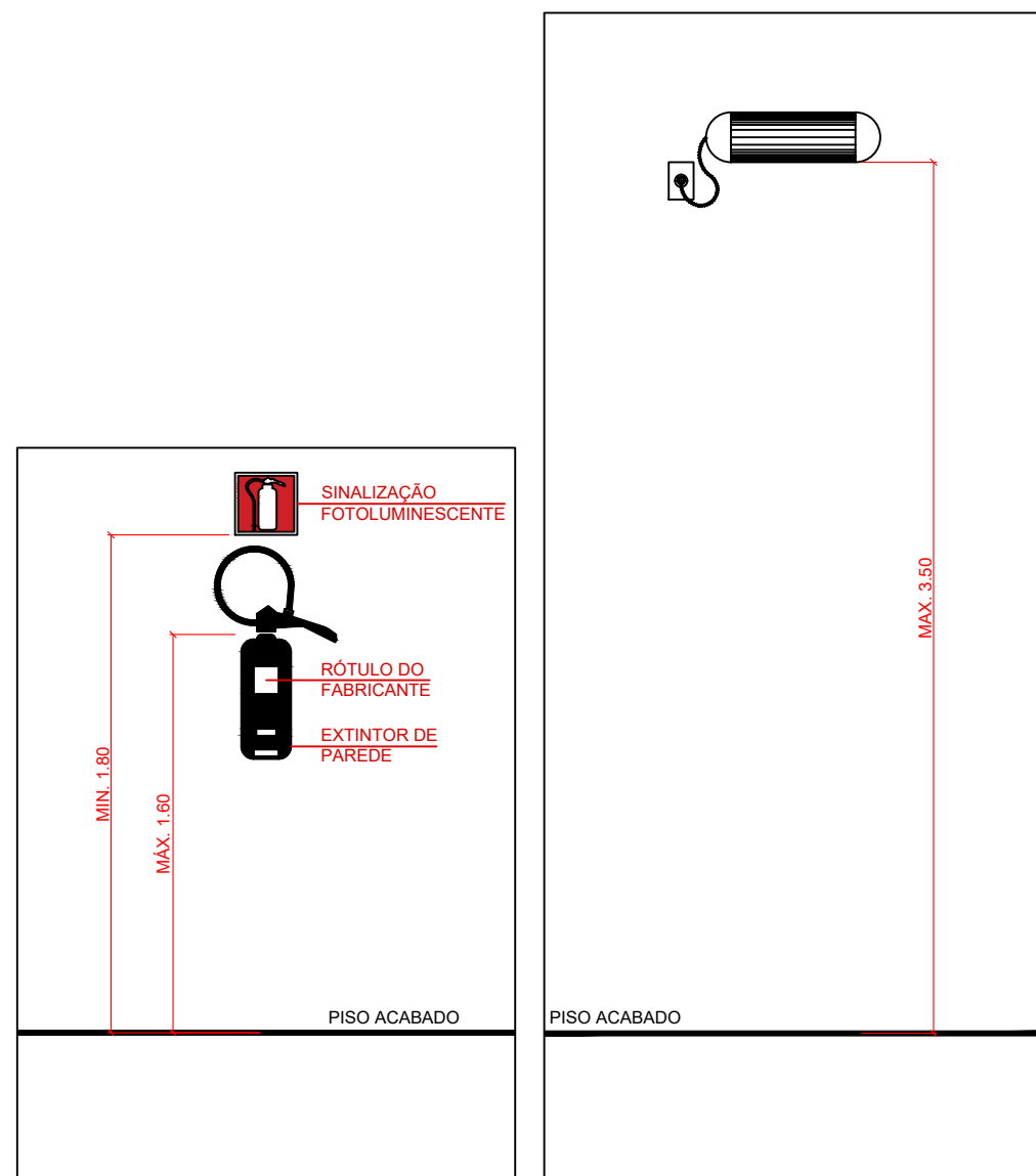
DET. EXTINTOR S/BSG. DET. ILUM. EMERGÊNCIA S/BSG.
