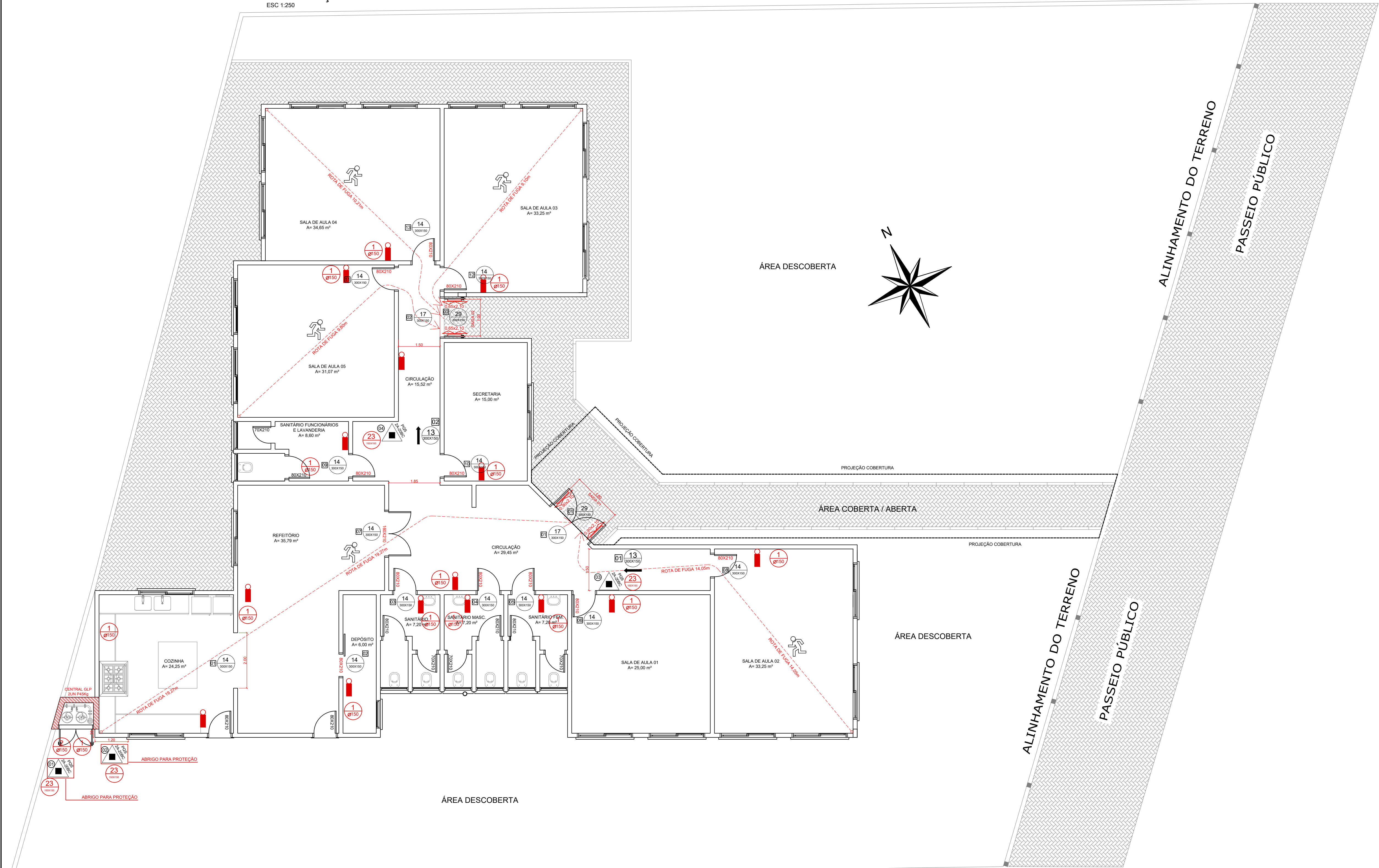
PLANTA BAIXA ESC 1:75
