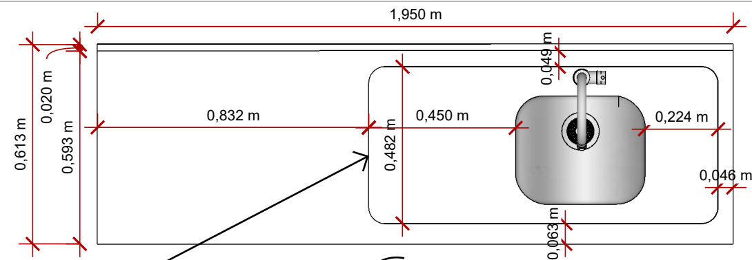
VISTA SUPERIOR PIA
