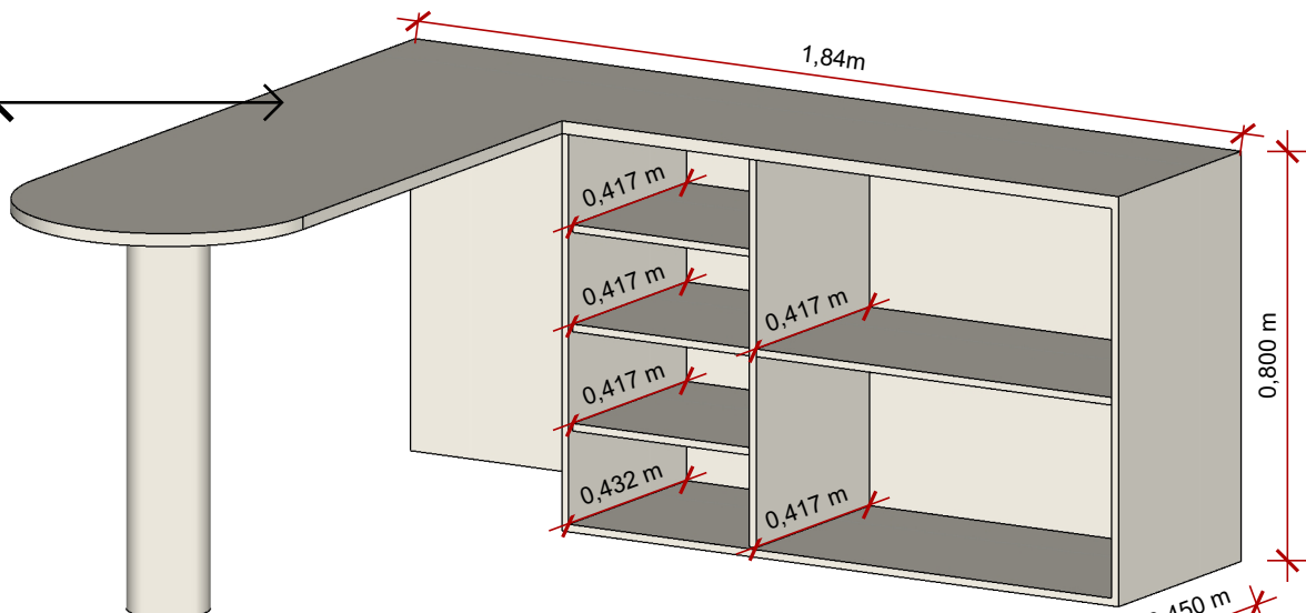
VISTA ISOMÉTRICA
