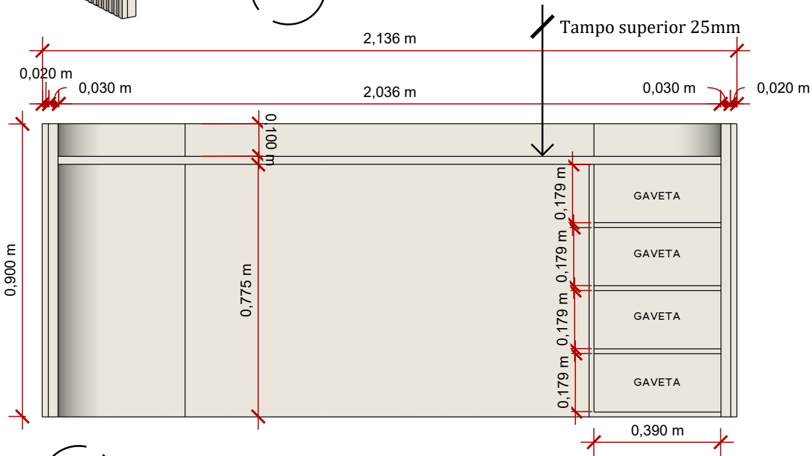
VISTA INTERNA
