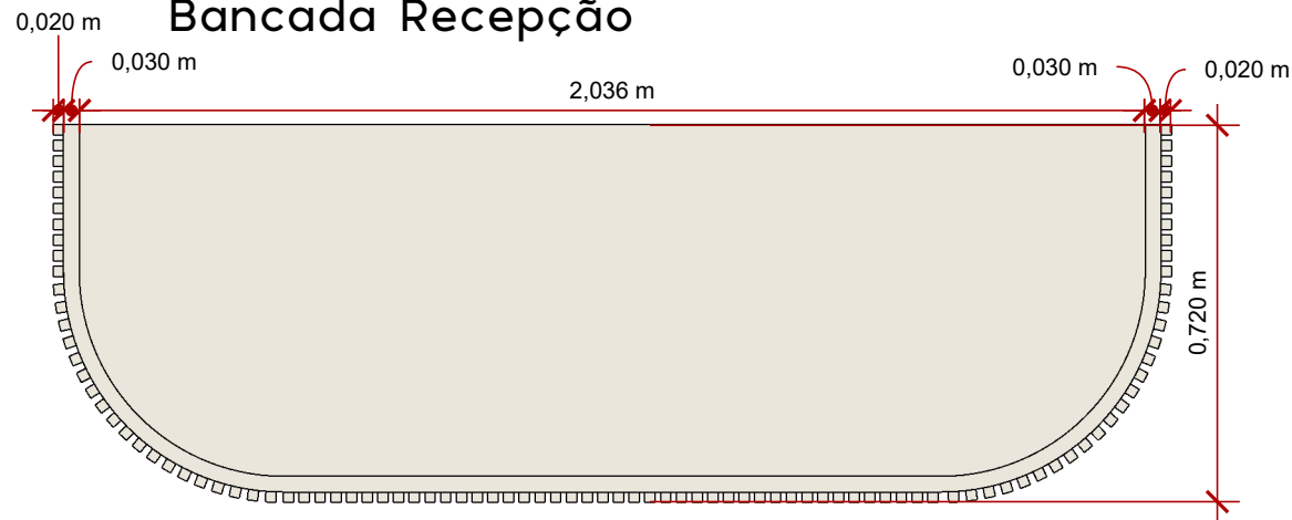
VISTA SUPERIOR
