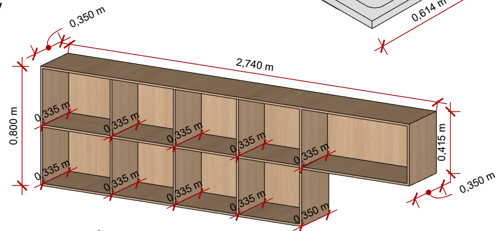
VISTA ISOMÉTRICA PIA
