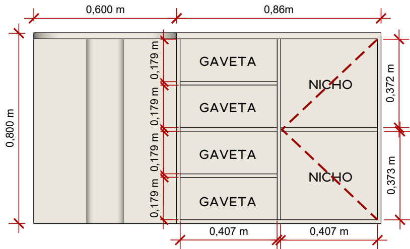
VISTA FRONTAL (MODELO 02 - SALA FISIOTERAPIA)
