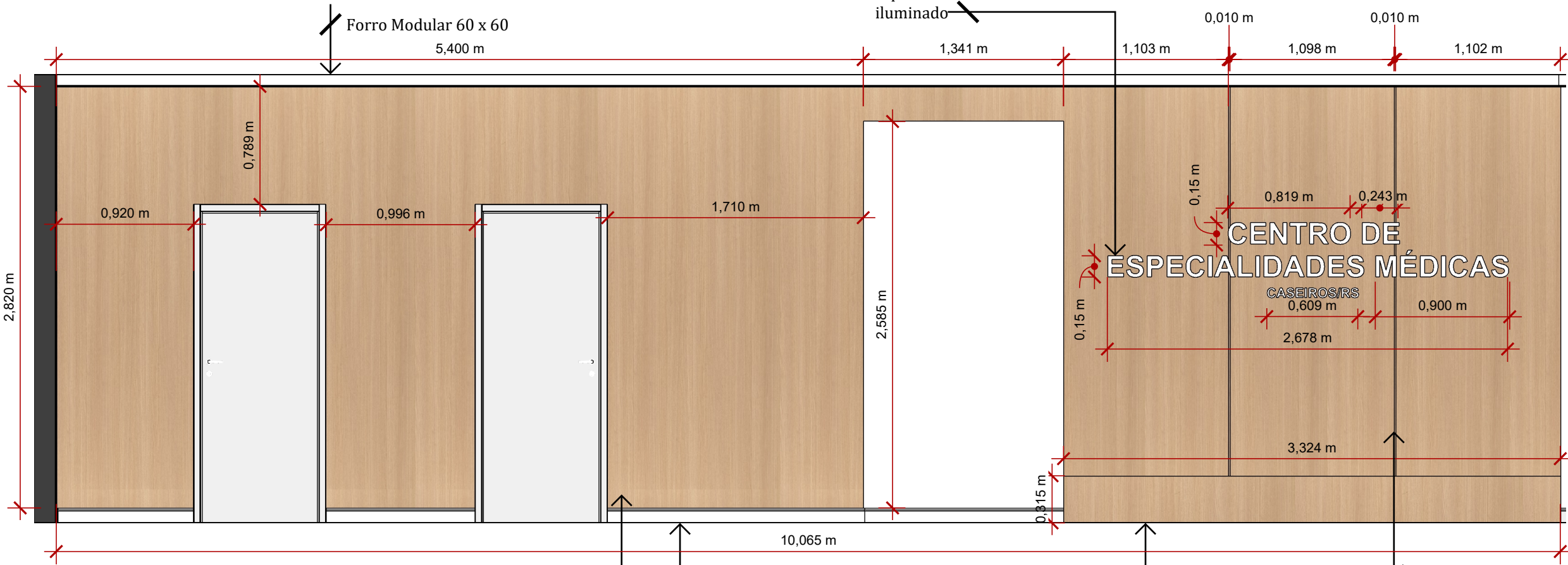
VISTA FRONTAL RECEPÇÃO
