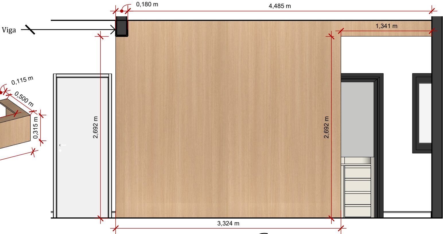
VISTA INTERNA CORREDOR BANHEIROS
