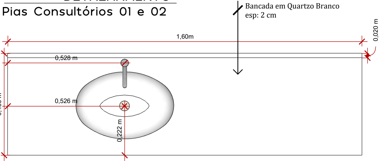
VISTA SUPERIOR
