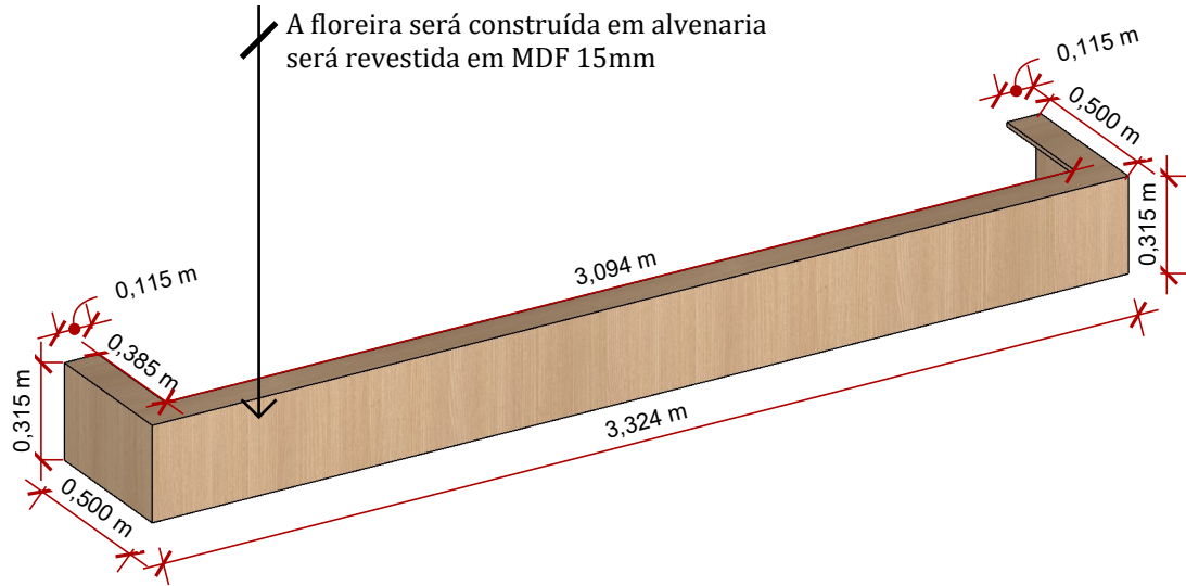
VISTA ISOMÉTRICA FLOREIRA
