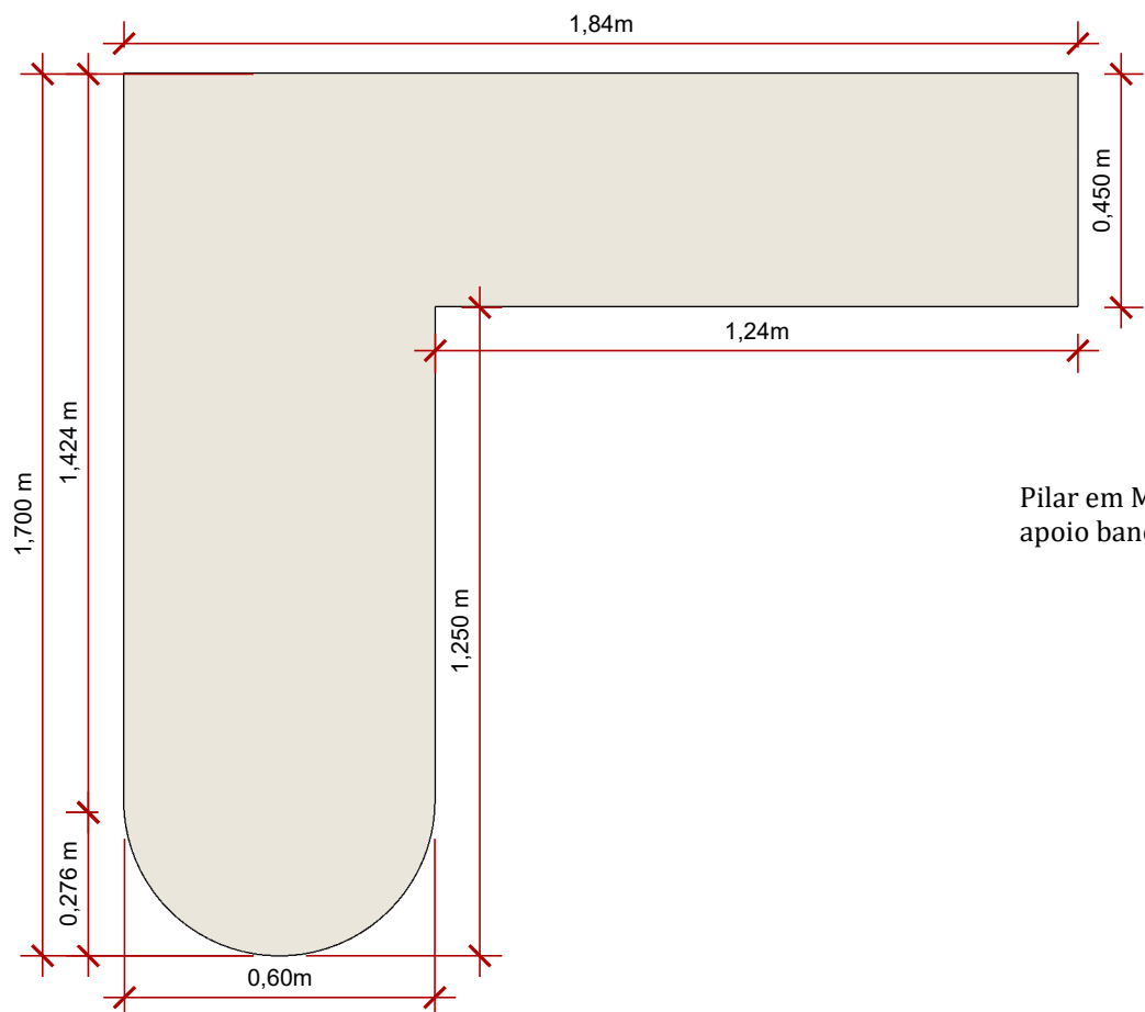
VISTA SUPERIOR
