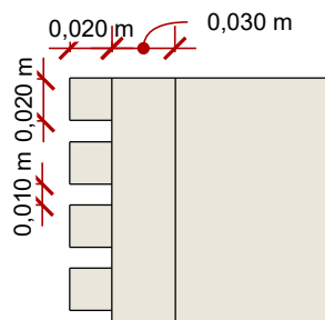
DET. RIPADO
