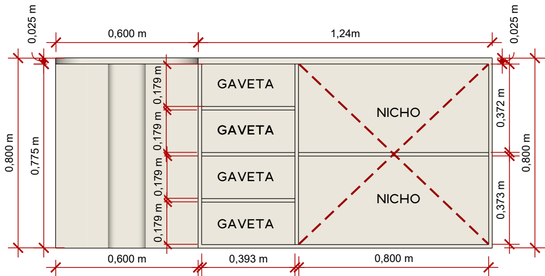
VISTA FRONTAL (MODELO 01)
