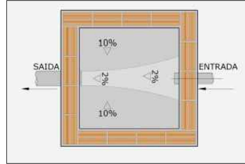
FILTRO ANAERÓBIO PLANTA BAIXA - ESC. 1:25
