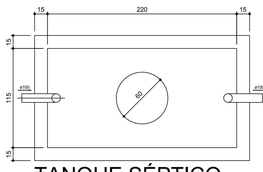
TANQUE SÉPTICO PLANTA BAIXA - ESC. 1:25
