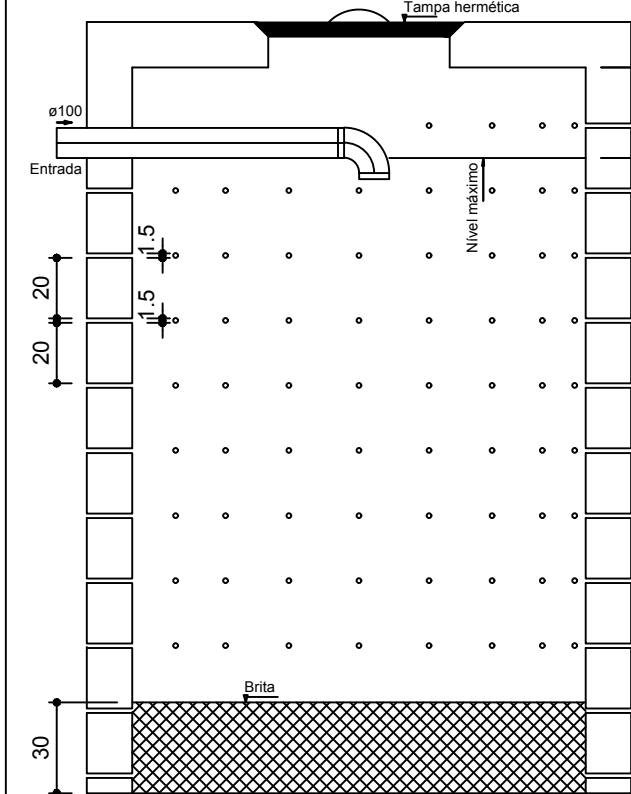
SUMIDOURO CORTE - ESC. 1:25
