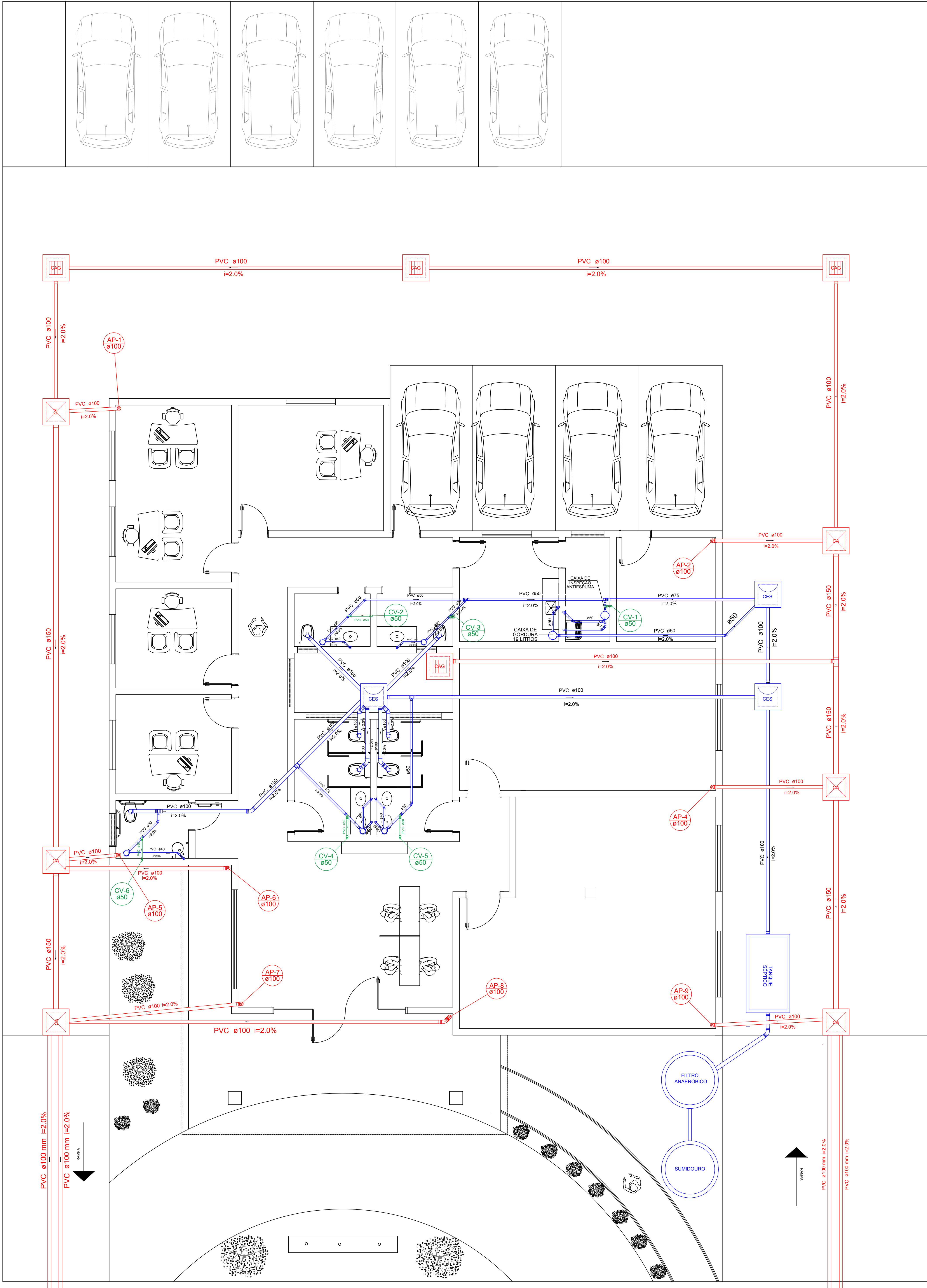
SUMIDOURO PLANTA BAIXA - ESC. 1:25
