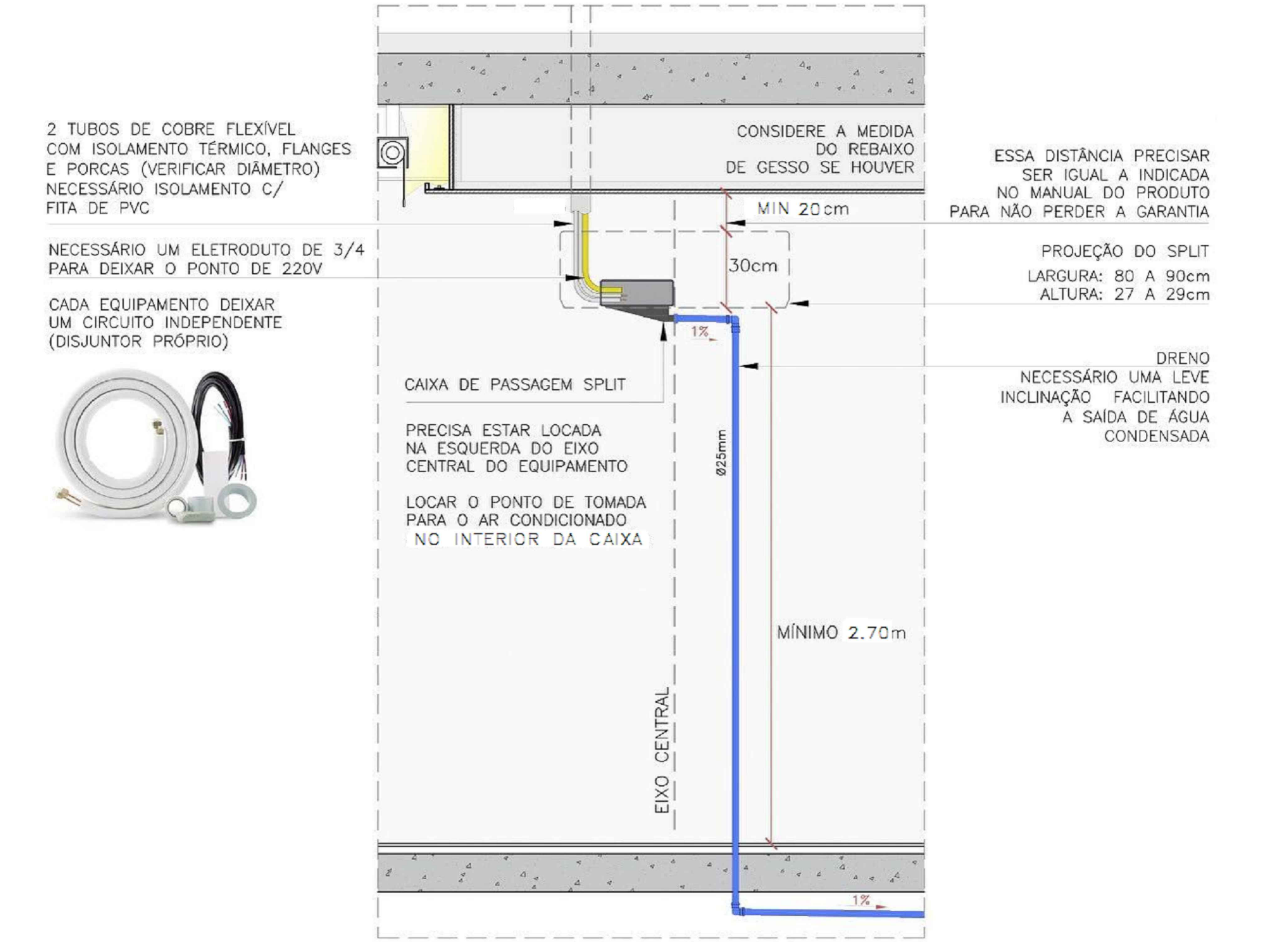
ESQUEMA ILUSTRATIVO DAS INSTALAÇÕES DAS ESPERAS OBS: Verificar os locais das unidades evaporadoras indicadas
