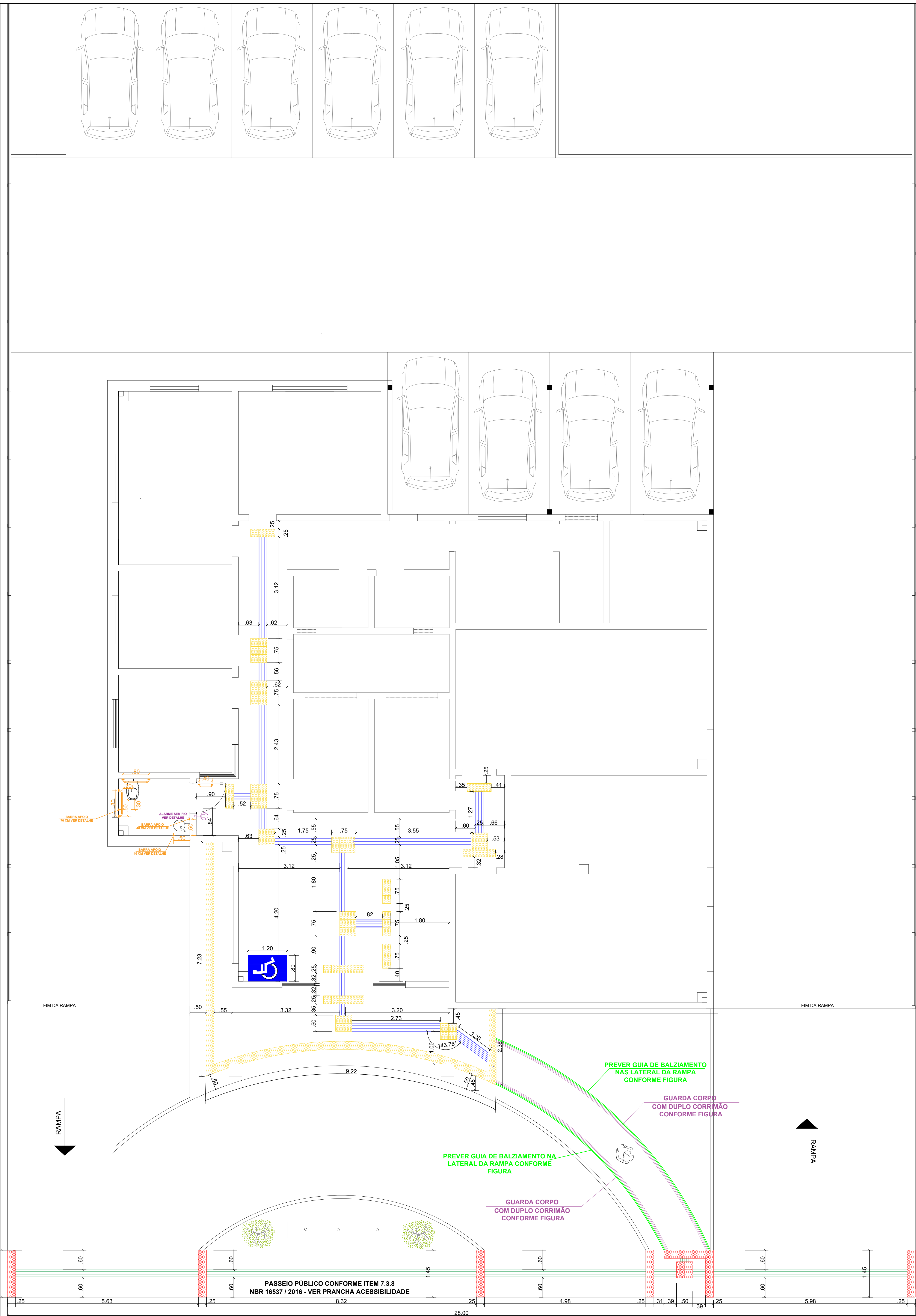
ACESSIBILIDADE / PASSEIO PÚBLICO
