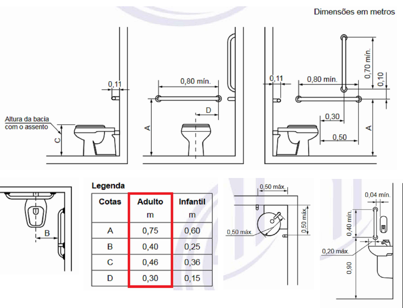
DETALHE INSTALAÇÕES BARRAS DE APOIO BANHEIRO PCD Conforme item 7.7.2.3.1 da NBR 9050/2024
