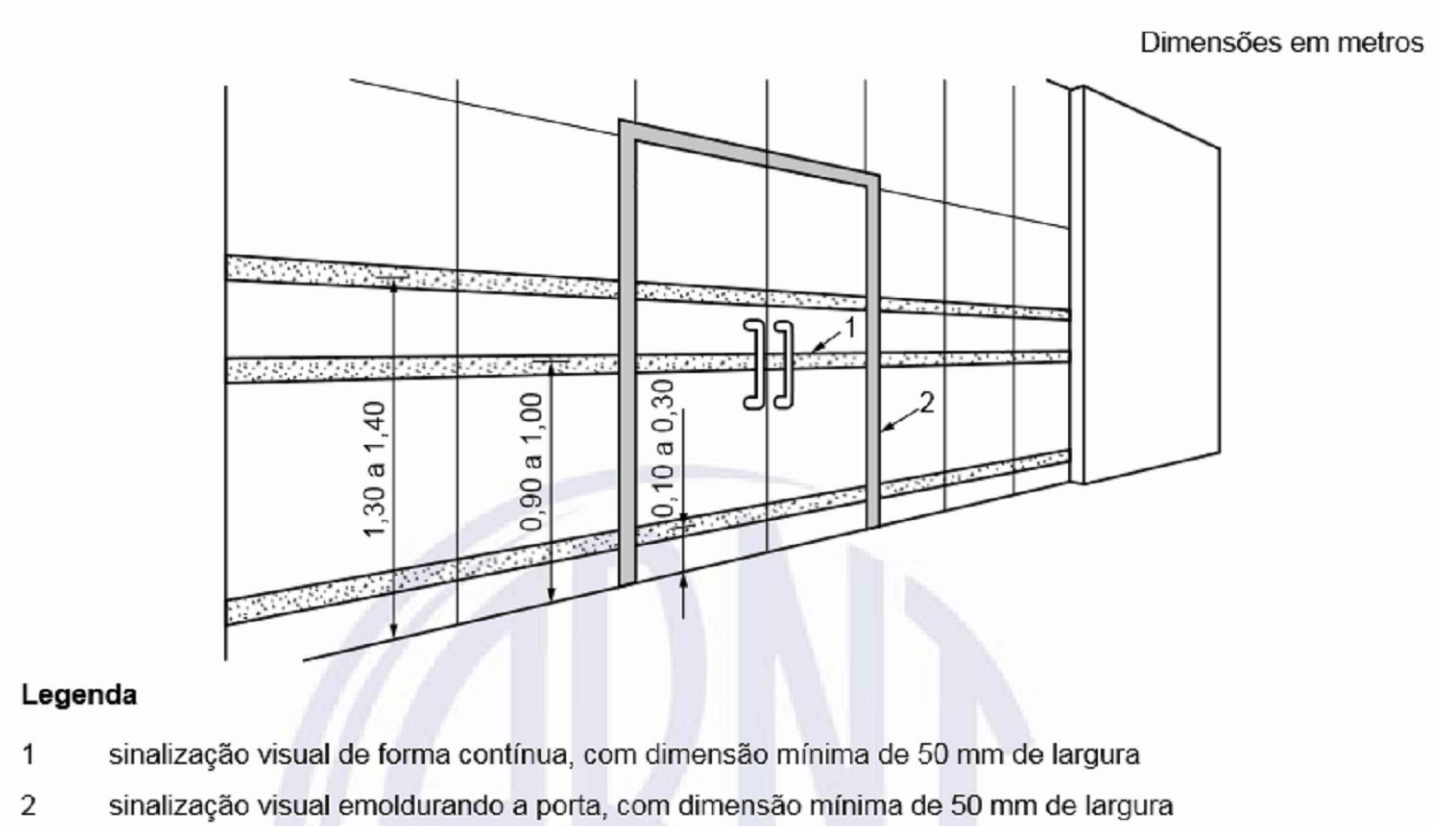
DETALHE SINALIZAÇÃO PORTA DE VIDRO PRINCIPAL ACESSO Conforme item 6.11.2.13 da NBR 9050/2024
