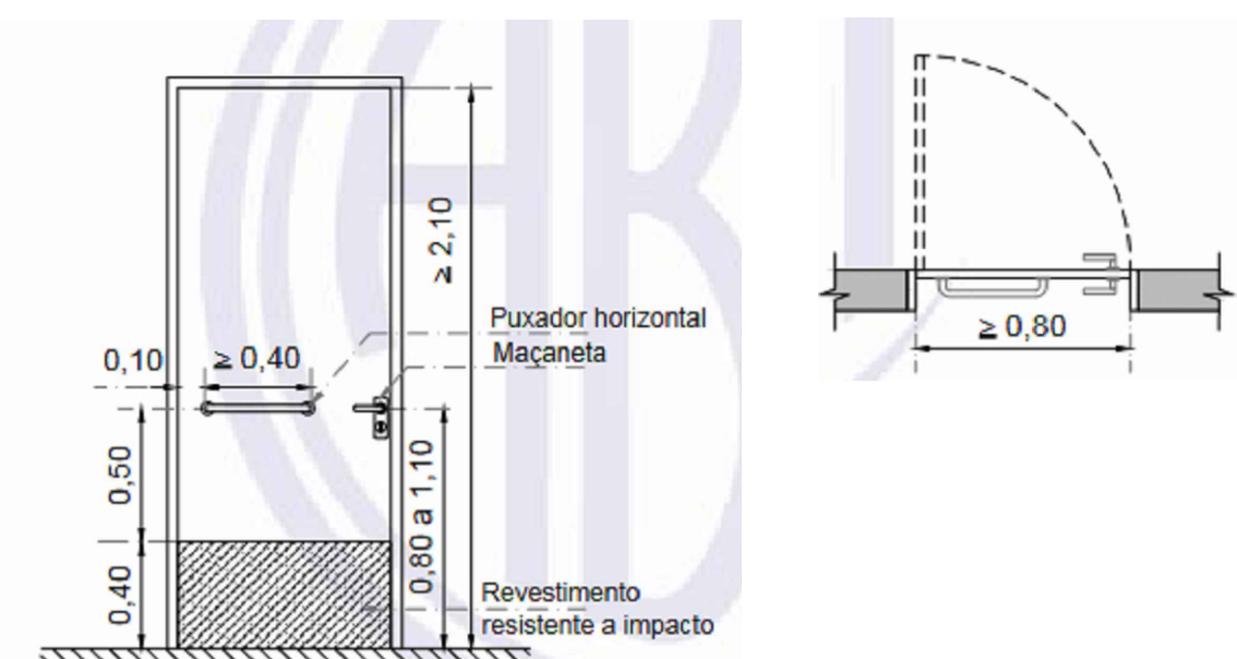
DETALHE ACESSÓRIOS PORTA BANHEIRO PCD Conforme item 6.11.2.7 da NBR 9050/2024
