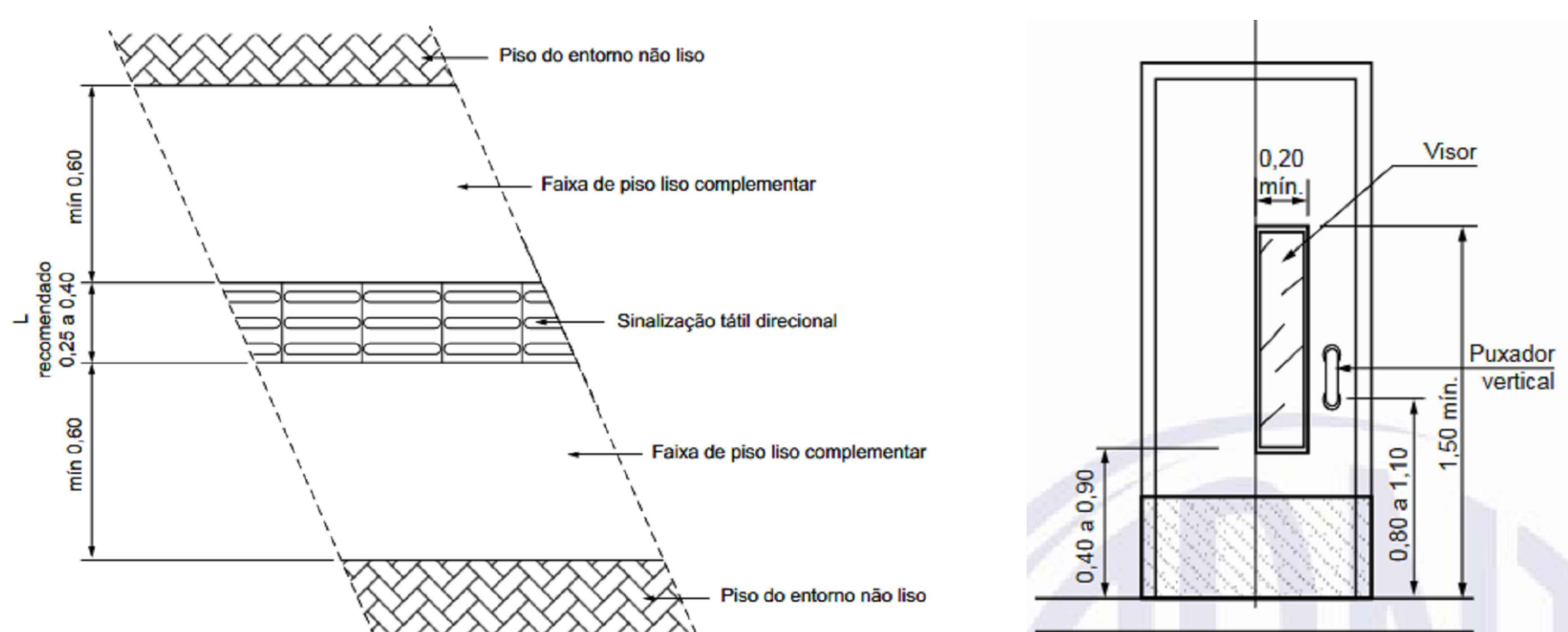
DETALHE PASSEIO PÚBLICO Conforme item 7.3.8 da NBR 16537/2016
