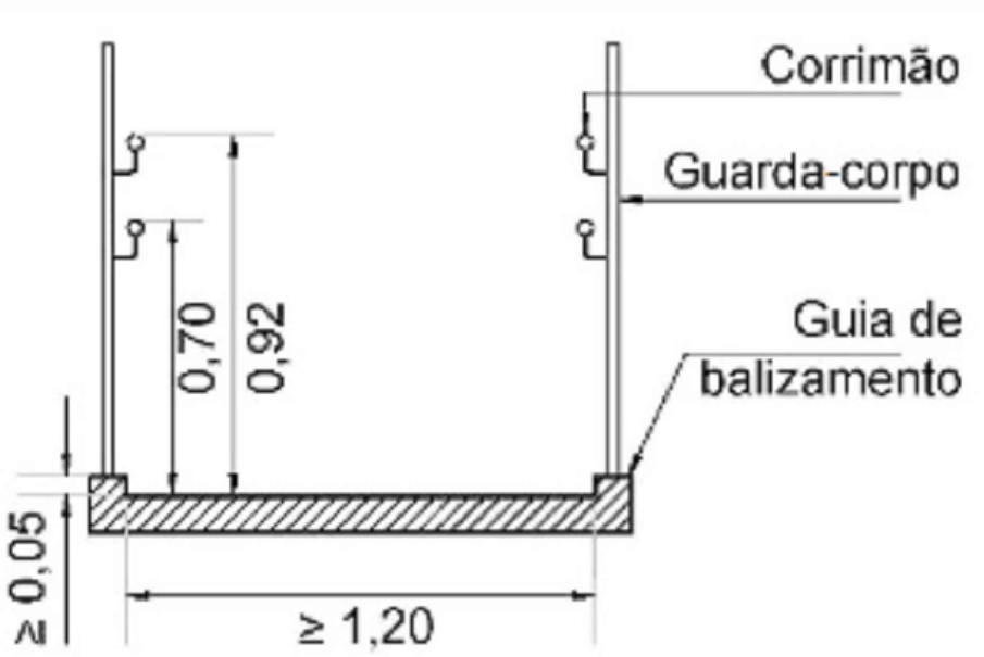
GUIA DE BALIZAMENTO CONCRETO RAMPA Conforme item 6.6.3 da NBR 9050/2024
