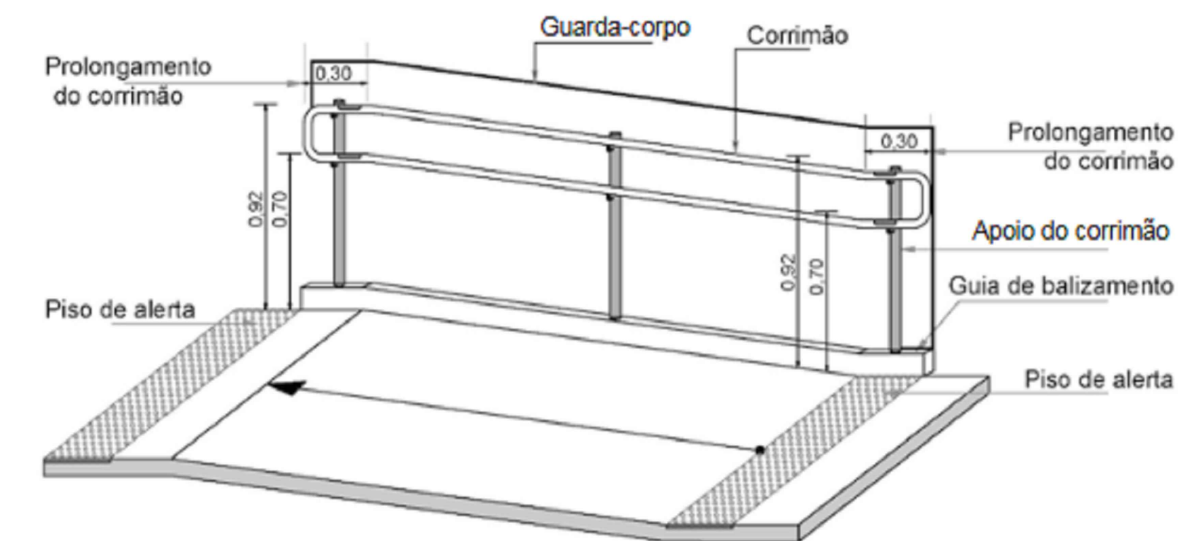
DETALHE DUPLO CORRIMÃO DA RAMPA DE ACESSO Conforme item 6.9.3.2 da NBR 9050/2024
