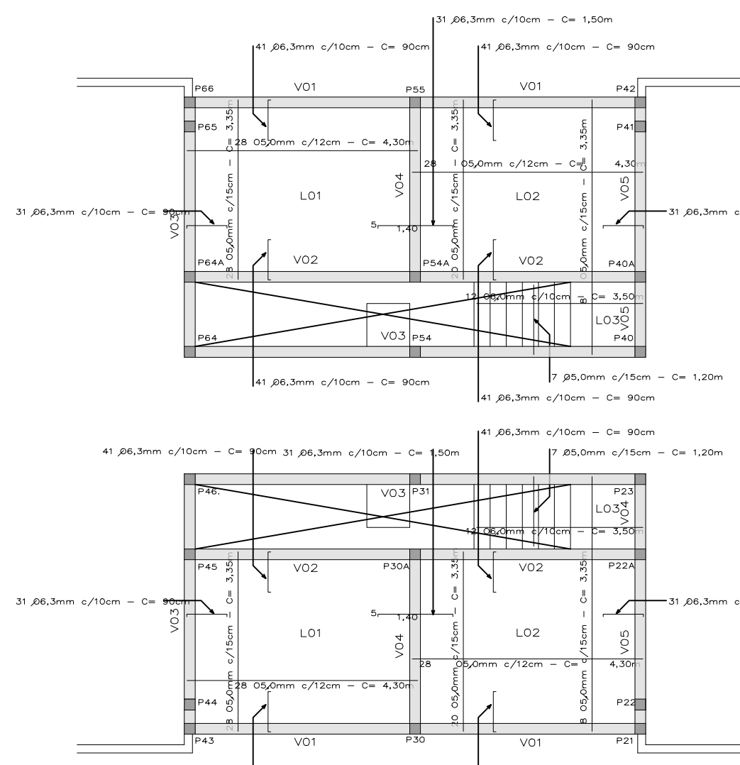
PLANTA BAIXA LAJES DOS RESERVATÓRIOS ESC. = 1:100
