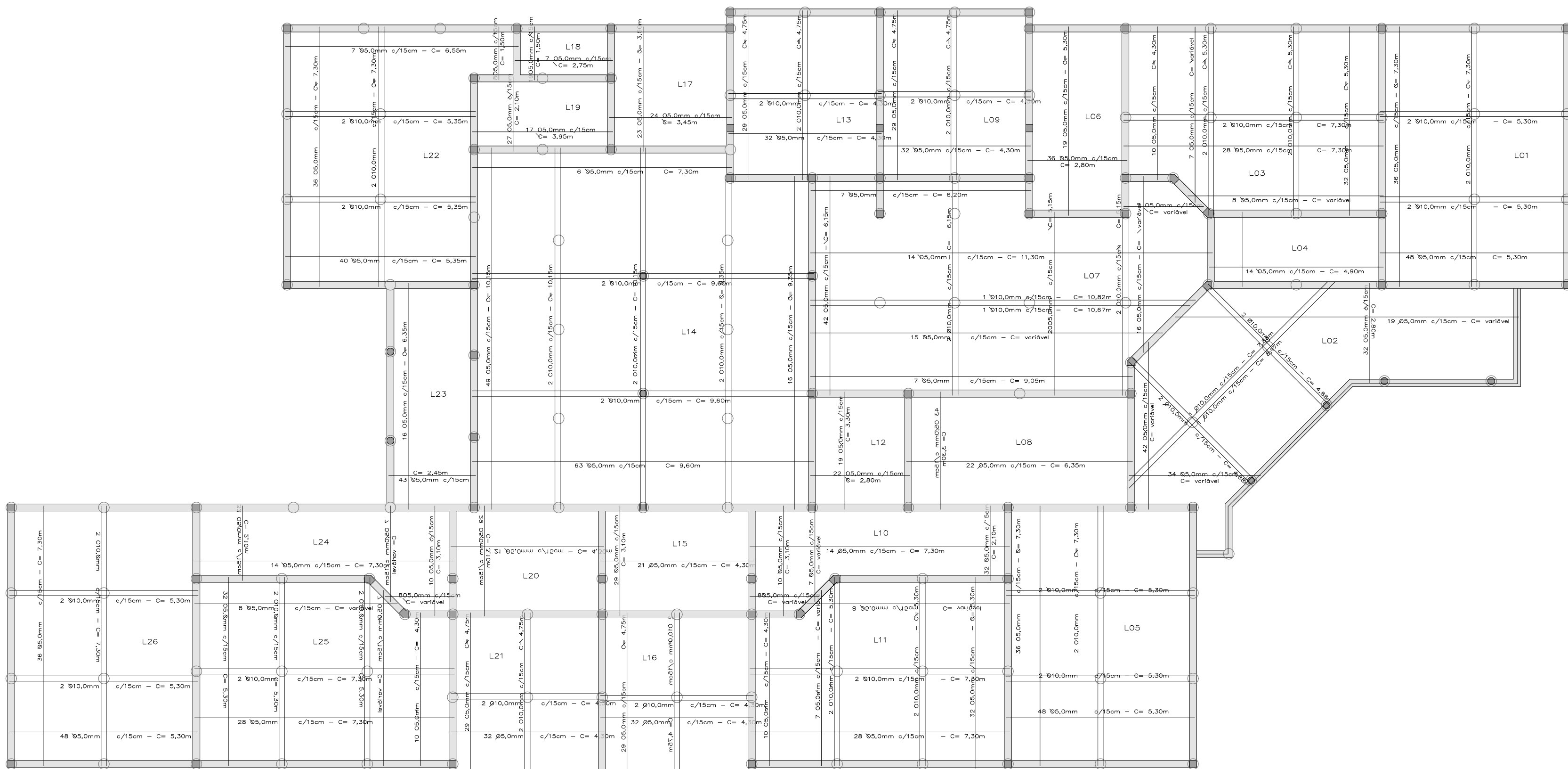
PLANTA BAIXA LAJES DE FUNDAÇÃO ESC. = 1:100
