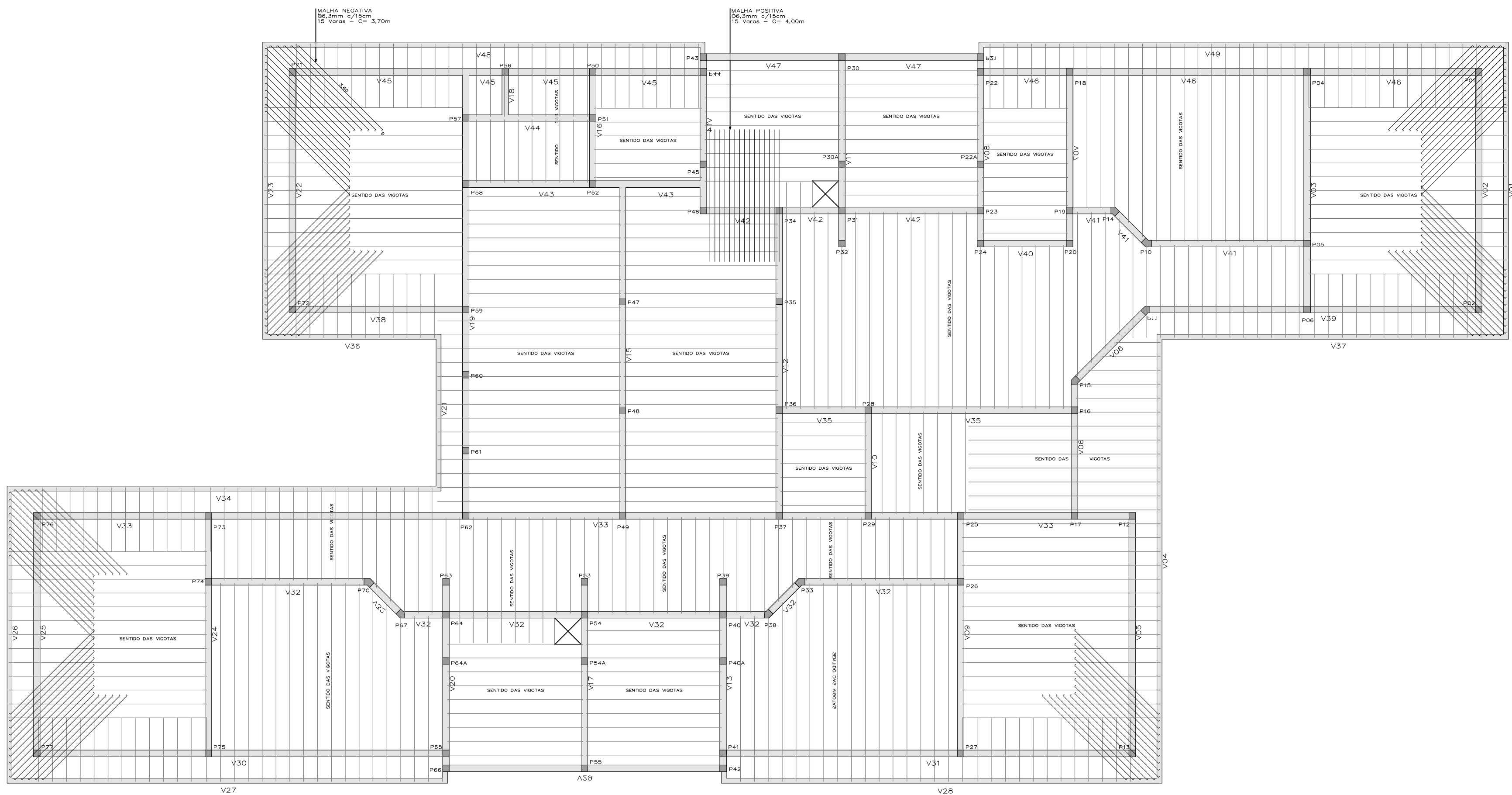
PLANTA BAIXA LAJES DE COBERTURA - PRE MOLDADAS ESC. = 1:100
