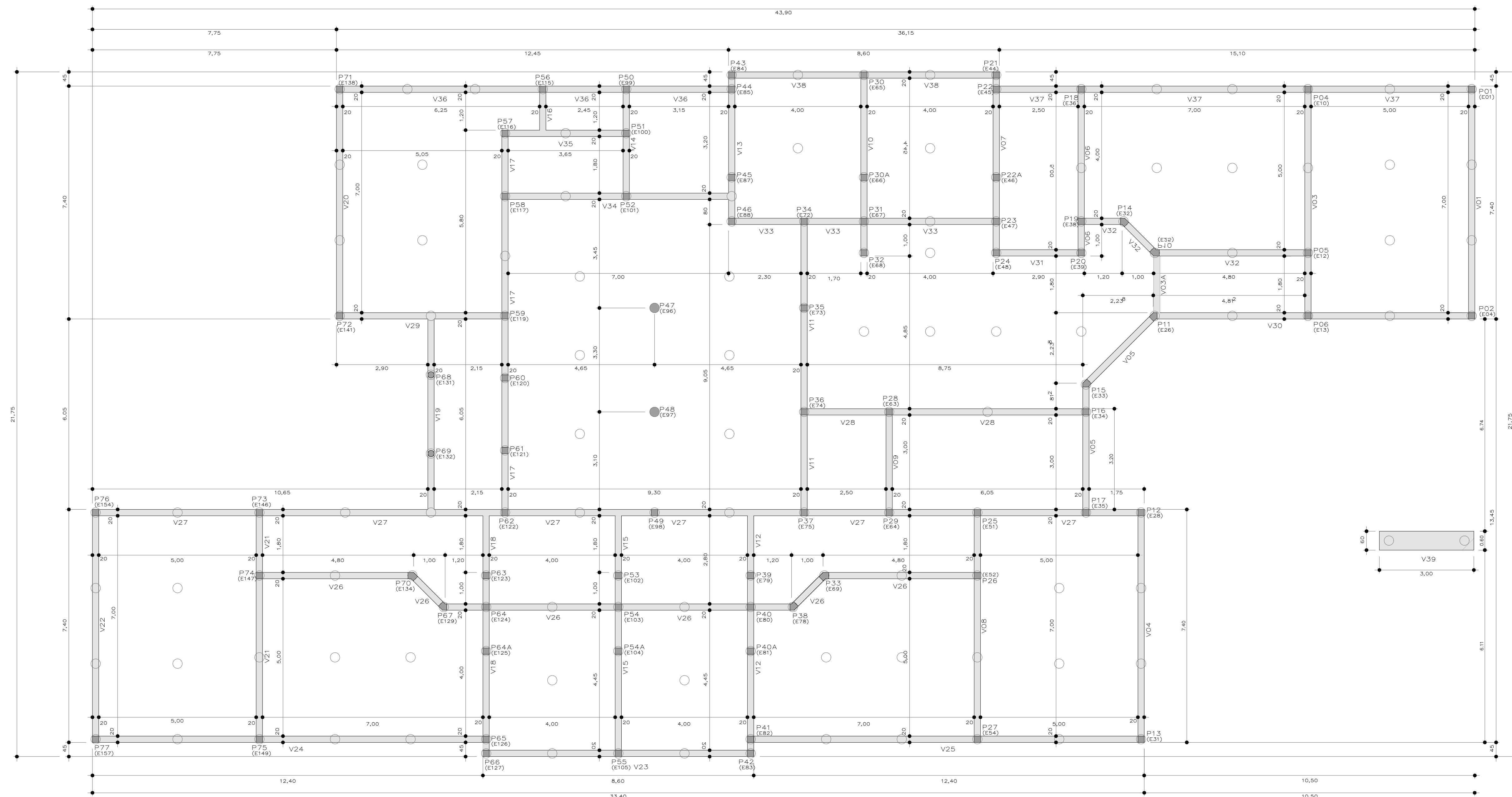
PLANTA BAIXA VIGAS DE BALDRAME E PILARES ESC. - 1:100
